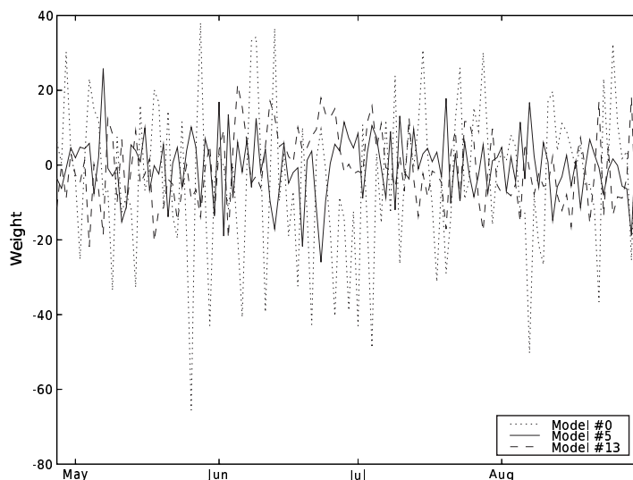
FIG. 5.4 – Évolution temporelle des trois poids les plus instables pour ELS d (ensemble 1, réseau 2), c'est-à-dire les poids ayant le plus grand écart-type. Les poids associés aux autres modèles sont aussi fortement variables.
