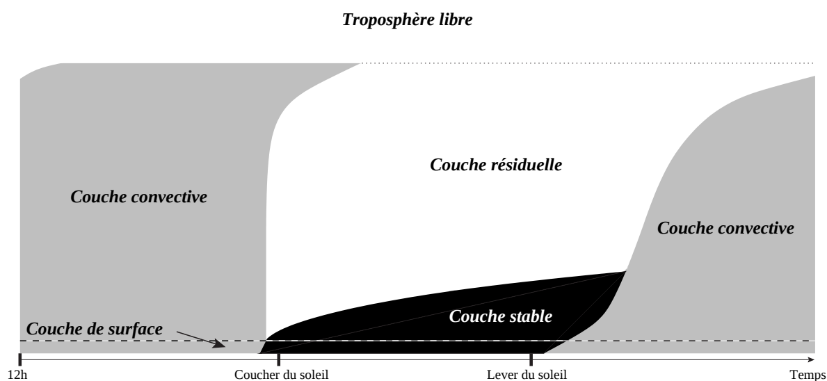
FIG. 1.3 – Évolution temporelle de la couche limite atmosphérique. Inspiré par Stull [1988].
