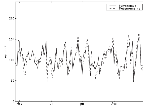
(d) Possen – RMSE : 15.5 \mu\text{g} \cdot \text{m}^{-3} , corrélation : 81.8%
