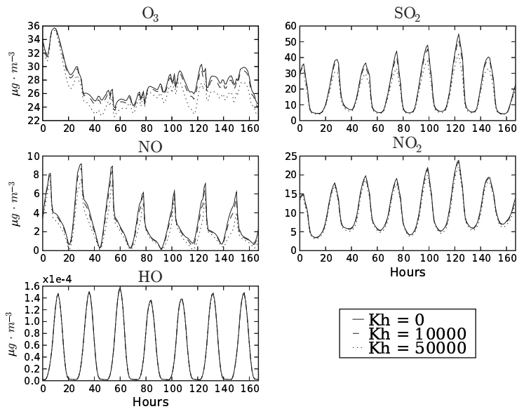
FIG. 3.12 – Évolutions temporelles des écarts-types spatiaux selon le coefficient de diffusion horizontale ( K_h = 0 \text{ m}^2 \cdot \text{s}^{-1} , K_h = 10000 \text{ m}^2 \cdot \text{s}^{-1} et K_h = 50000 \text{ m}^2 \cdot \text{s}^{-1} ).
