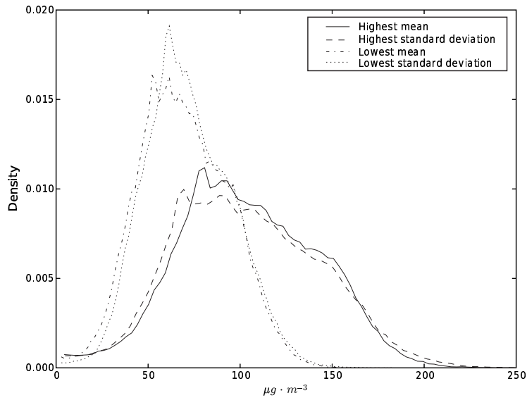
FIG. 3.32 – Distribution (spatio-temporelle) des concentrations d’ozone pour des simulations extrêmes, dont les caractéristiques sont d’avoir la moyenne la plus grande ( 103.4 \mu\text{g} \cdot \text{m}^{-3} ), l’écart-type le plus grand ( 40.3 \mu\text{g} \cdot \text{m}^{-3} ), la moyenne la plus petite ( 69.2 \mu\text{g} \cdot \text{m}^{-3} ) et l’écart-type le plus petit ( 23.6 \mu\text{g} \cdot \text{m}^{-3} ).
