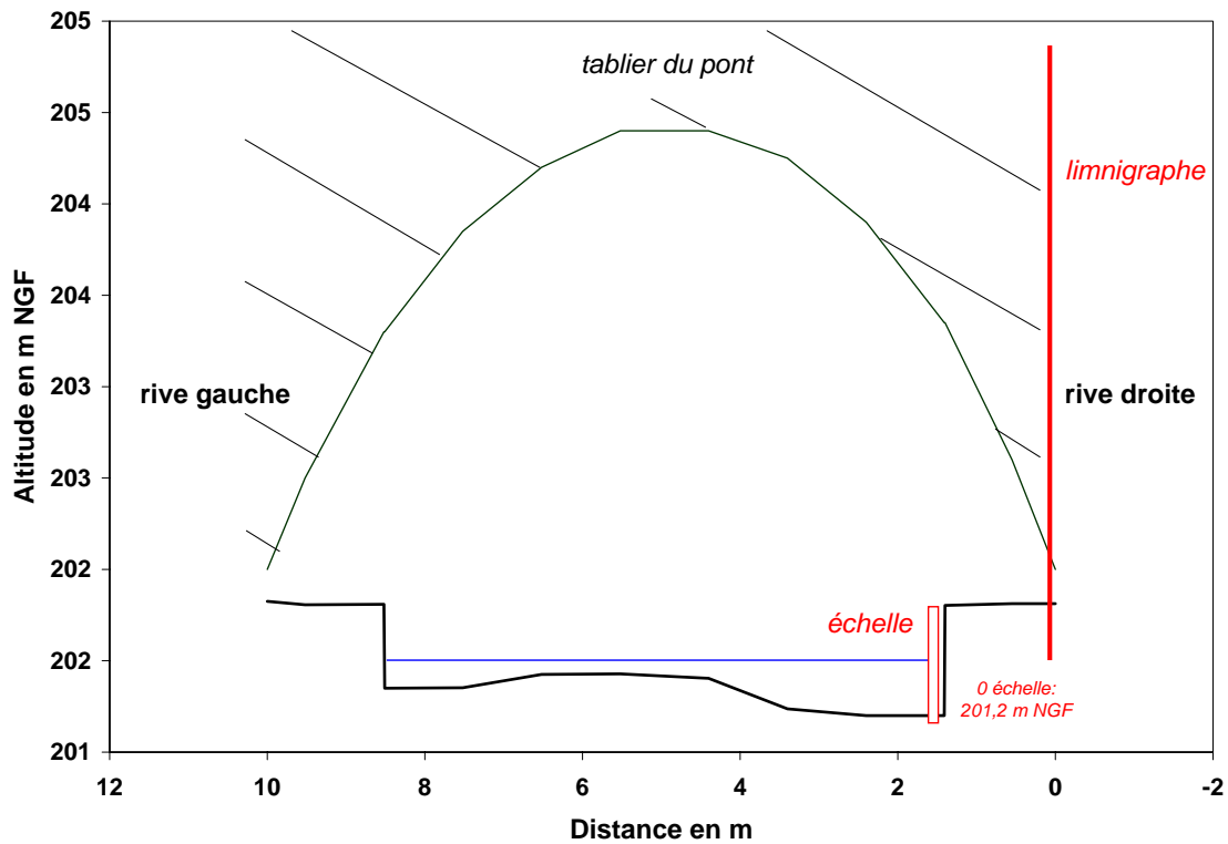
FIG. 3.3 – Station de mesure de Villeneuve Minervois sur la Clamoux - Schéma de la section
