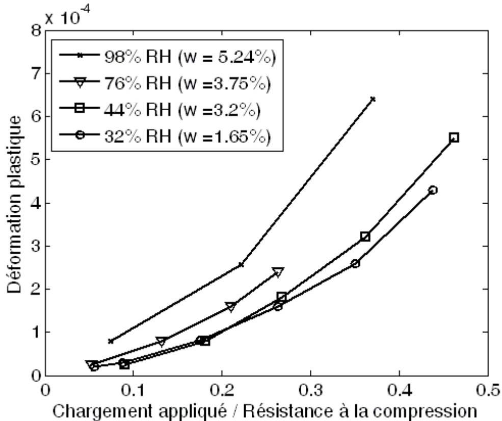
Figure 3-20 : Variation de la déformation plastique par rapport au chargement.
