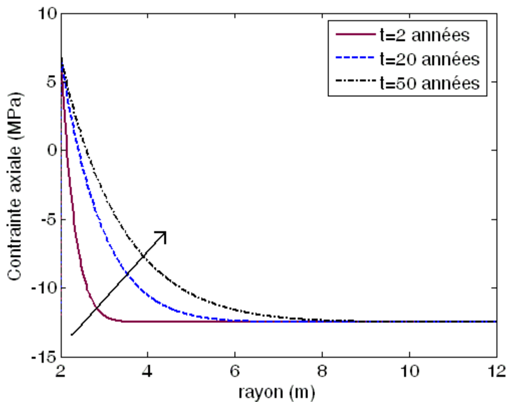
Figure 5-7 : Variation de la contrainte axiale (98%RH-80%RH).
