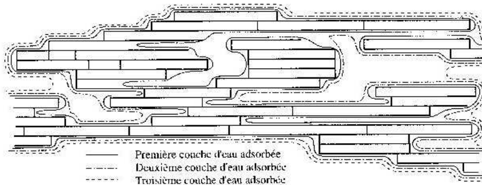
Figure 1-8 : L'eau adsorbée dans un paquet de feuillets smectitiques (Van Damme 2001).
