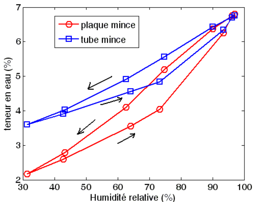
Figure 2-6a : Courbe de rétention.
