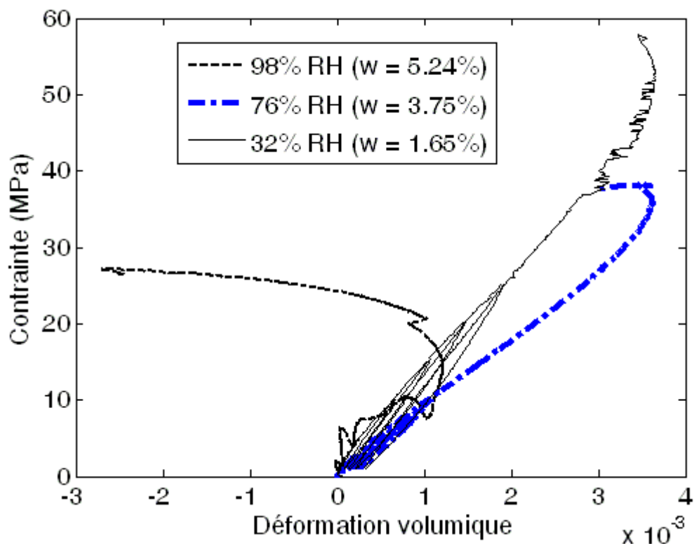
Figure 3-19 : Déformation volumique.
