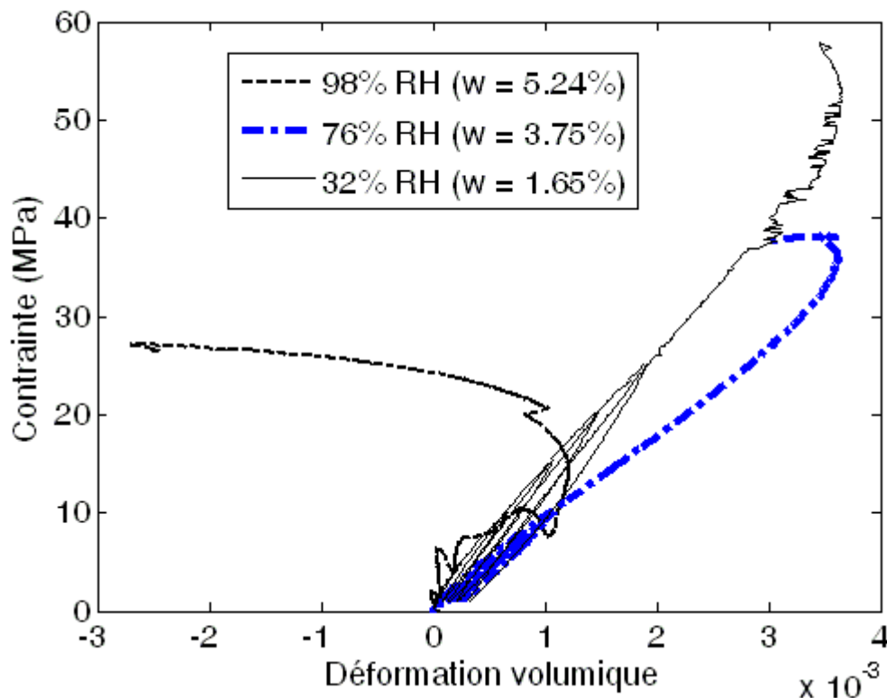
Figure 3-19 : Déformation volumique.
