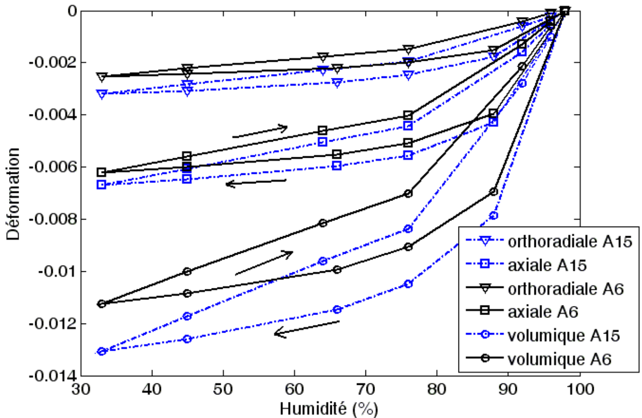
Figure 3-4 : Variation des déformations hydriques par rapport à l'humidité.
