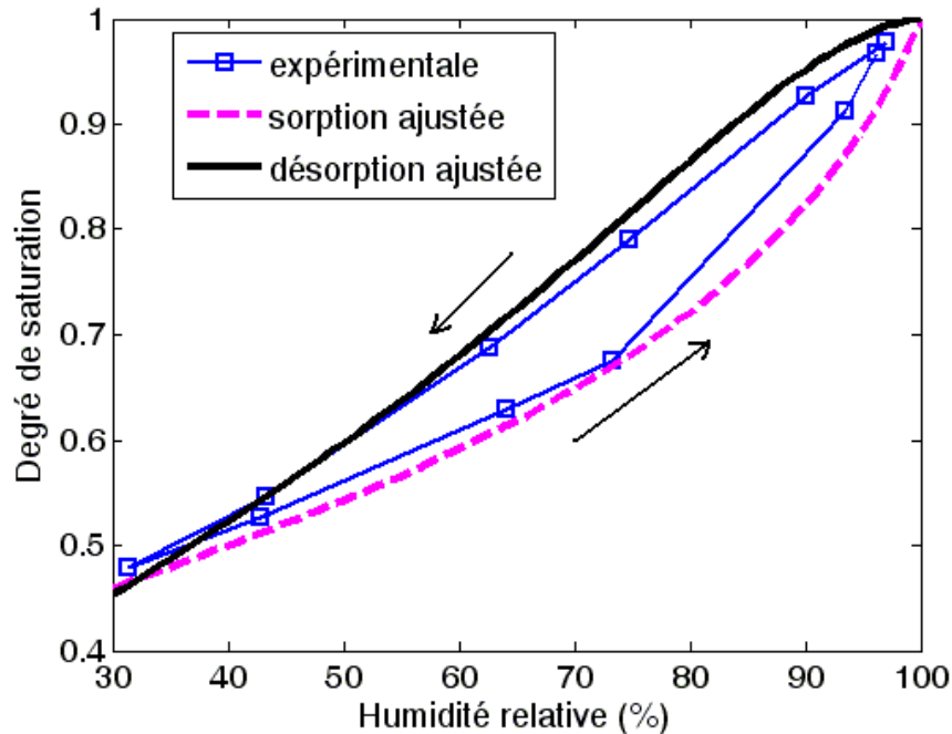
Figure 2-6b : Isotherme de sorption-désorption.
