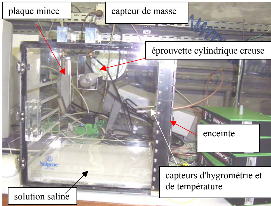
Figure f-2 : Instrumentation pour essais de transfert hydrique.
