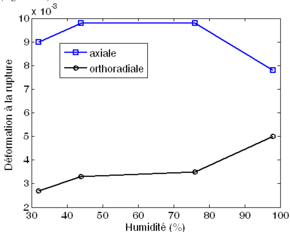
Figure 3-23 : Déformations à la rupture.
