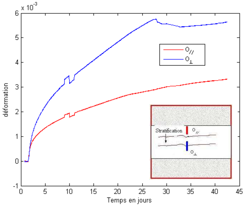
Figure 4-22 : Variation des déformations orthoradiales centres GT2 par rapport au temps.
