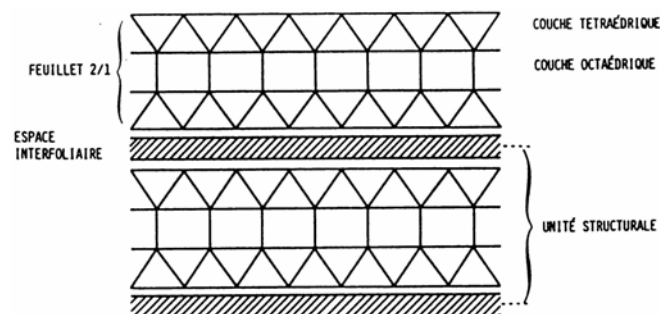
Figure 1-1 : Représentation schématique d'une structure de couche argileuse.
