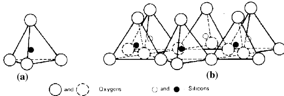
Figure 1-2 : a) Unité tétraédrique à cœur de silicium; b) Schéma d'une couche de tétraèdre [\text{Si}_4 \text{O}_{10} (\text{OH})_2]_{6-} avec arrangement hexagonal (Mitchell 1993).
