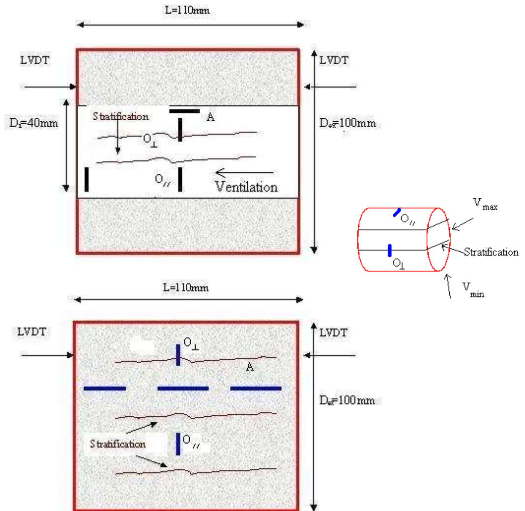
Figure 4-1b : Implantation des mesures de déformation des tubes GT1 et GT2 à leur trou et sur leur surface extérieure (en noir, jauges orthoradiales ( O_{//} et O_{\perp} ) et axiales A à l'intérieur du trou ; en bleu, jauges orthoradiales ( O_{//} et O_{\perp} ) et axiales A à la surface extérieure ; en rouge, gaine de protection).
