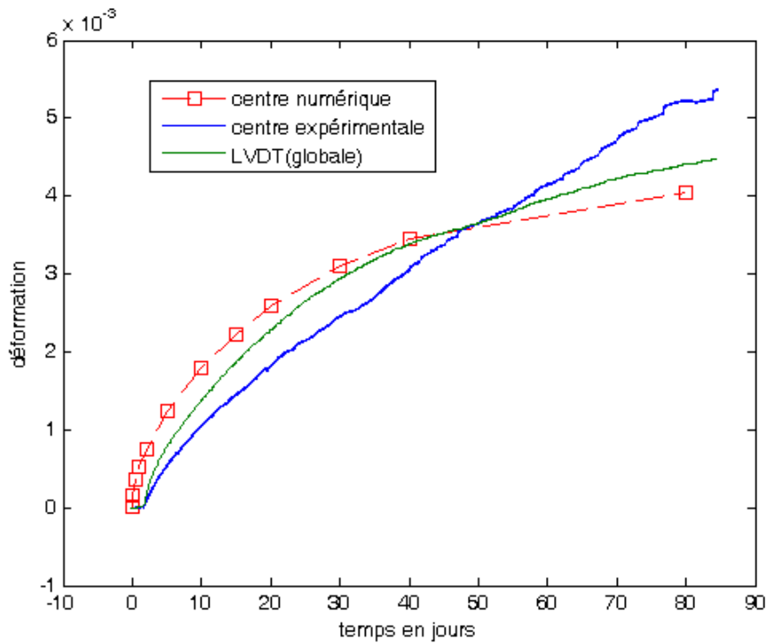
Figure 4-39 : Variation de la déformation axiale par rapport au temps (92 %RH- 97 %RH).
