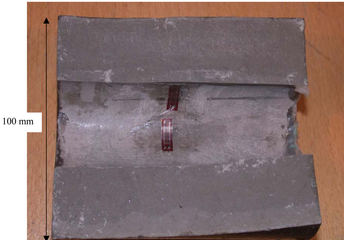
Figure 4-21d : Coupe transversale du tube GT1 (plan de rupture).
