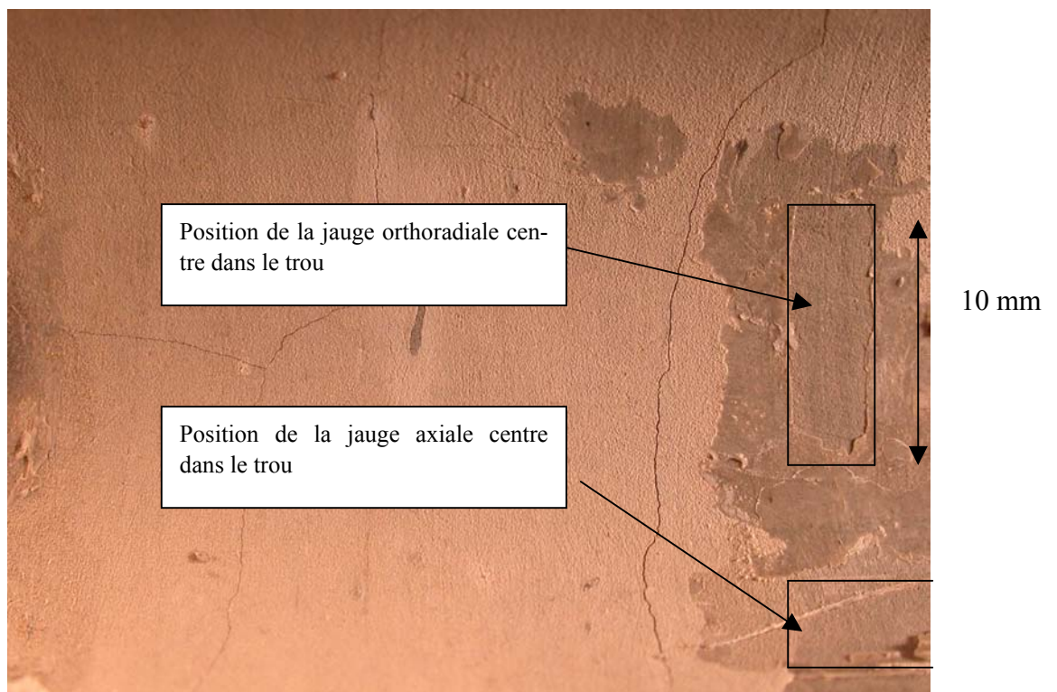
Figure 4-16b : Fissures dans le trou de tube épais et les position des jauges intérieures.
