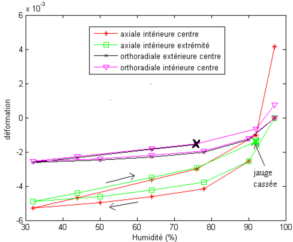
Figure 4-10 : Variation des déformations par rapport à l'humidité.
