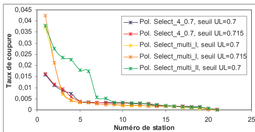
Figure 6.27 : Taux de coupure moyen par station (rangé dans l'ordre décroissant) pour les politiques Select_4_0.7 , Select_multi_I et Select_multi_II sur la zone de la ville 1.
