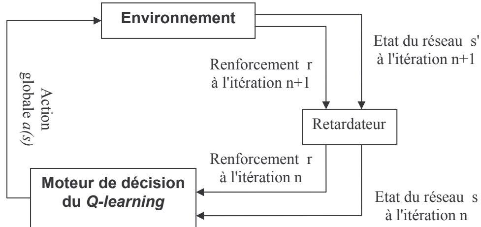
Figure 4.9 : Fonctionnement général de l'algorithme de Q-learning
