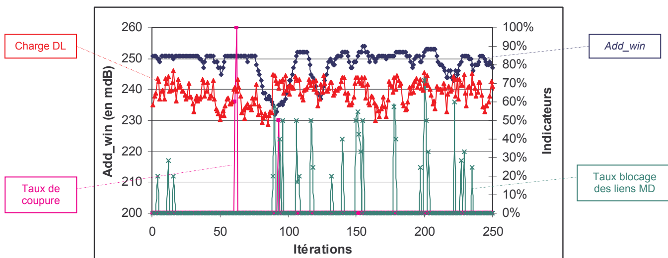
Figure 5.5 : Variations des indicateurs de charge DL (rouge), taux de coupure instantané (rose), taux de blocage des liens de MD instantané (vert) et du paramètre Add_win (bleu) sur une cellule chargée.
