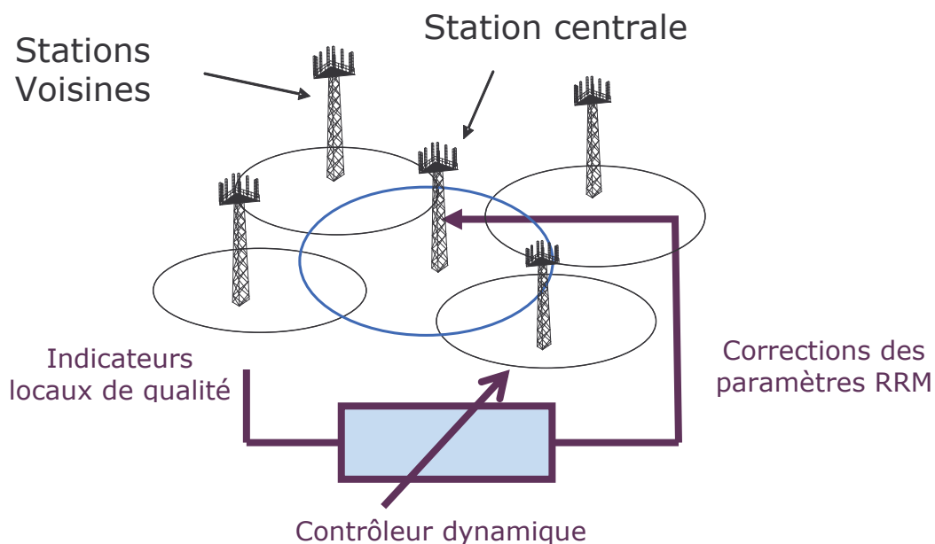
Figure 1.2 : Contrôleur dynamique de logique floue des paramètres RRM de la station centrale**.
