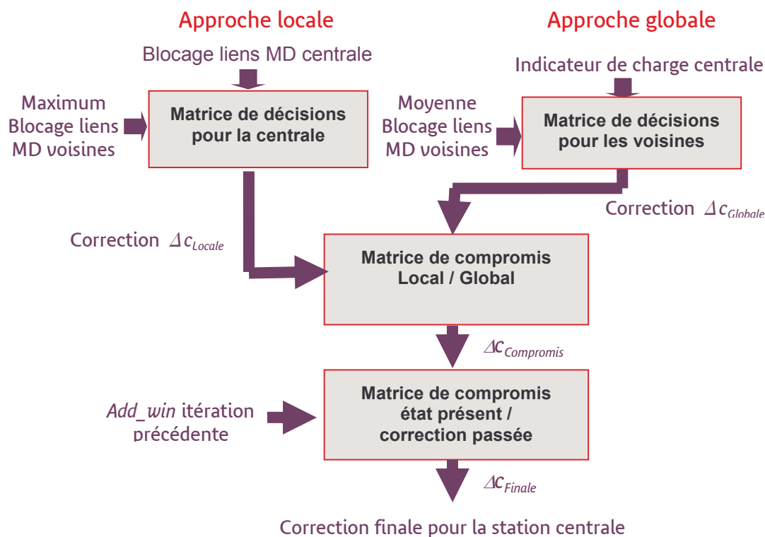
Figure 3.21 : Schéma de fonctionnement du contrôleur de logique floue pour le paramétrage de la macro-diversité
