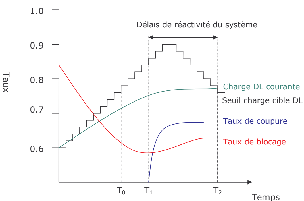
Figure 3.13 : Sans prise en compte de la différence entre la charge et le seuil de charge cible courants
