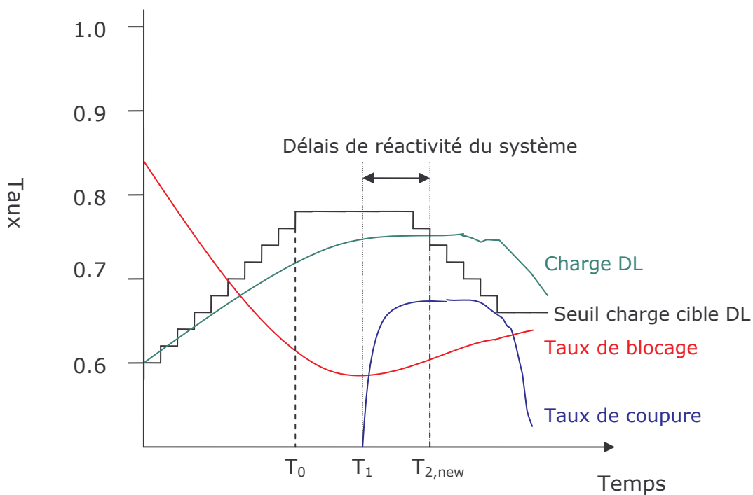
Figure 3.14 : Avec prise en compte de la différence entre la charge et le seuil de charge cible courants En revanche sur la figure 3.14, pour déterminer la correction à l'itération courante \Delta c^n le contrôleur prend en compte la différence entre la charge de la cellule et le seuil de charge
