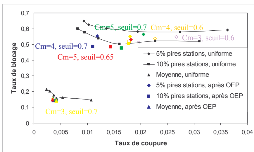
Figure 6.17 : Efficacité des politiques optimisées pour différents couples (paramétrage initial / coefficient de mixage) par rapport aux fronts P.U. dans le plan taux de coupure / taux de blocage.
