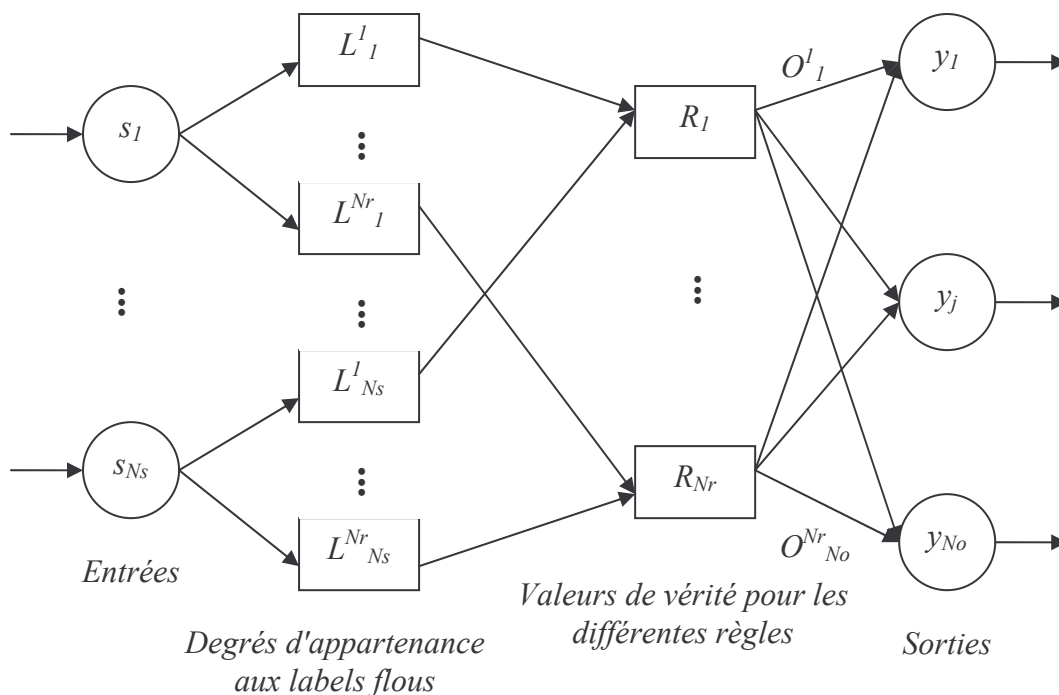
Figure 3.1 : Diagramme d'un système d'inférence floue.
