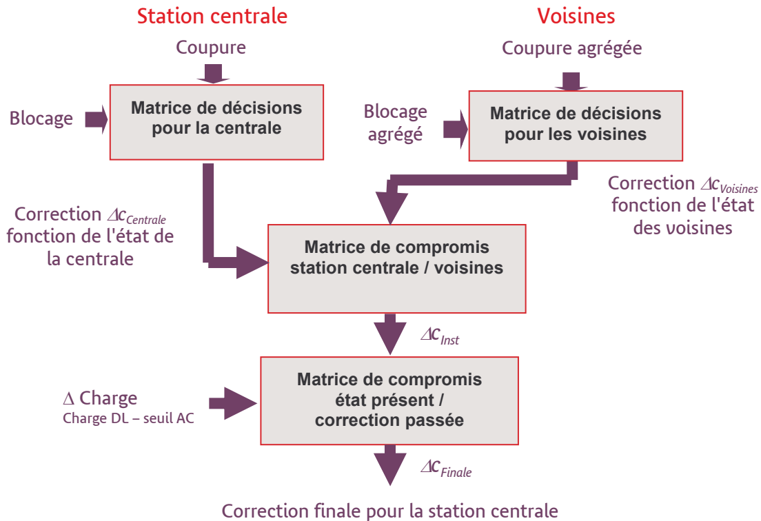
Figure 3.20 : Schéma de fonctionnement du contrôleur de logique floue pour le paramétrage du contrôle d'admission
