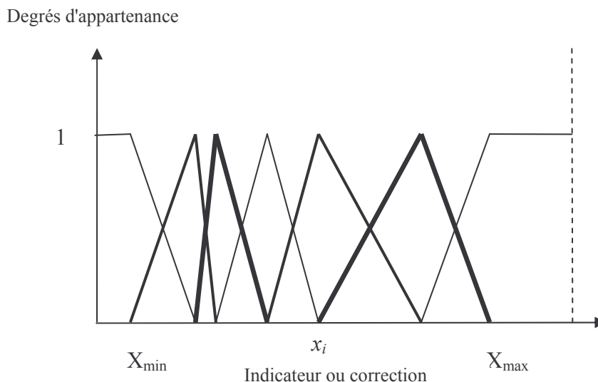
Figure 3.12 : Famille irrégulière de sept valeurs floues. Les valeurs de rang 1, 3, 5, 7 sont définies par 7 paramètres. Les autres s'en déduisent.
