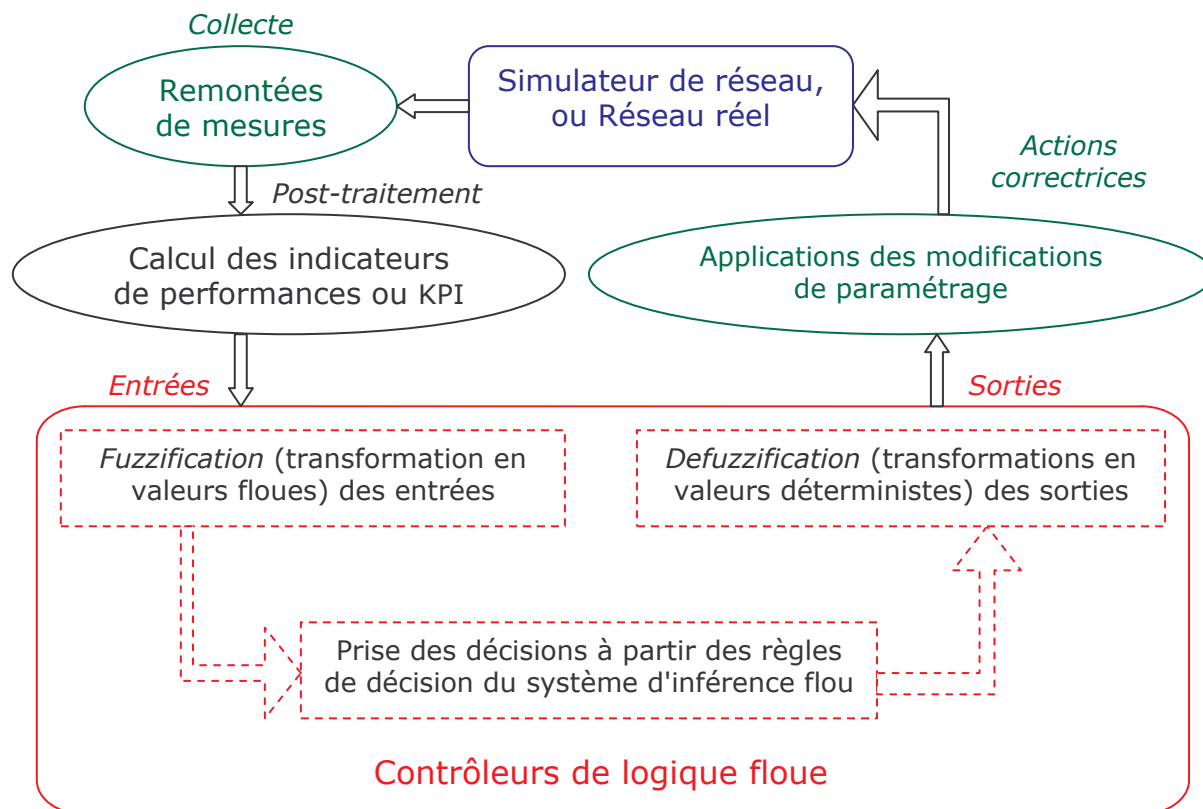
Figure 3.4: Schéma de fonctionnement du contrôle automatique par logique floue.
