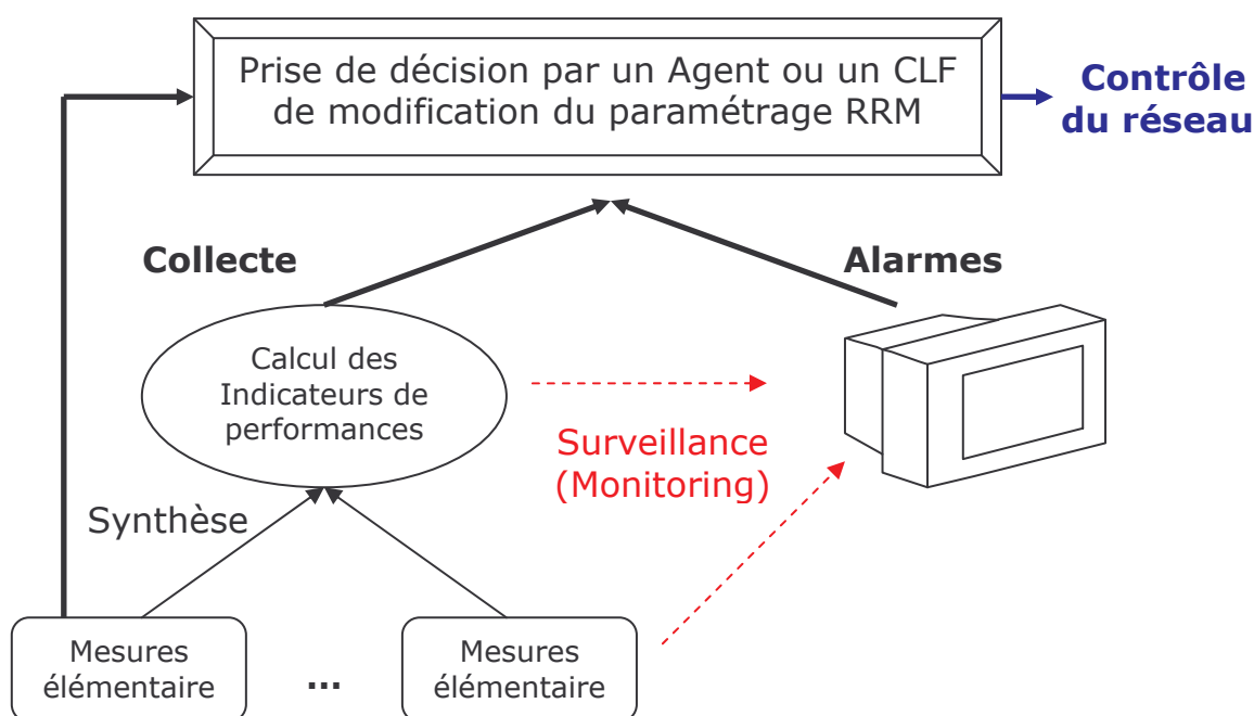
Figure 3.6 : Schéma de remontées de mesures et surveillance dans un réseau mobile.
