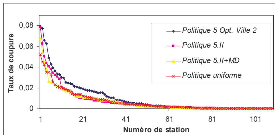
Figure 6.14 : Taux de coupure moyen par station (rangé dans l'ordre décroissant) pour les politiques uniforme, 5 Opt. Ville 2 , 5.II et 5.II+MD sur la zone de la ville 2.
