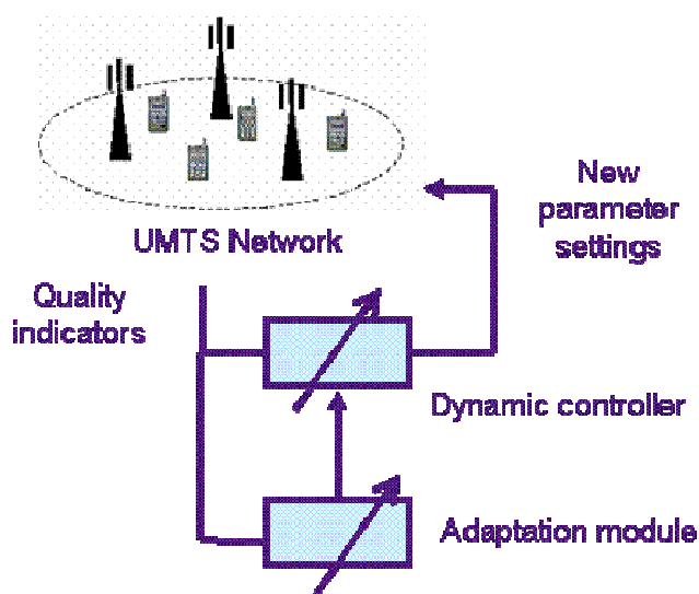
Figure 4.1 : Adaptation dynamique des paramètres des contrôleurs de logique floue
