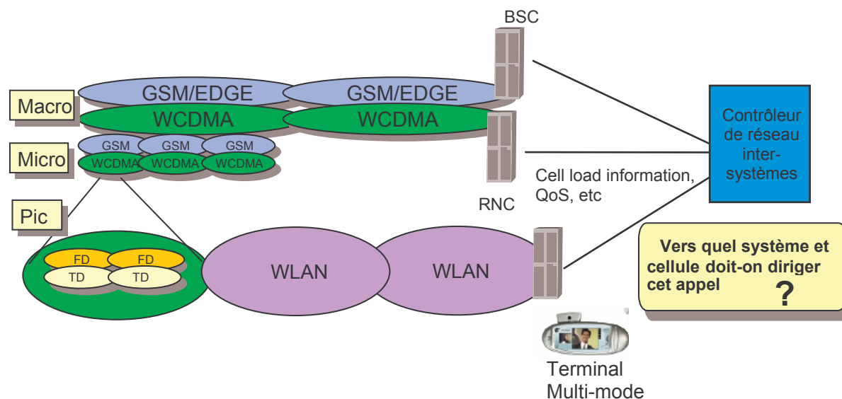
Figure 2.4 : Problème de la sélection de réseau pour la gestion coordonnée multi-systèmes
