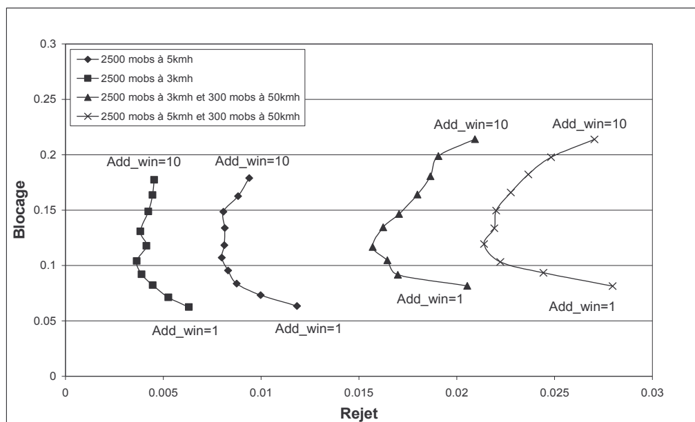
Figure 2.3 : Variations des taux moyens de blocage et de coupure en fonction du paramètre Add_win (statique et uniforme sur l'ensemble des stations) et du trafic
