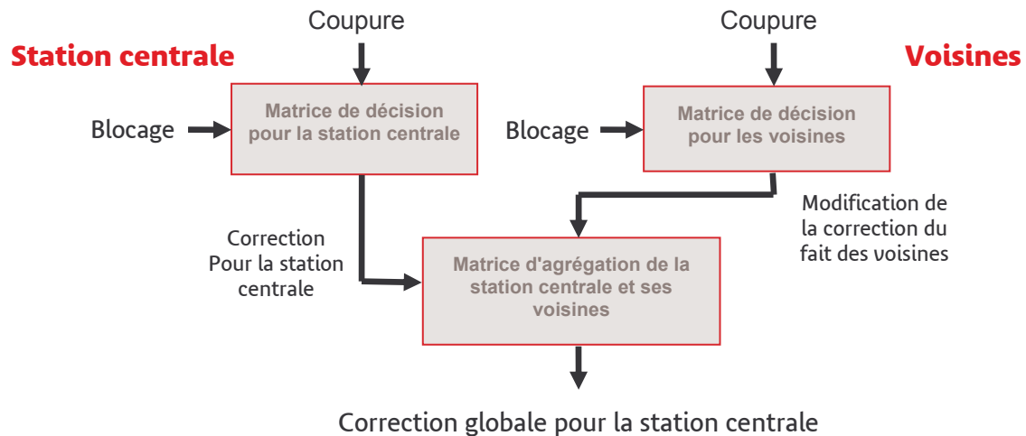
Figure 4.6 : Système de matrices de décisions pour le contrôle de l'algorithme d'admission
