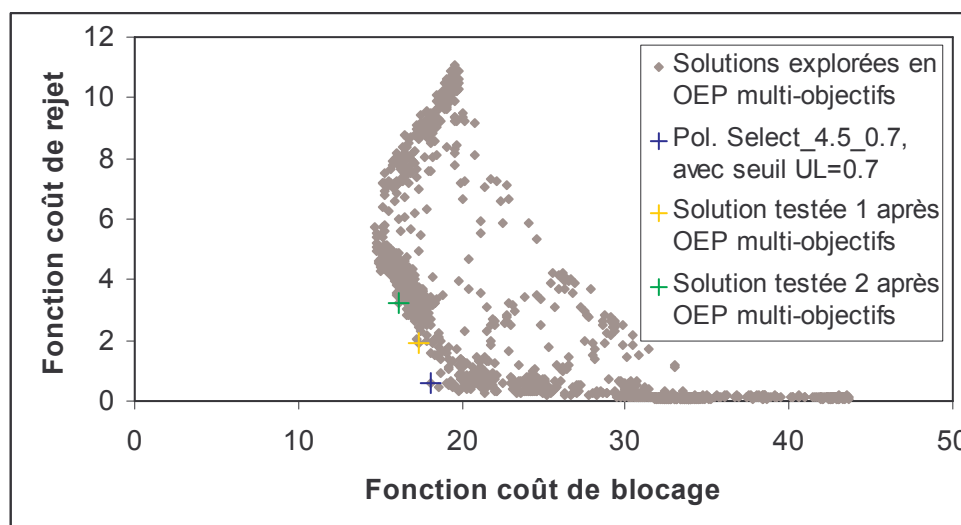
Figure 7.2 : Solutions explorées en OEP multi-objectifs (dont les solutions 1 et 2 du front optimal) comparées avec la politique Select_4.5_0.7 obtenue en mono-objectif pour un coefficient de mixage égal à 4.5 dans le plan fonction coût de blocage – fonction coût de coupure.
