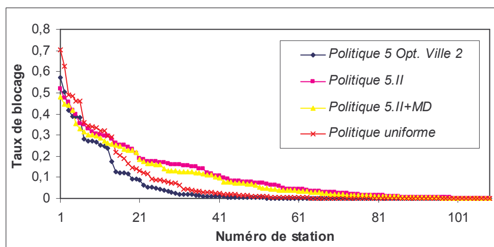
Figure 6.13 : Taux de blocage moyen par station (rangé dans l'ordre décroissant) pour les politiques uniforme, 5 Opt. Ville 2 , 5.II et 5.II+MD sur la zone de la ville 2.
