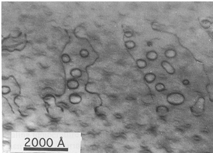
Figure 1.22 : Boucles d'Orowan de dislocations parfaites entourant les précipités \gamma' du Waspaloy déformé à 1,5 % à 650°C à une vitesse de 2.10^{-3} \text{ s}^{-1} [Guimier 1970]
