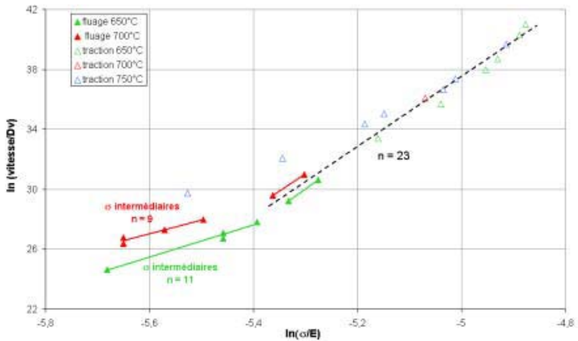
Figure 5.20 : Diagramme de Norton de l'Udimet 720 HS dans le domaine des contraintes fortes et intermédiaires établi à partir des essais de fluage et de traction
