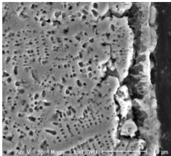
Figure 4.14 : Demi-coupe polie attaquée du fût de l'Udimet 720 HS, rompue en fluage à 650°C sous 750 MPa, t_f=1400h^1 - MEB
