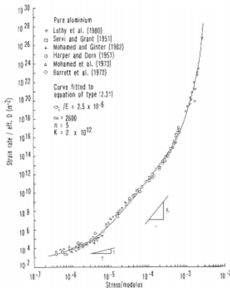
Figure 1.13 : Vitesse de déformation stationnaire de l'aluminium sur une large gamme de contraintes, d'après Wu et Sherby, [Nabarro 1995]
