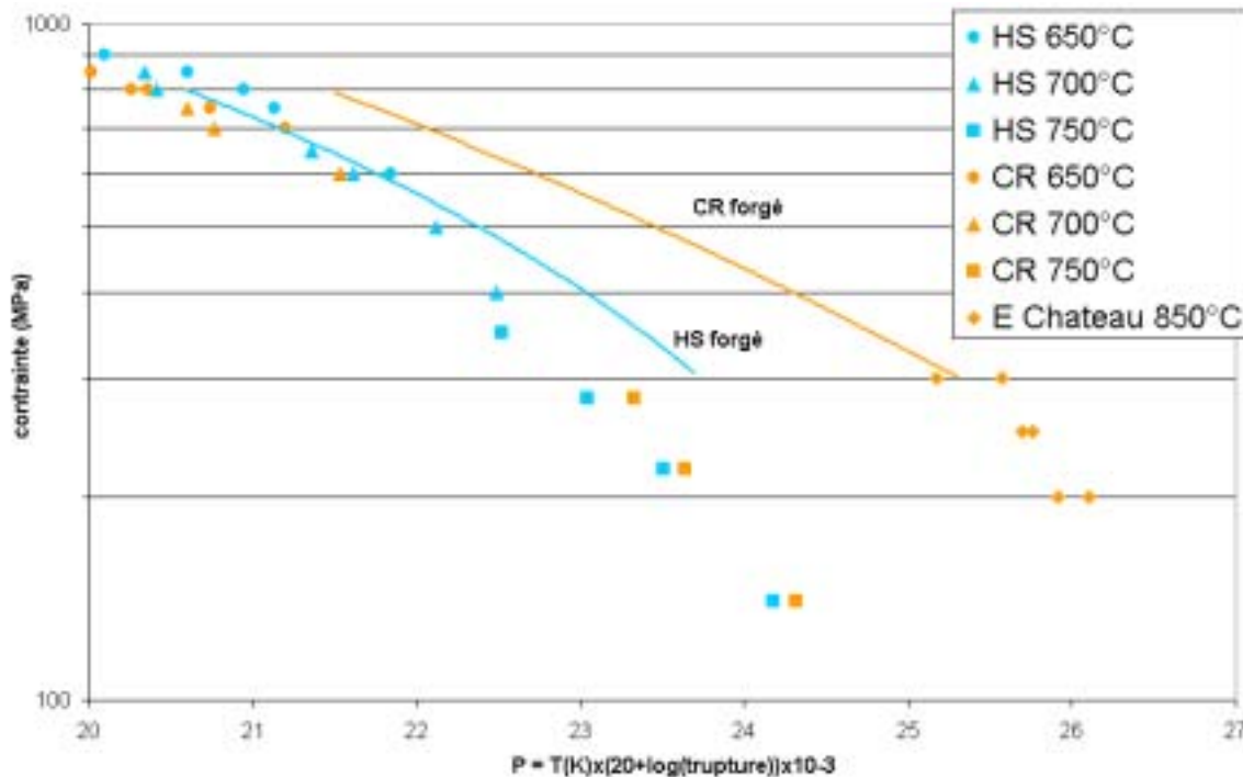
Figure 3.14 : Diagramme de Larson-Miller des résultats de fluage à 650°C, 700°C et 750°C de l'Udimet 720 HS et CR de l'étude, comparé à l'Udimet 720 forgé entre 400°C et 900°C (en trait plein) [Scerzernie 1988] et [Château 1999] à 850°C
