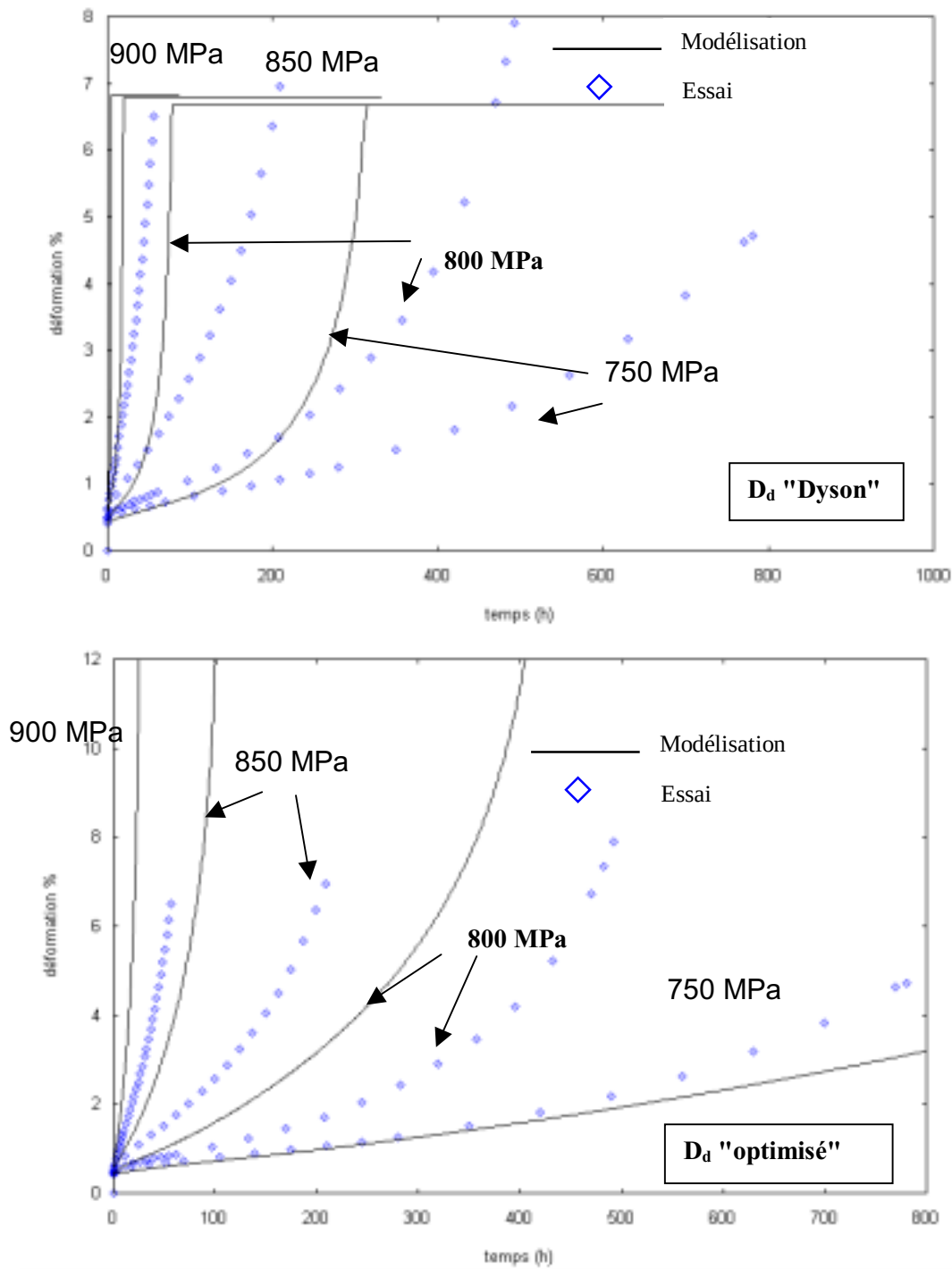
Figure 5.37 : Comparaison des courbes expérimentales et simulées de l' Udimet 720 HS en fluage à 650°C - Déformation totale vraie en fonction du temps
