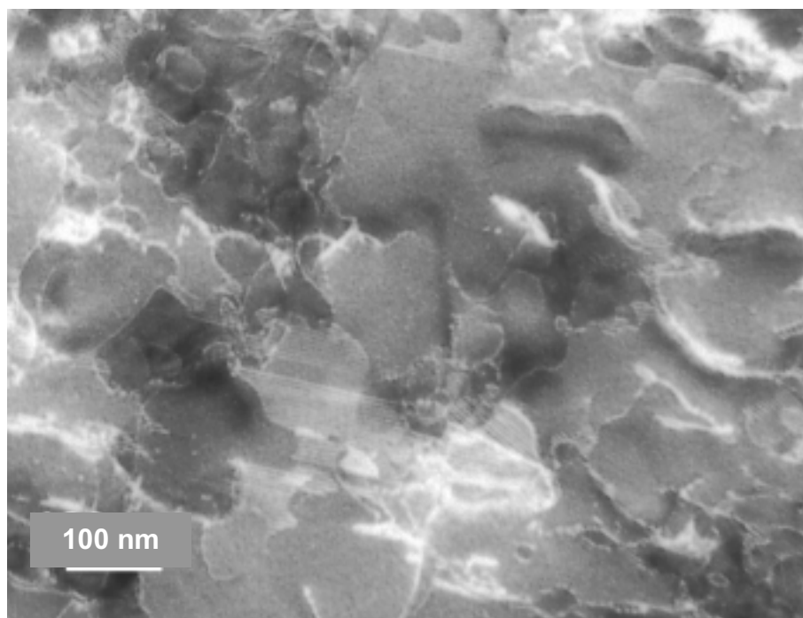
Figure 5.18 : Structure de dislocations observée dans l'Udimet 720 HS déformé de 1,6 % en traction à 650°C ( \dot{\epsilon} = 5.10^{-4} \text{ s}^{-1} ) - champ faible
