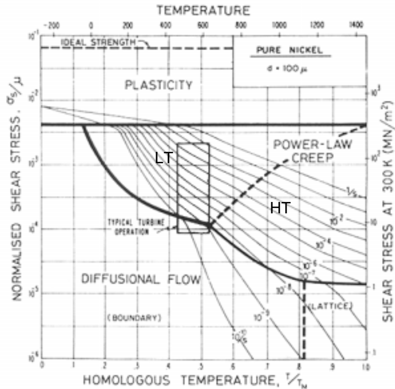
Figure 1.20a: Carte des mécanismes de déformation dans le cas du nickel pur de 100 \mu\text{m} de taille de grain [Frost 1982]
