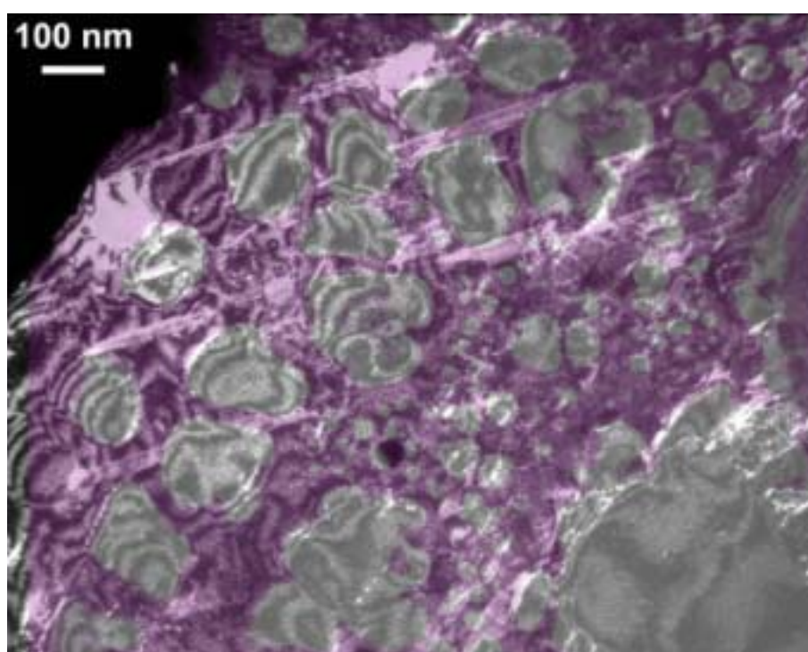
Figure 5.18 : Structure de dislocations observée dans l'Udimet 720 HS déformé de 1,6 % en traction à 650°C ( \dot{\epsilon} = 5.10^{-4} \text{ s}^{-1} ) - champ faible
