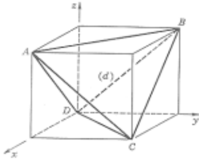
Figure B1 : Tétrahèdre de Thompson défini selon les axes cristallographiques \langle 111 \rangle d'un cube de côté a/2 [Hirth 1982]
