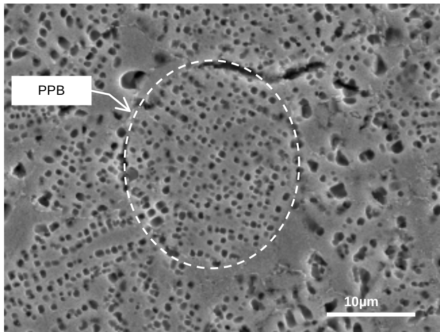
Figure 4.12 : Demi-coupe polie attaquée proche du faciès de rupture de l' Udimet 720 HS , 650^{\circ}\text{C} sous 750\text{ MPa} , t_r=1400\text{h}^2 - MEB
