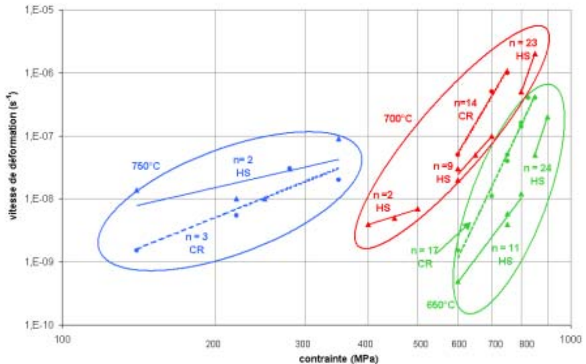
Figure 3.15: Représentation de la sensibilité de la vitesse à la contrainte : Évolution de la vitesse de déformation minimale ou stationnaire en fonction de la contrainte pour chaque température.
