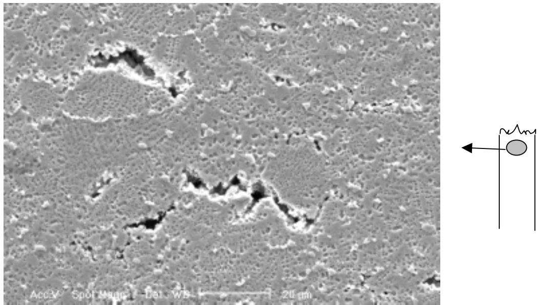
Figure 4.16 : Demi-coupe polie attaquée proche du faciès de rupture de l'Udimet 720 HS, 750°C sous 140 MPa, t_r = 2500 \text{ h} 4 – MEB
