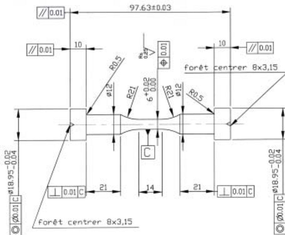
Figure D2 : Plan d'une éprouvette utilisée en relaxation
