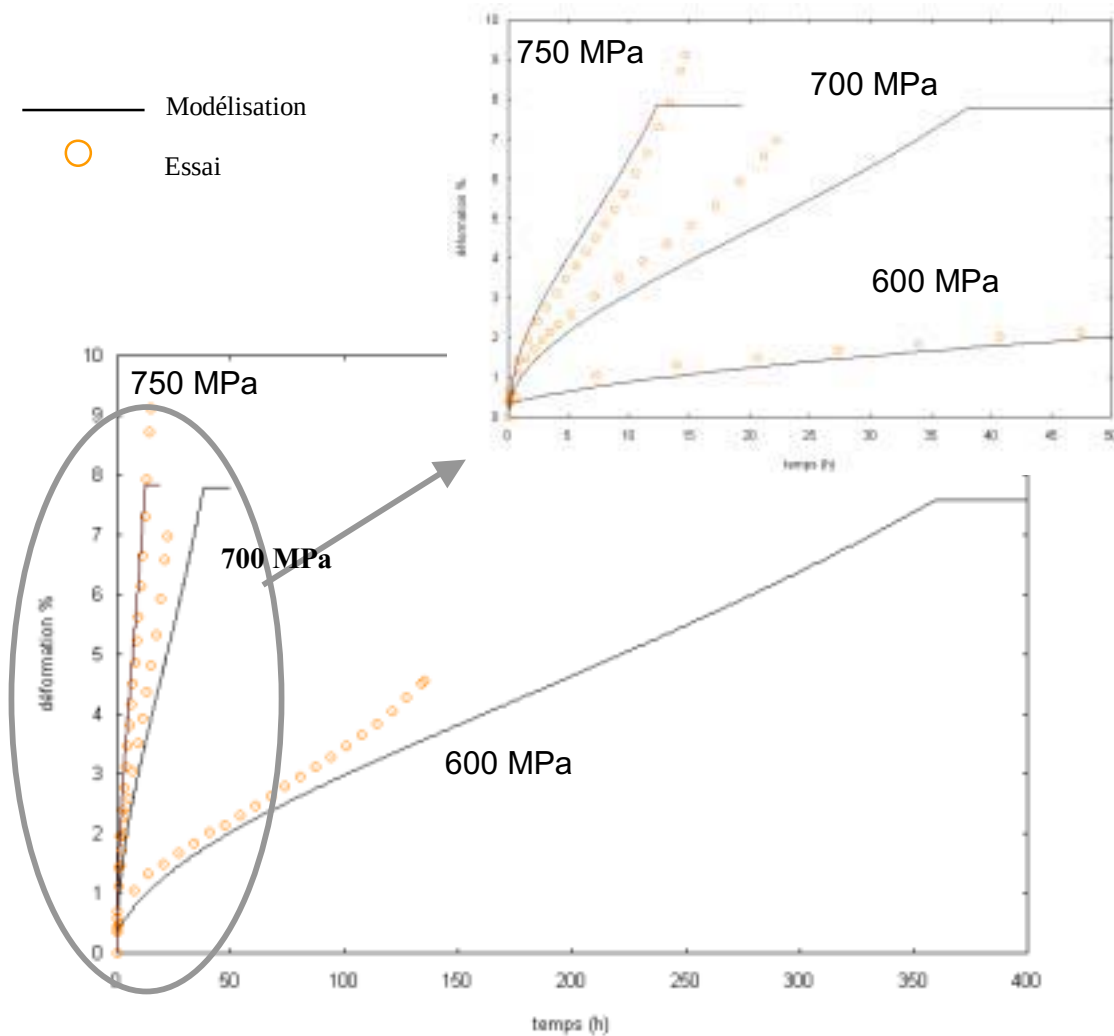
Figure 5.32 : Comparaison des courbes expérimentales et simulées de l' Udimet 720 CR en fluage à 700°C - Déformation totale vraie en fonction du temps Pas de paramètre de dommage
