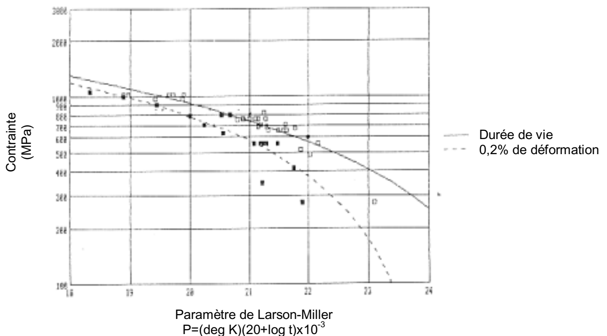
Figure 1.12 : Diagramme de Larson-Miller de l'Udimet 720 HS forgé établi pour le temps à rupture et le temps pour atteindre une déformation de 0,2 % [Sczerzernie 1988]
