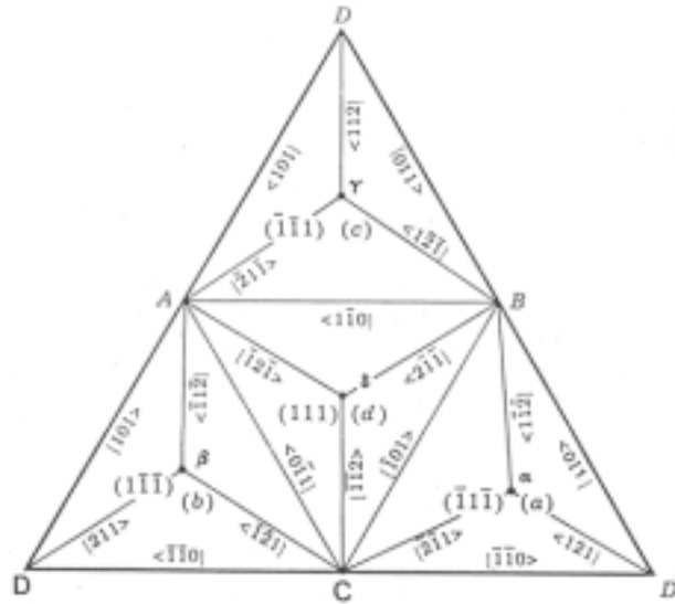
Figure B2 : Tétrahèdre de Thompson déplié à partir du sommet D. \overline{AB} correspond au vecteur a/2[-110] . Les partielles associées sont \delta B et A\delta , soit a/6[-211] et a/6[-12-1] [Hirth 1982]
