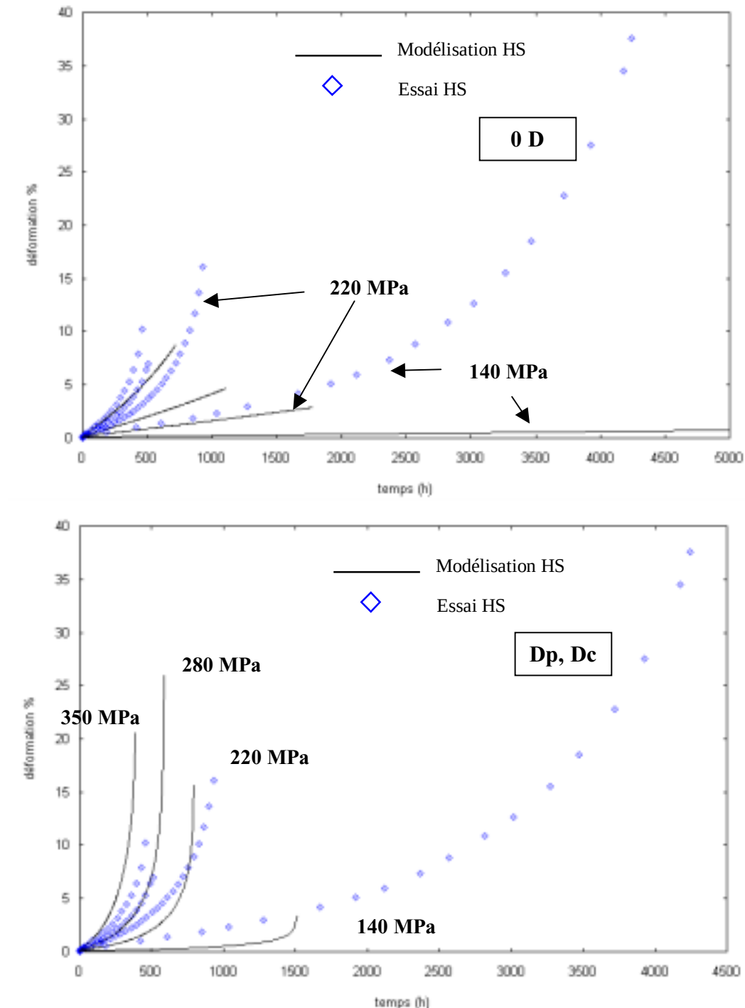
Figure 5.39 : Comparaison des courbes expérimentales et simulées de l' Udimet 720 HS en fluage à 750°C - Déformation totale vraie en fonction du temps Paramètre de dommage : cavitation et coalescence des précipités \gamma'
