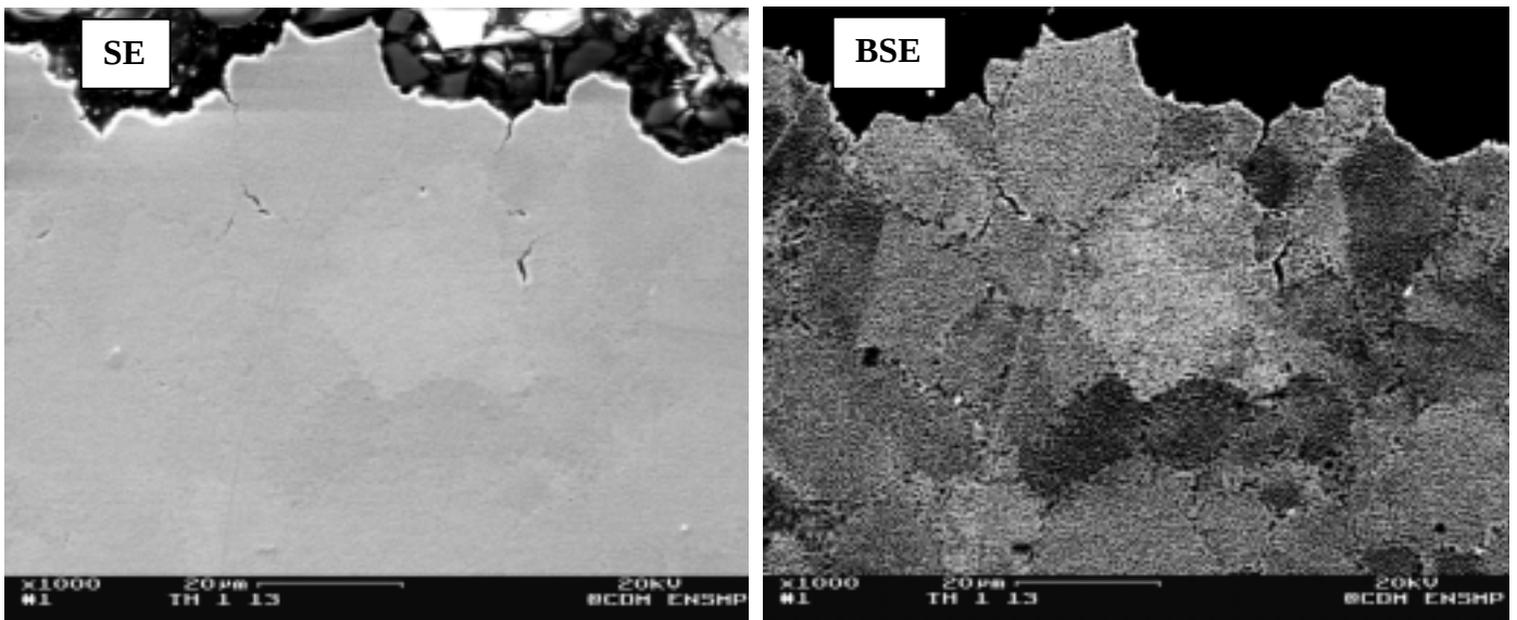
Figure 4.13 : Demi-coupe polie proche du faciès de rupture de l' Udimet 720 CR , 650^{\circ}\text{C} sous 800\text{ MPa} , t_r=90\text{ h} - MEB : cliché de gauche pris en électrons secondaires (SE) et cliché de droite pris en électrons rétrodiffusés (BSE)
