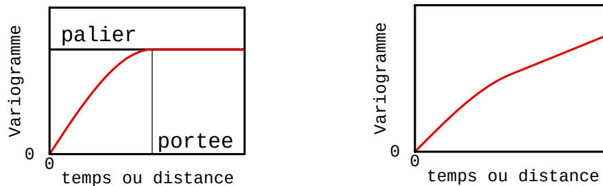
Figure 2 : Quelques modèles de variogramme. A gauche, palier et portée pour un modèle élémentaire, à droite : exemple de deux structures gigognes.
