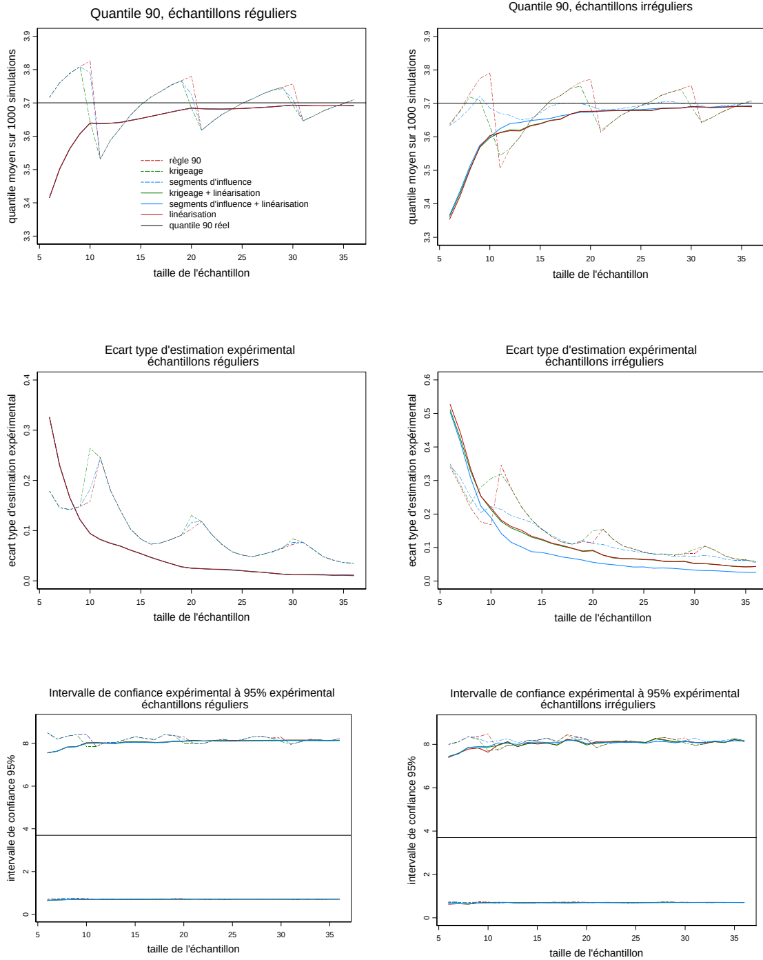
FIG. 6-3 : Variogramme périodique d'amplitude 20 et de période 365.25. A gauche, échantillons réguliers. A droite, échantillons irréguliers. De haut en bas : quantile 90 moyen sur 1000 simulations, Ecart type d'estimation expérimental, Intervalle de confiance expérimental à 95%.
