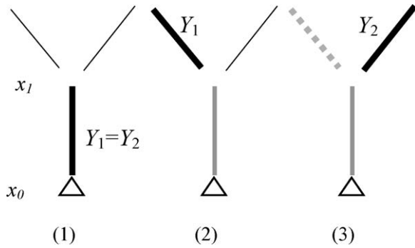
Fig. 3. Indépendance conditionnelle de Y_1 et Y_2 entre la confluence u_{IJ} et les sources. Trait noir épais, le segment en construction ; trait gris épais, les « données » utilisées pour le conditionnement ; tireté : poids de krigeage nuls.
