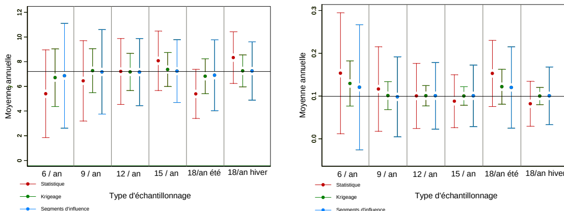
FIG. 6-7 : Estimation de la moyenne annuelle par 3 méthodes et intervalle de confiance à 95% prédit par chaque méthode. A gauche : Station 50500, nitrates, année 1985. A droite : Station 57800, nitrites, année 1996. Echantillonnage préférentiel et régulier. Les résultats par statistique classique sont présentés en rouge, par krigeage en vert et par segments d'influence en bleu, les indicateurs de référence en noir.
