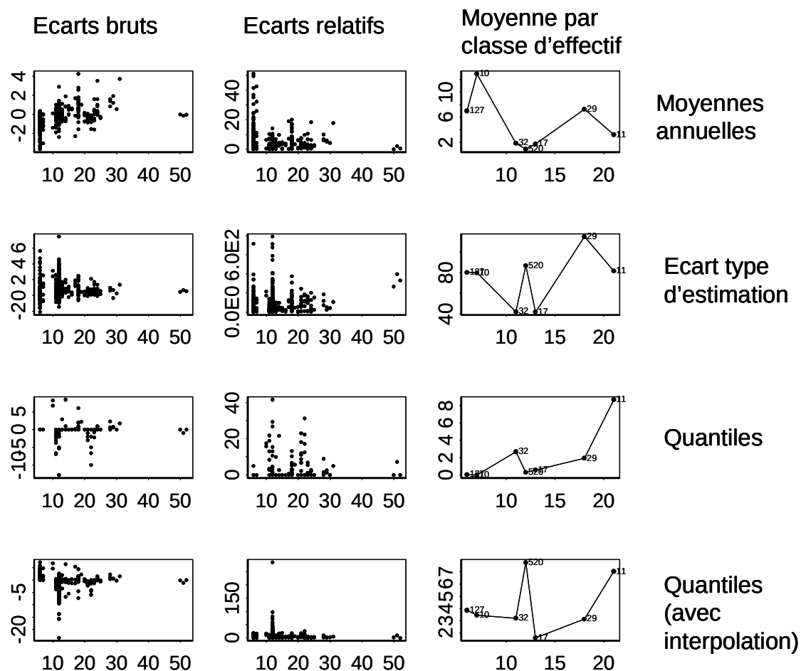
FIG. 7-2 : Ecart entre les estimations statistiques et géostatistiques par année pour les nitrates sur les 269 station RNB8 entre 2002 et 2004. Se reporter au début du paragraphe pour la lecture des graphiques.
