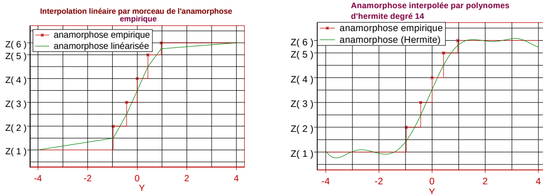
FIG. 5-9 : Exemple d'interpolation de l'anamorphose empirique. A gauche : par interpolation linéaire. A droite : par développement hermitien.
