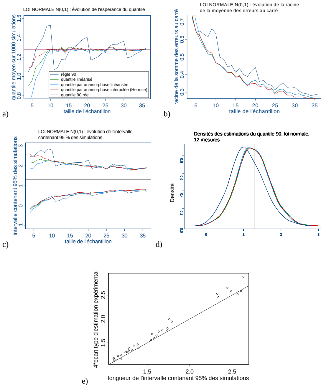
FIG. 5-10 : Evaluation du quantile 90 pour une loi normale ; calcul sur 1000 simulations. a) quatre estimateurs du quantile 90, en fonction du nombre de mesures. b) écart-type d'estimation. c) intervalle de confiance à 95%. d) histogramme des estimations pour un échantillon de 12 mesures. e) nuage de corrélation entre la longueur de l'intervalle de confiance à 95 % et 4 fois l'écart-type d'estimation.
