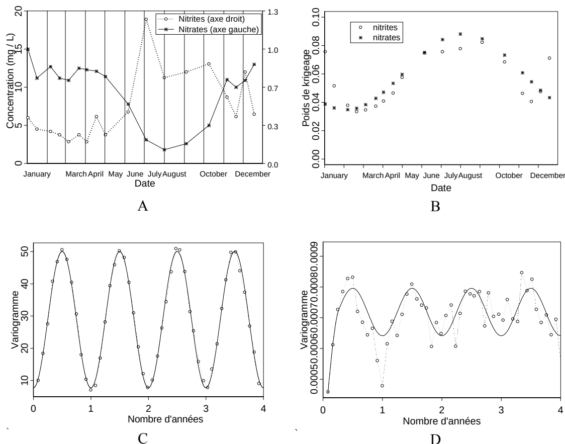
FIG. 4-1: A) Concentrations en nitrates et nitrites en 1995, station 56000 sur la Loire. B) Poids de krigage pour la moyenne annuelle, échantillonnage préférentiel avec doublement de la fréquence des mesures en période hivernale. C) Variogramme temporel des nitrates. D) Variogramme des nitrites.
