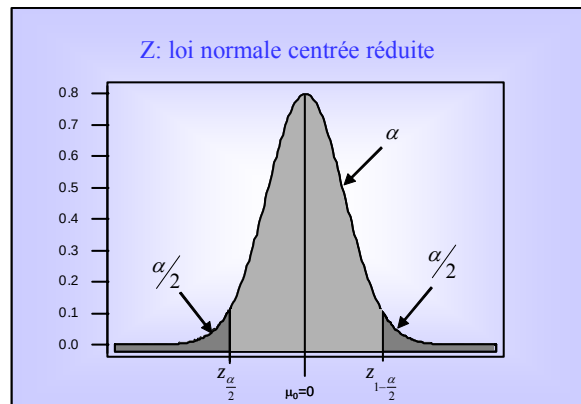
FIG. 3-1 : quantiles d'ordre \alpha/2 et 1 - \alpha/2 d'une loi normale centrée réduite
