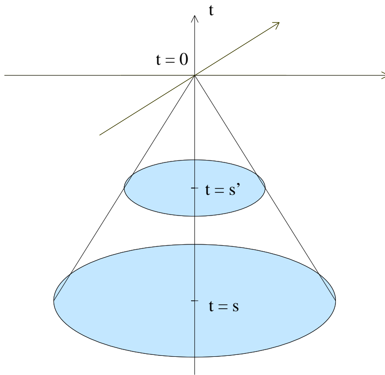
Figure 5.2: Le cône de lumière inverse issu de (0, 0) . On a colorié les disques D_s et D_{s'} .
