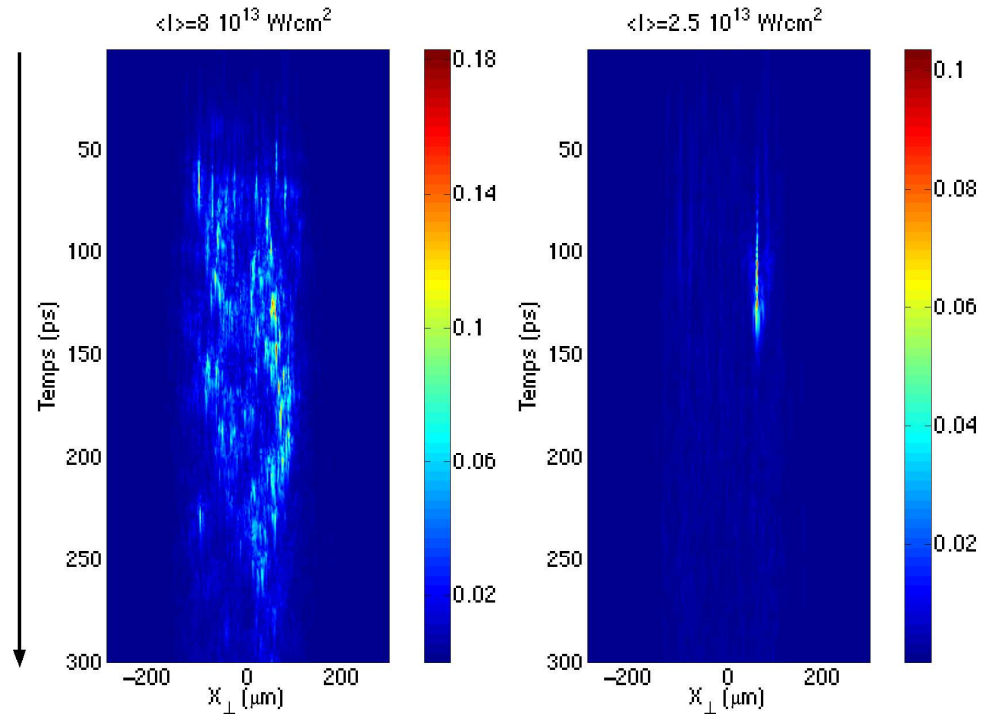
FIG. 4.11.: Diagnostics de type “camera streak” illustrant une coupe longitudinale (en z = -320 \mu m ) de la composante fondamentale des ondes sonores \sqrt{n_1/N_0} exprimée en fonction du temps (en picosecondes) et de la direction transverse (en \mu m ) pour \langle I \rangle = 8 \cdot 10^{13} \text{ W cm}^2 et \langle I \rangle = 2.5 \cdot 10^{13} \text{ W cm}^2
