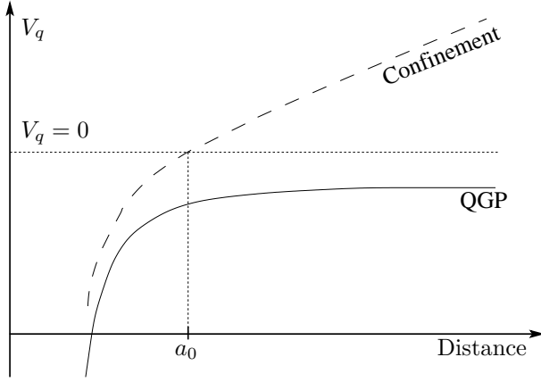
FIG. I.2 – Potentiel inter-quark V_{qq} en fonction de la distance r , a_0 est la taille d'un hadron. La courbe en pointillés représente le potentiel à T = 0 : lorsque la distance est grande la tension de la corde \sigma relie les quarks et les tient confinés. Lors de la création d'un PQG : la tension \sigma \rightarrow 0 et \alpha_s devient plus faible.
