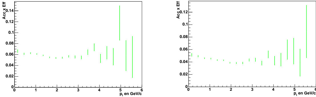
FIG. III.27 – Les corrections d'acceptance et d'efficacité en fonction de l'impulsion transverse p_t (en GeV/c) du J/\psi pour les bras sud (à gauche) et pour le bras nord (à droite).
