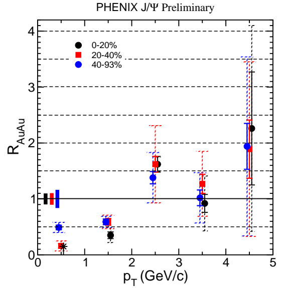
FIG. IV.20 – Facteur de modification nucléaire R_{AuAu} en fonction de l'impulsion transverse pour trois classes de centralité : 0-20 % (cercles noirs), 20-40 % (carrés rouges) et 40-93 % (losanges bleus). Les inertitudes liées à N_{coll} sont représentées par les barres verticales en noir pour 0-20 %, rouge pour 20-40 % et bleu pour 40-93 %.
