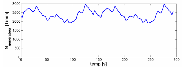
Fig. 9.16 Vitesse du générateur éolien
