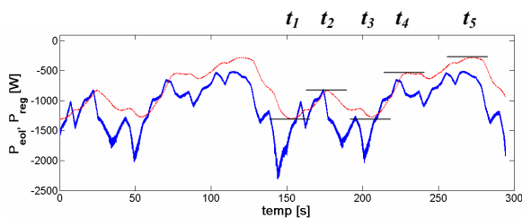
Fig. 9.46 Puissance générée (courbe continue) et puissance réglée (courbe pointillée), dans le cas du contrôle vectoriel
