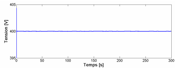
Fig. 6.60 Tension du bus continu
