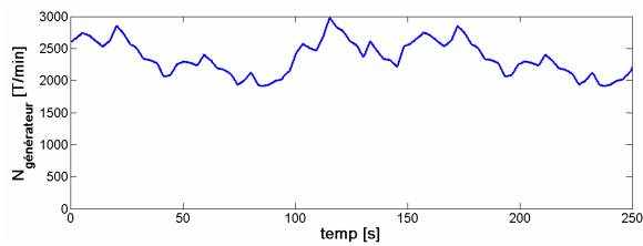
Fig. 9.4 Vitesse du générateur éolien
