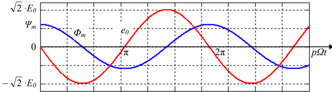
Fig. A.4.1 Enveloppes du flux magnétique et de la tension induite dans un enroulement
