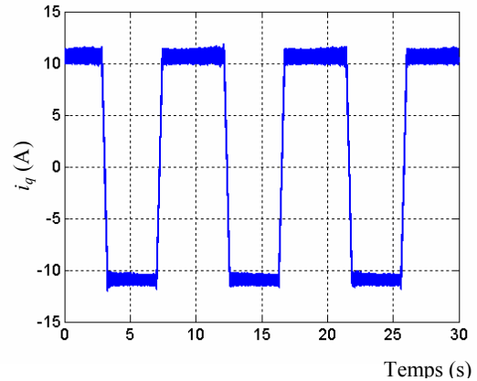
Fig. 8.12 Courant i_q de la MSAP pour \cos\phi = 1
