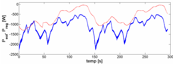
Fig. 9.23 Puissance générée (courbe continue) et puissance réglée (courbe pointillée)
