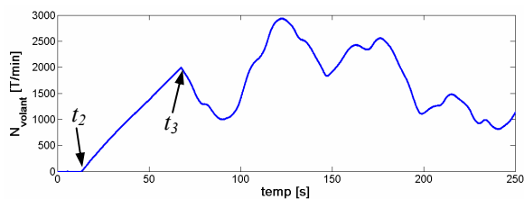
Fig. 9.9 Vitesse du volant d'inertie
