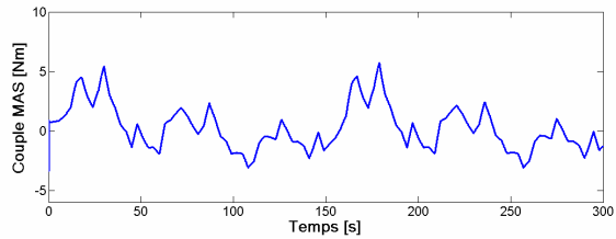
Fig. 6.53 Couple de la MAS
