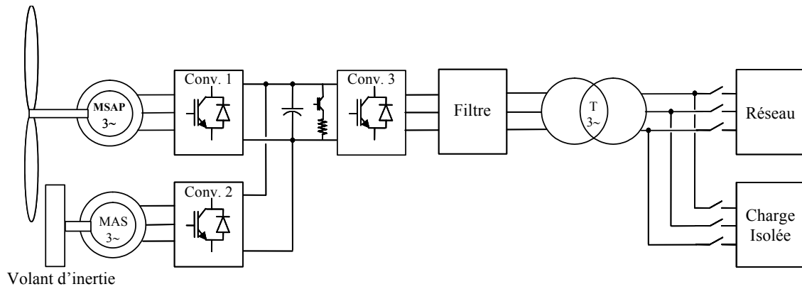
Fig. 5.4 Eolienne à vitesse variable associée à du stockage en vue d'un fonctionnement sur réseau ou sur charges isolées
