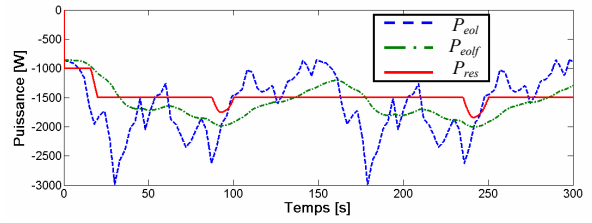
Fig. 6.86 Puissance générée, puissance générée filtrée et puissance envoyée au réseau (DTC pour la MAS et J = 3,6 \text{ kg}\cdot\text{m}^2 )
