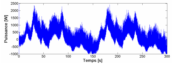
Fig. 6.89 Puissance du SISE
