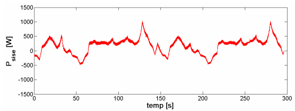
Fig. 9.32 Puissance de la MAS
