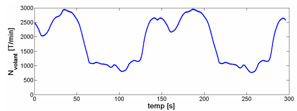
Fig. 9.33 Vitesse du volant d'inertie
