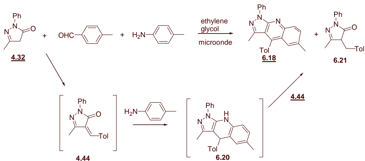
Figure 6- 12 : Réaction réalisée par Chacztrian et mécanisme proposé
