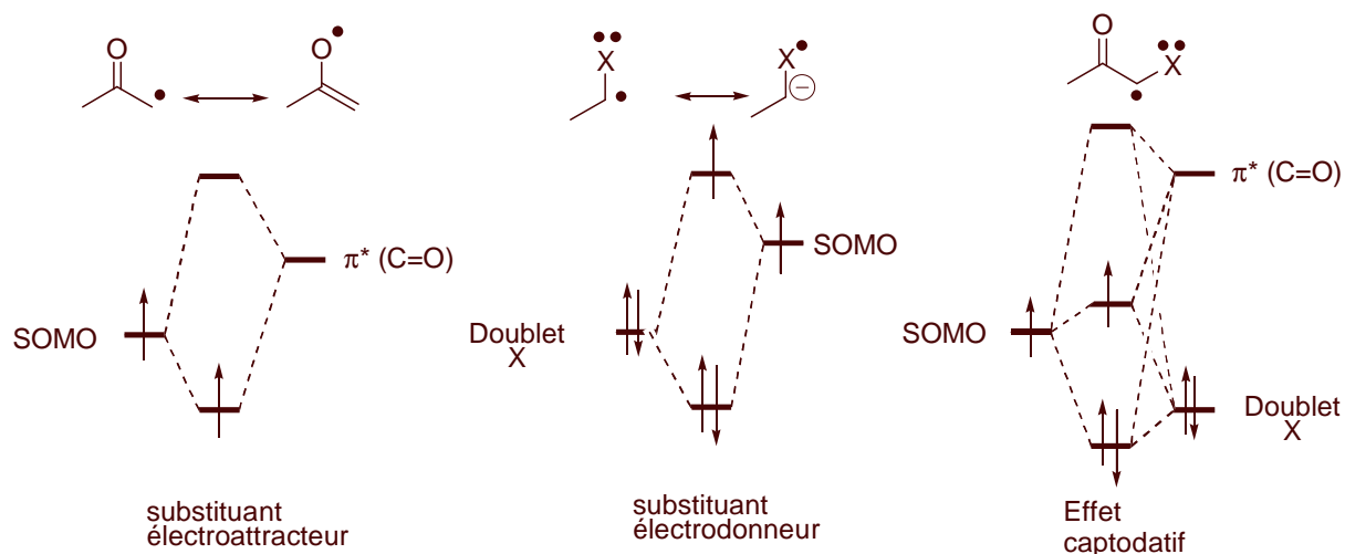
Figure 1- 3 : Stabilisation du radical par mésomérie en présence de substituants électro-donneurs et attracteurs
