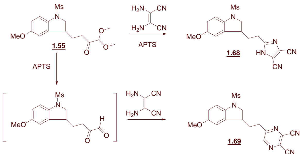
Figure 1- 38 : Réaction avec le diaminomaleonitrile
