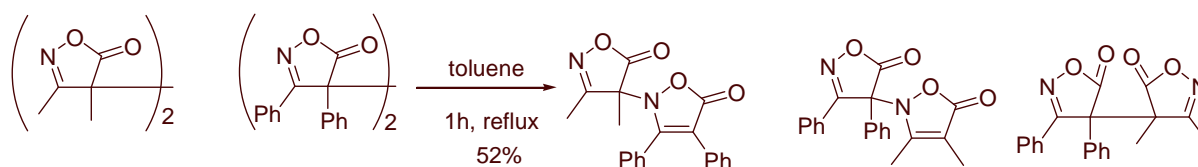
Figure 4- 25 : Visualisation de la dissociation de dimères effectuée par Twana Saleh
