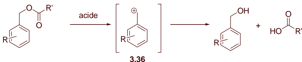
Figure 3- 34 : Décrochage en milieu acide
