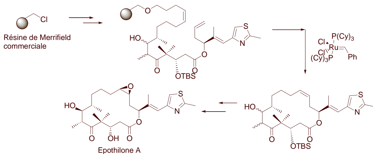
Figure 3- 3 : Synthèse de l'Ephilone A sur support solide par Nicolaou
