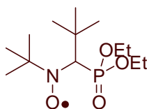
Figure 2- 17 : Structure de SG1
