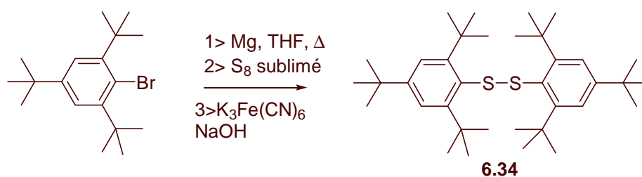
Figure 6- 21 : Synthèse du disulfure 6.34
