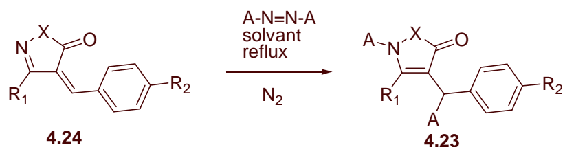
Figure 4- 20 : Etape d'addition radicalaire
