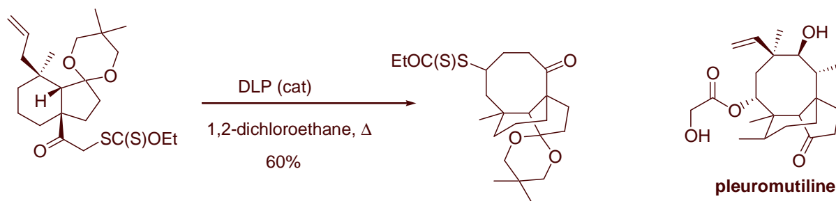
Figure 1- 19 : Formation du squelette tricyclique de la pleuromutiline
