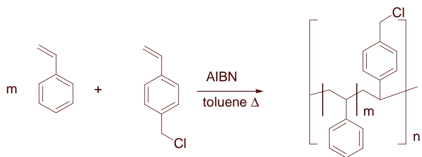
Figure 3- 8 : Synthèse des supports polystyrènes par copolymérisation
