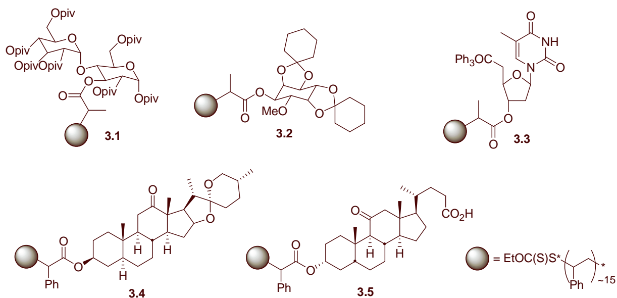
Figure 3- 10 : Substrats supportés complexes synthésisés par B.Sire et A. Wilczewska
