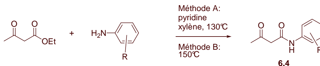
Figure 6- 4 : Synthèse des \beta -cétamide
