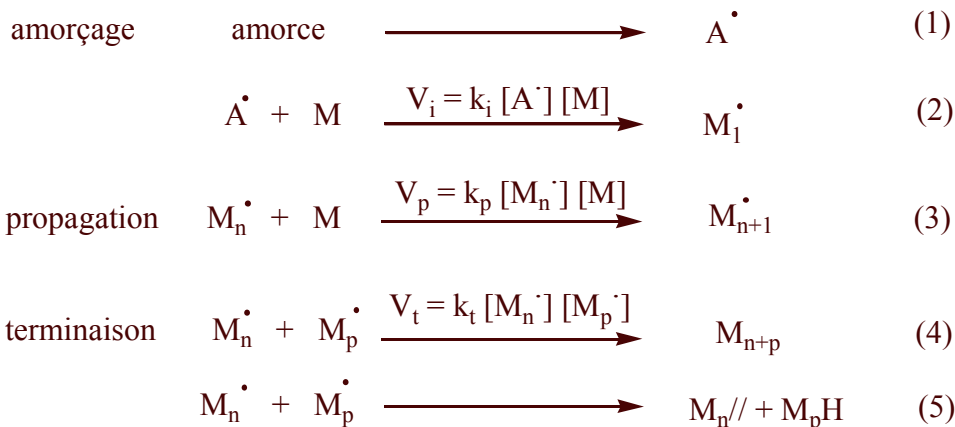
Figure 2-1 : Principe de la polymérisation radicalaire classique
