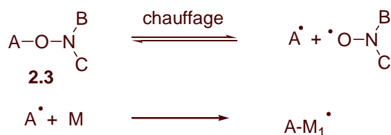
Figure 2- 16 : Amorçage de la NMP
