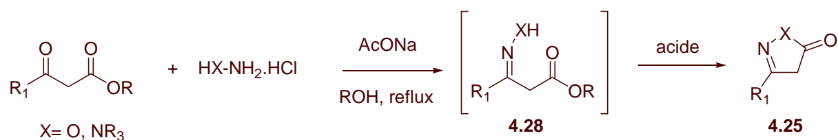
Figure 4- 18 : Synthèse des noyaux isoxazolones et dihydro-pyrazolones
