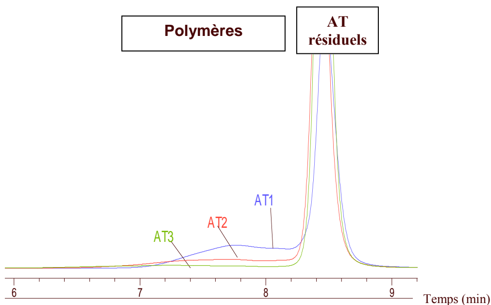
Figure 5- 7 : Superposition des spectres CES obtenus par détection UV (315nm) lors de la polymérisation du méthacrylate de méthyle en présence de AT1, AT2 et AT3. Polymérisations réalisées dans le toluène (ES= 30%) à 110°C et pendant 12h
