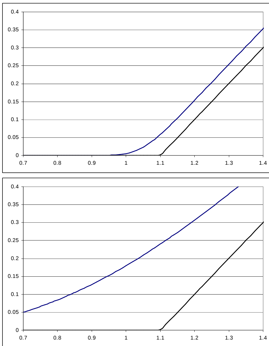
FIG. 3.5 – Prix du call dans le modèle de BLACK et SCHOLES; t = 0 , K = 1.1 , T = 1 , r = 0.05 ; \sigma = 0.05 (haut) ou 0.5 (bas)
