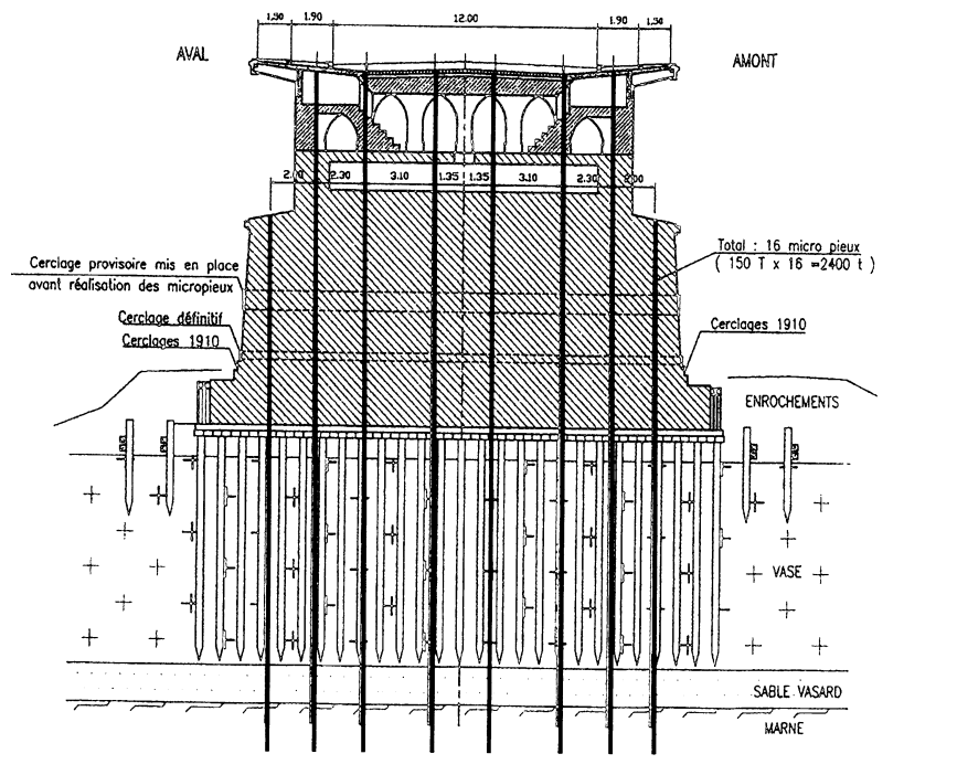
FIG. 1.3: Exemple de reprise en sous-œuvre par des micropieux : pile du pont de pierre à Bordeaux (Ledoux (1997) [55])
