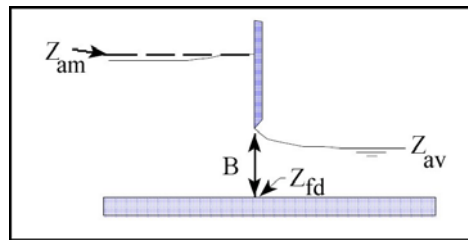
Figure 8.9 : Schéma simplifié d'une vanne (adapté de (USACE, 2005a)).
