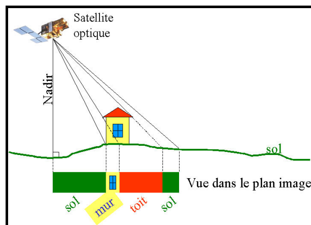
Figure 2.4 : Distorsions géométriques du au relief sur images optiques.
