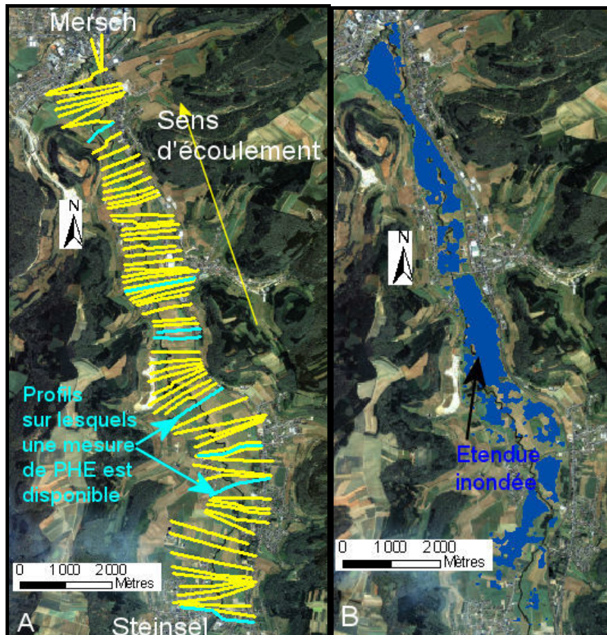
Figure 7.9 A et B : A) Profils en travers du modèle hydraulique 1D de l'Alzette (Matgen et al., 2004) et mesures de PHE, et B) étendue inondée extraite de l'image ENVISAT du 2 février 2003, sur fond d'une image satellitaire optique IKONOS (résolution spatiale 1m).
