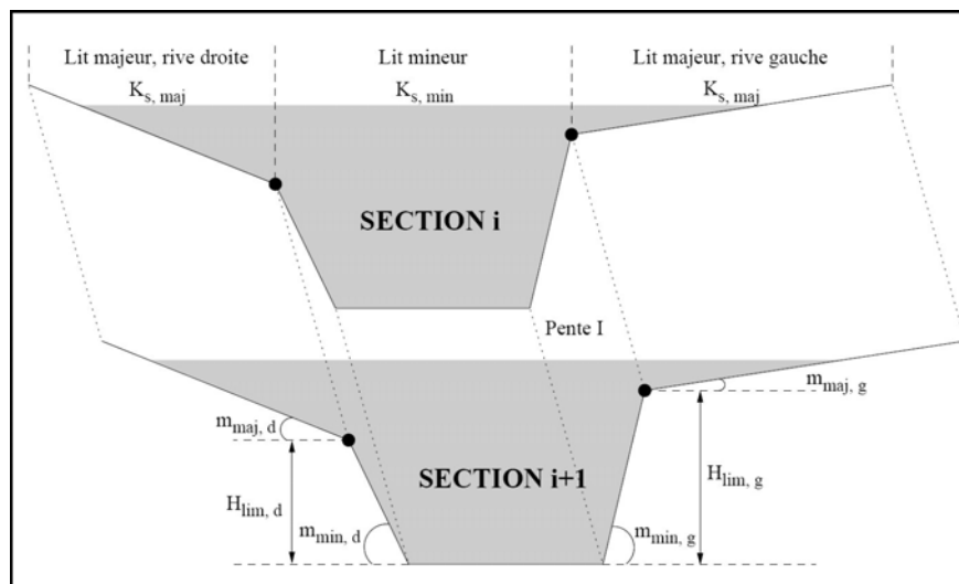
Figure 3.8 : Paramètres géométriques et de freinage à l'écoulement associés au modèle 1D à géométrie simplifiée (Roux et al., 2003).
