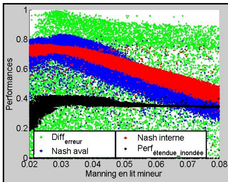
Figure 8.13 : Critères de performance de Nash, \text{Diff}_{\text{erreur}} , et \text{Perf}_{\text{étendue\_inondée}} obtenus à l'issue des simulations Monte-Carlo pour le Manning en lit Mineur (un point de chaque couleur par simulation, une couleur par critère).
