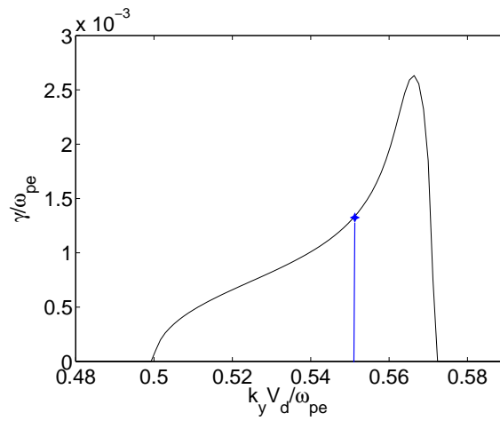
FIG. 2.17 – Position du mode k_y V_d / \omega_{pe} = 0.55 dans le lobe instable 1D n=5 .
