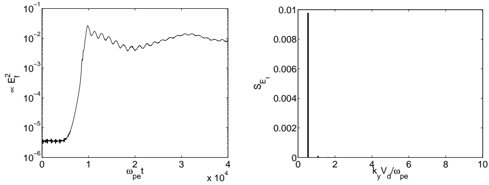
(a) Évolution temporelle de l'énergie électro- (b) Densité spectrale de puissance au temps statique \omega_{pe} t = 8 \cdot 10^3
