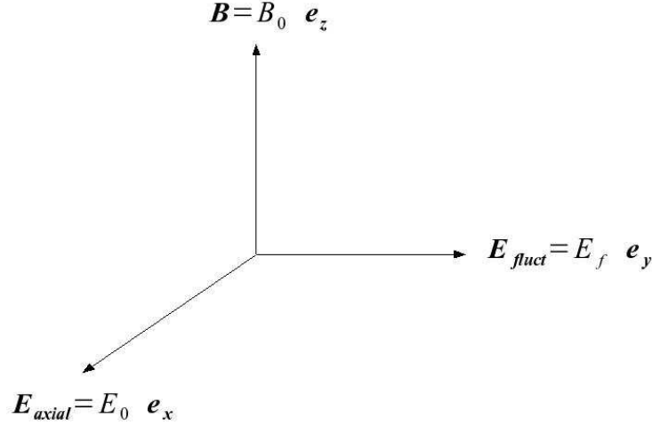
FIG. 6.1 – Configuration de champs électrique et magnétique dans laquelle évoluent les électrons.
