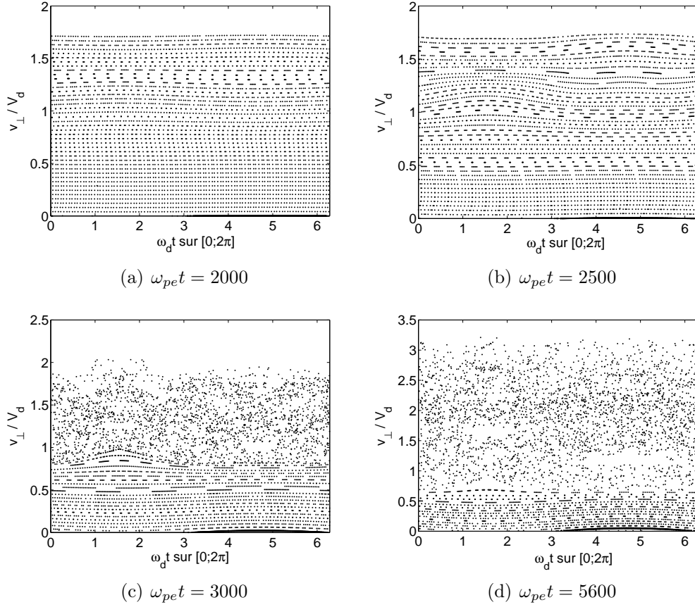
FIG. 7.5 – Apparition de la stochasticité pour le cas k_y V_d / \omega_{pe} = 1.04 .
