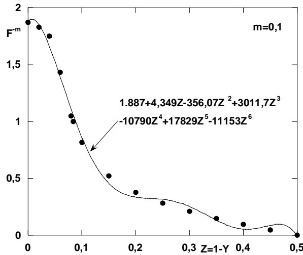
Figure A6-1.2: Evolution avec Z=1-Y de la fonction F^m caractérisant le gradient de pression dans la filière en conditions isothermes et régression polynomiale pour différentes valeurs de m
