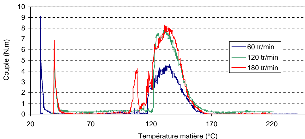
Figure 22 : Evolution de la consistance du savon XNa80 en fonction de la température et de la vitesse de rotation des rotors
