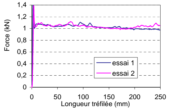
Filière \alpha=5^\circ
