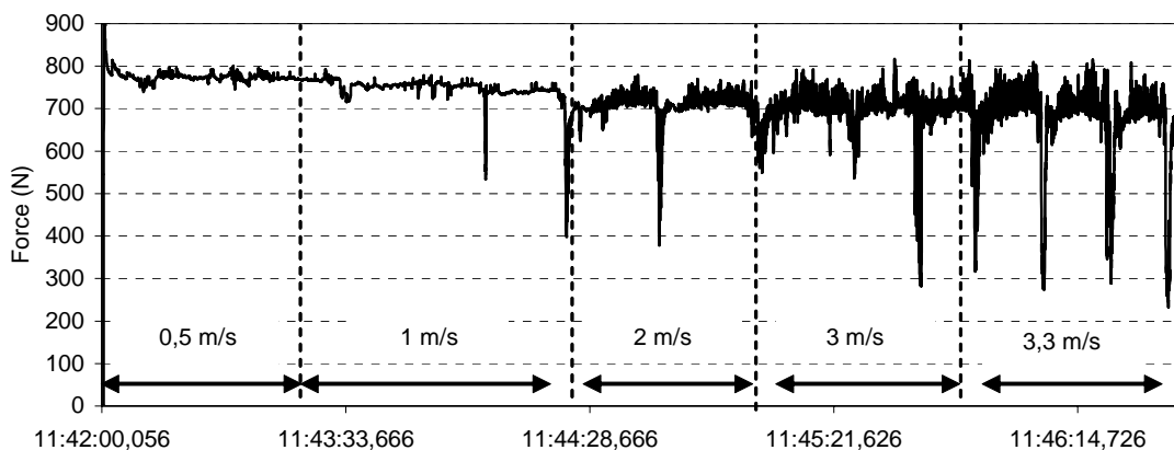
Figure 5 : Evolution de la force de tréfilage avec la vitesse [Fil 2R_e=2,2mm - Filière 2R_s=1,85mm/2\alpha=16^\circ - u = 0,5-3 m/s - savon XNa80]
