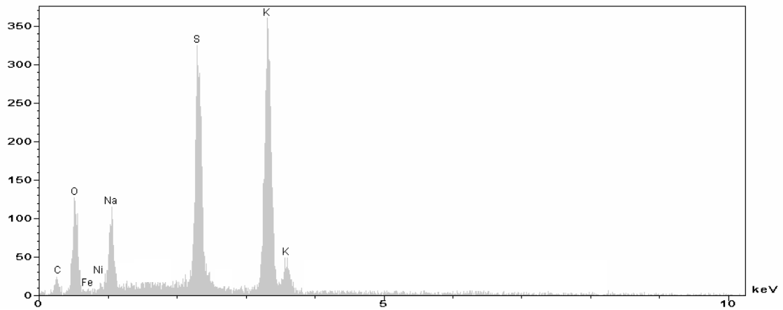
Figure 18 : spectre EDS de la zone grise de la figure 16 (revêtement salin)
