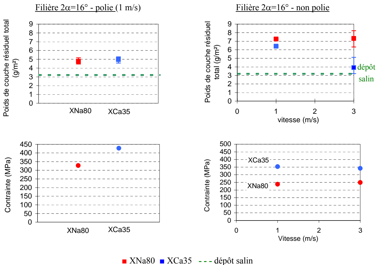
Figure 17 : Influence de l'état de surface de la filière sur le poids de couche résiduel total et la contrainte de tréfilage [Tréfileuse Marshal - u=0,5-3\text{m/s} - Acier AISI 304 Cu, 2R_e=2,2\text{ mm} - Filière 2R_s=1,85\text{ mm}/2\alpha=16^\circ ]
