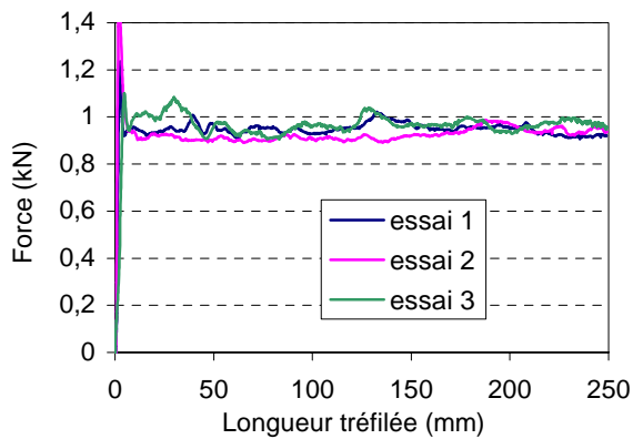
Filière \alpha=8^\circ
