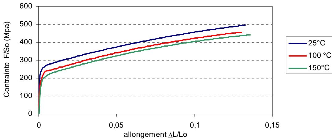
Figure 4 : Courbes de traction typiques obtenues avant tréfilage ( 2R_e=2,2mm ) - [Machine de traction Instron : vitesse de traction constante = 1mm/s - extensomètre 10mm]
