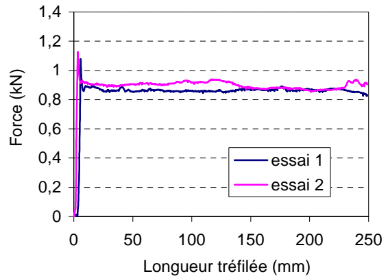
Filière \alpha=5^\circ
