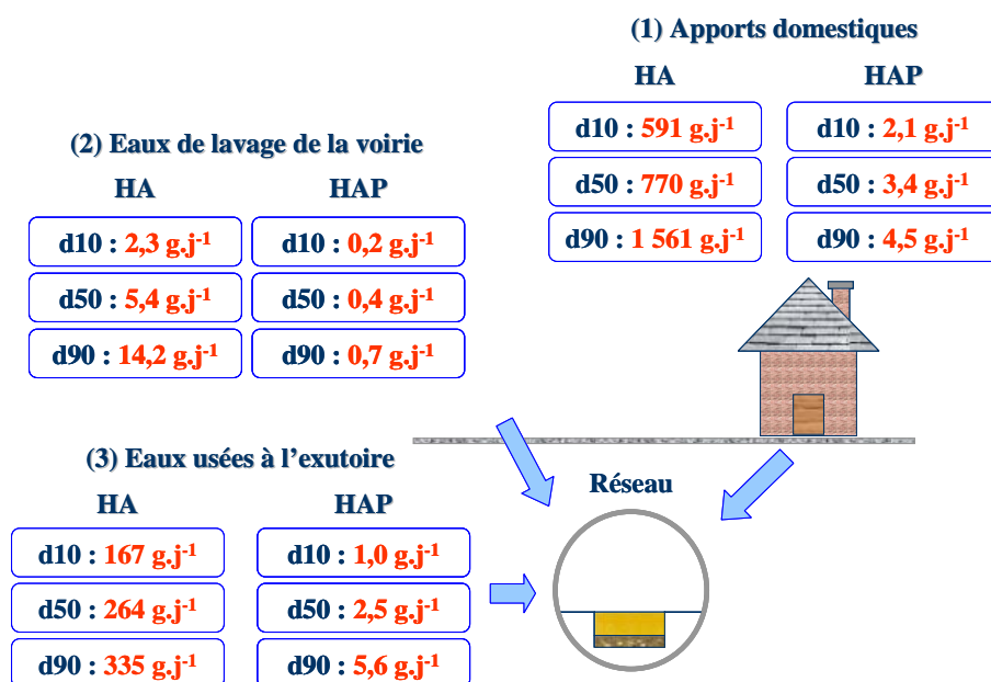
Figure III.14 : Flux en HA et HAP introduits quotidiennement dans le réseau via les apports domestiques et les eaux de lavage de la voirie à l'échelle du bassin versant du Marais
