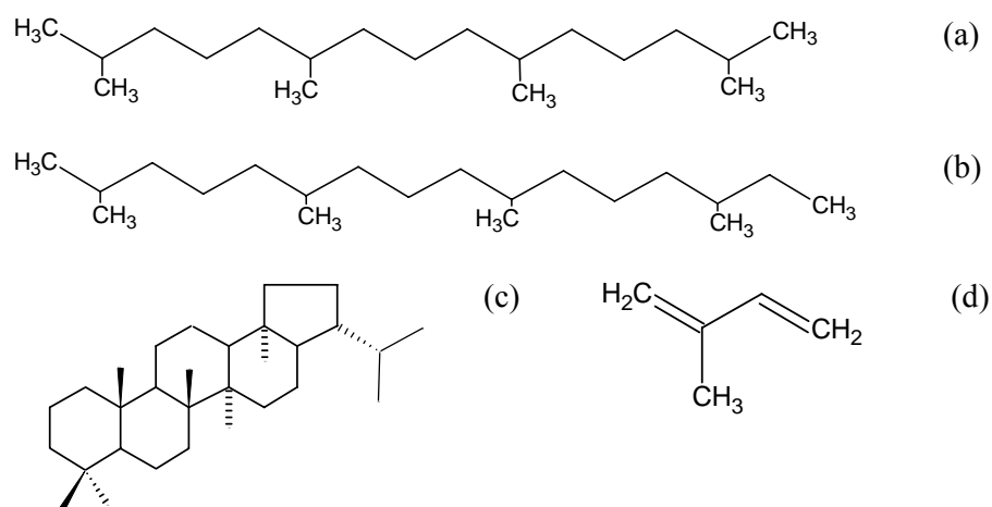
Figure I.2 : Structure des composés isoprénoïques, pristane et phytane (a et b), du squelette des hopanes (c) et de l'isoprène (d)
