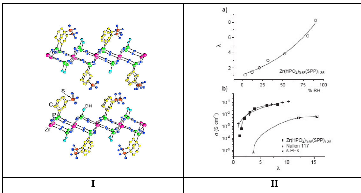
Figure 10 : I Modèle structural et II a) Nombre de molécules d'eau par groupe acide sulfonique ( \lambda ) en fonction de l'humidité relative, b) conductivité protonique en fonction de \lambda à 100^\circ\text{C} [28].
