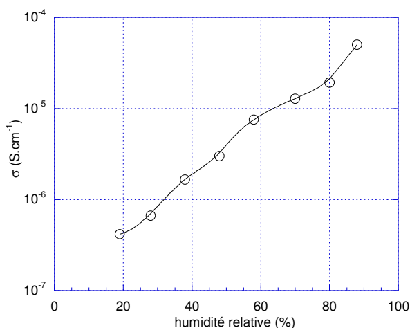
Figure 17 : Conductivité protonique \sigma de la poudre de zircone greffée à l'acide phosphorique en fonction de l'humidité relative avec laquelle elle a été équilibrée à 20 °C.
