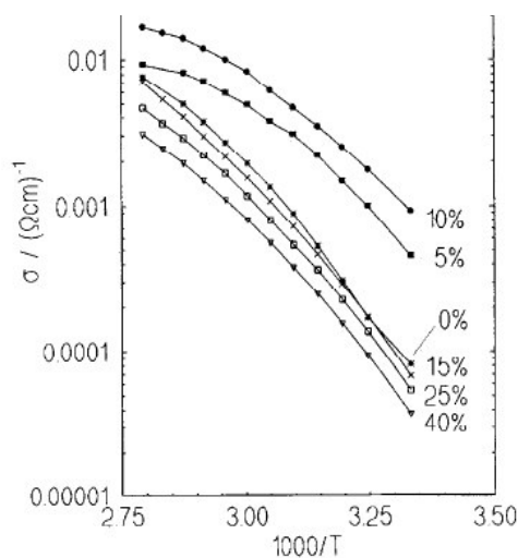
Figure 7 : Variation de la conductivité protonique en fonction de la température pour un système \text{H}_3\text{PO}_4 / PEI ( \text{PO}_4^{3-} / polymère = 1,5) avec différentes quantités de silice ajoutée [17].
