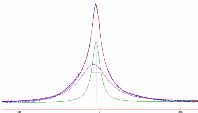
Figure 12 : Modélisation des pics obtenus dans le spectre RMN 1 H en statique de la poudre anhydre de zircone greffée à ASFP.
