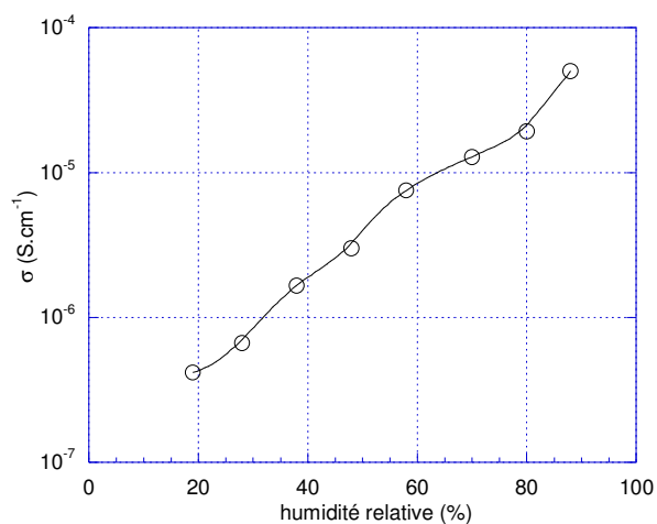
Figure 17 : Conductivité protonique \sigma de la poudre de zirconie greffée à l'acide phosphorique en fonction de l'humidité relative avec laquelle elle a été équilibrée à 20 °C.
