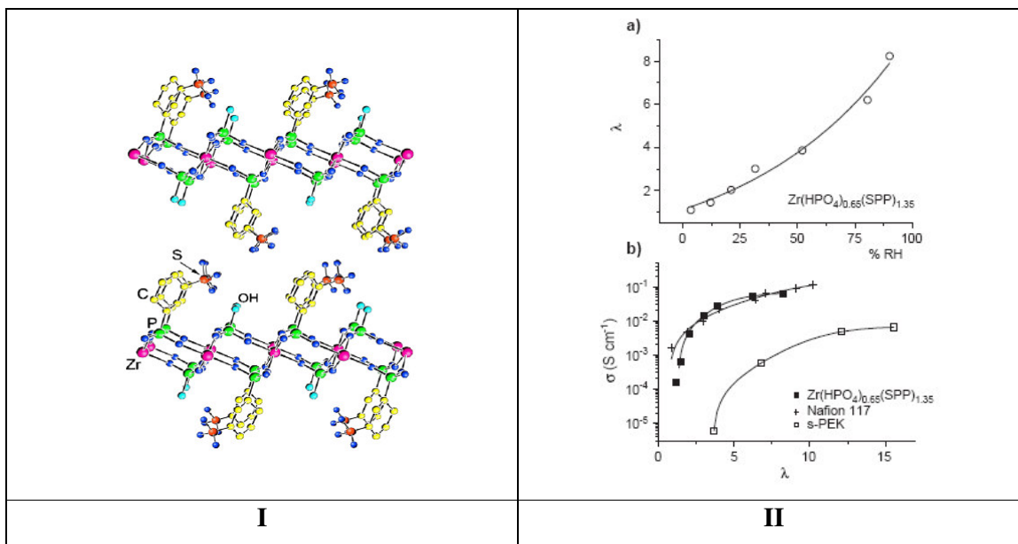
Figure 10 : I Modèle structural et II a) Nombre de molécules d'eau par groupe sulfonique ( \lambda ) en fonction de l'humidité relative, b) conductivité protonique en fonction de \lambda à 100 °C [28].
