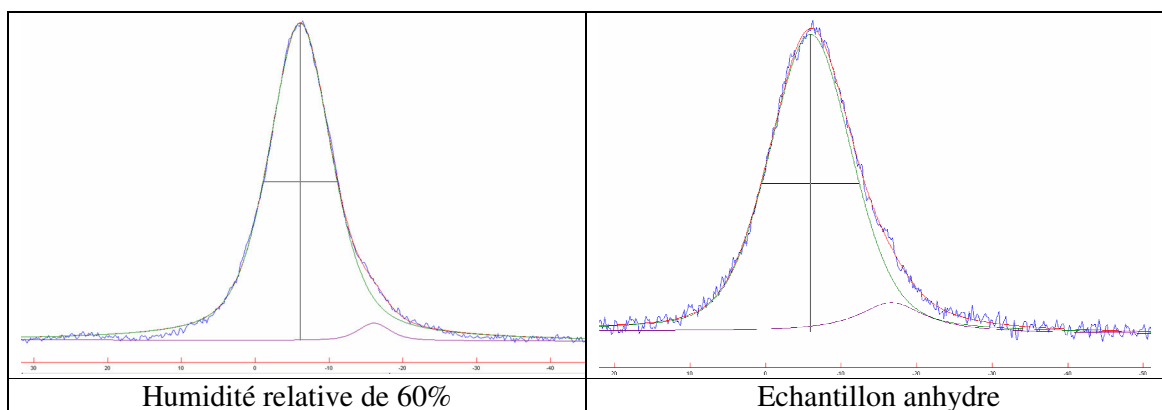
Figure 33 : Modélisation des pics contenus dans le spectre RMN ^{31}\text{P} de la zirconce greffée à l'ASFP.
