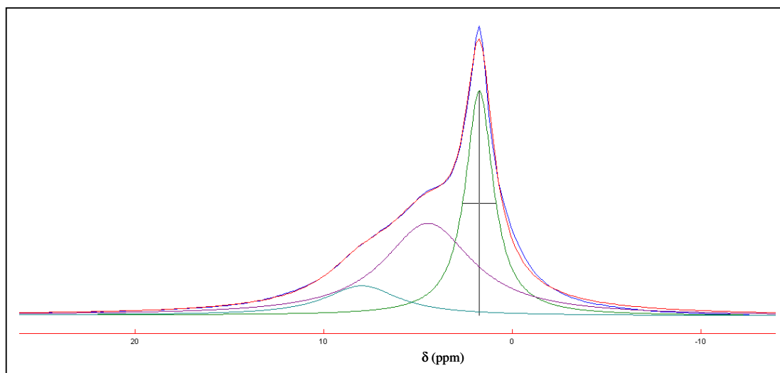
Figure 8 : Modélisation x des pics contenus dans le spectre RMN 1 H en rotation de la poudre de zirconne anhydre.
