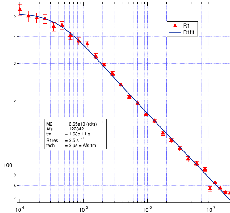
Figure 24: Efficacité de relaxation R_1=1/T_1 en fonction de la fréquence, obtenue par l'expérience de relaxométrie sur la poudre anhydre de zircon greffée à l'ASFP. La seule différence avec la Figure 22 est que le tracé a été effectué ici en échelle logarithmique ce qui permet de mieux apprécier la pente. Le trait plein représente la modélisation.
