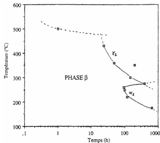
Figure I-16 : Diagramme Temps-Température-Précipitation [17]
