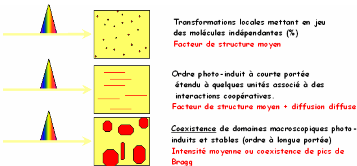
Figure 1.14 : Processus de croissance apparaissant sous irradiation lumineuse.
