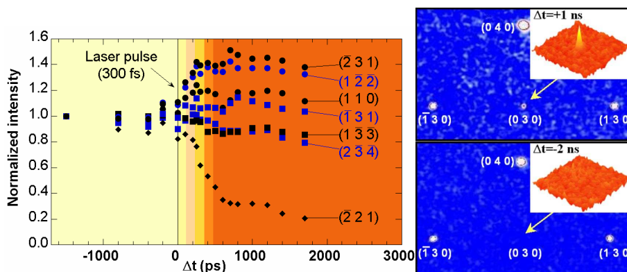
Figure 4.6 : Intensités normalisées de quelques pics de Bragg pour un délai entre la pompe laser pulsé (1.55 eV, 800 nm) et la sonde pulsé X variant entre -1 ns et +2 ns par pas de 100 ps (à gauche). (A droite) Apparition de la raie (030) caractéristique d'un ordre ferroélectrique intermédiaire +1 ns après l'impulsion laser. Le monocristal était excité à 90 K dans la phase N haute température (Collet (2003)).
