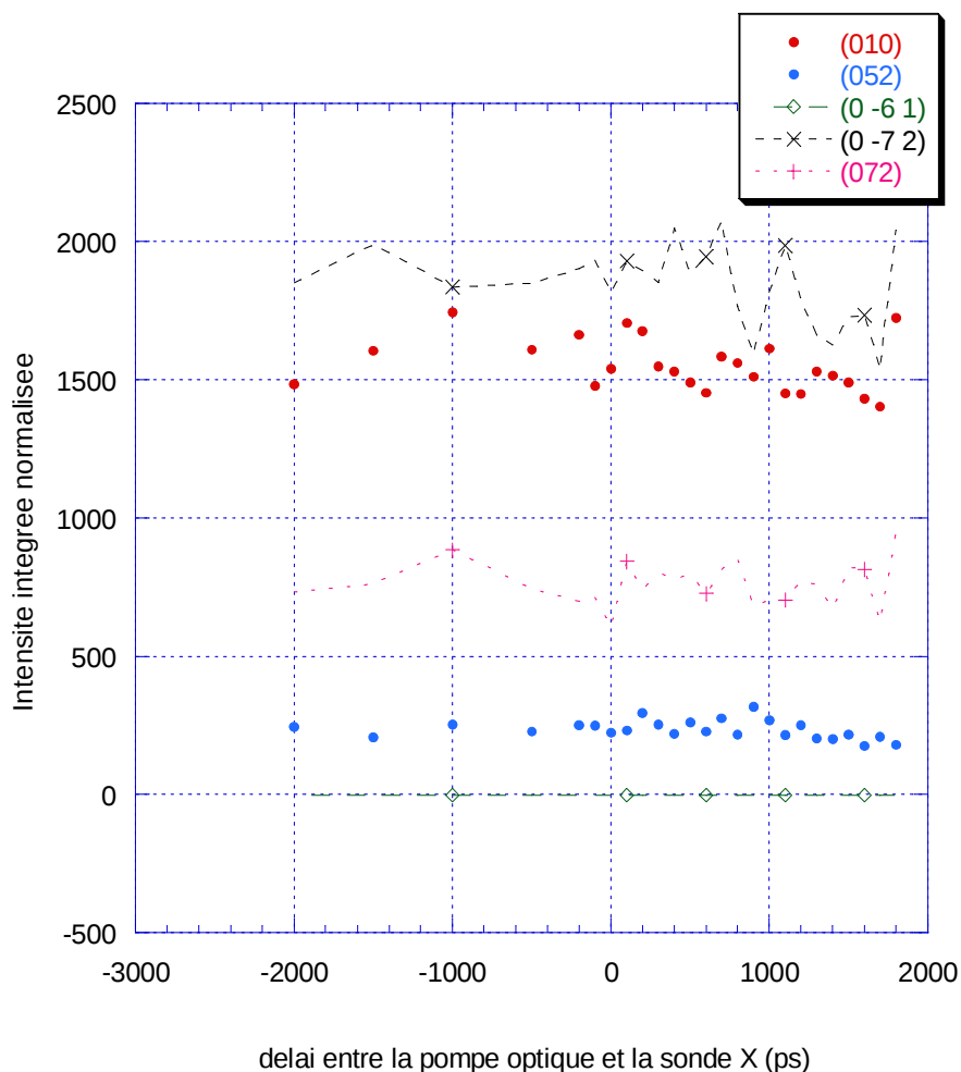
Figure 3.39 : Evolution de l'intensité après normalisation de quelques pics de Bragg du composé (\text{EDOTTF})_2\text{PF}_6 en fonction du délai entre la pompe optique et la sonde X.
