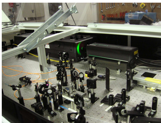
Figure 3.27 : Description de l'ancienne chaîne laser de la ligne ID09 de l'ESRF.
