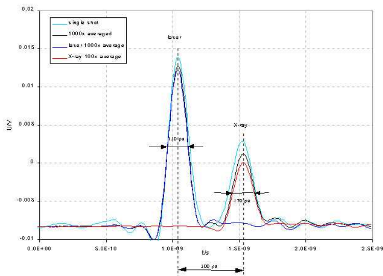
Détection du pulse laser et du pulse X par la diode GaAs. Le zéro temporel peut être déterminé à 60 ps près ( http://www.esrf.fr/exp_facilities/ID9/id9.html ).
