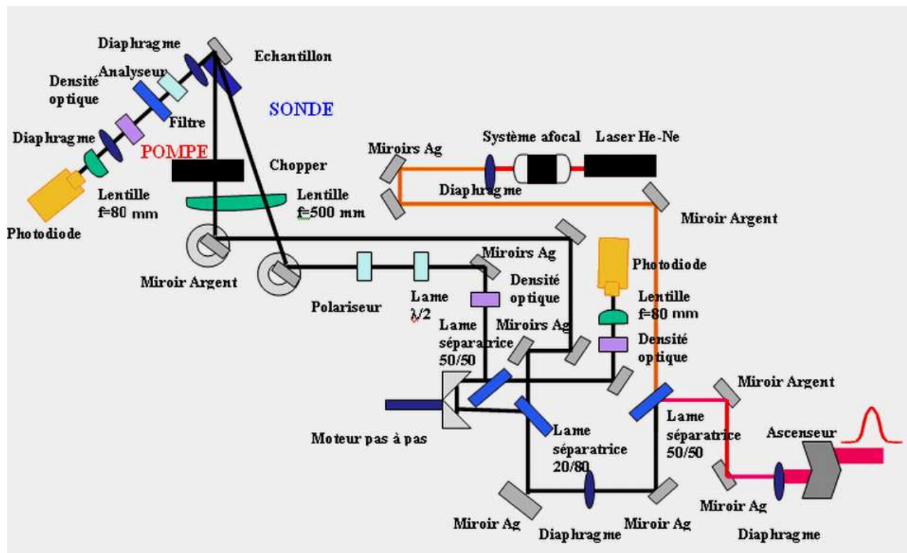
Figure 3.2 : Chemin optique du dispositif expérimental de spectroscopie pompe sonde.
