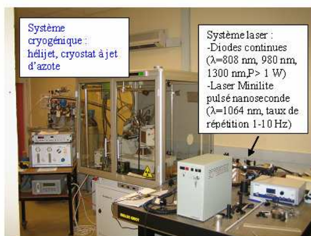
Figure 2.20 : Schéma du dispositif expérimental de diffraction X sous irradiation laser (par diodes continues ou laser pulsés) et sous basse température (hélium ou azote).
