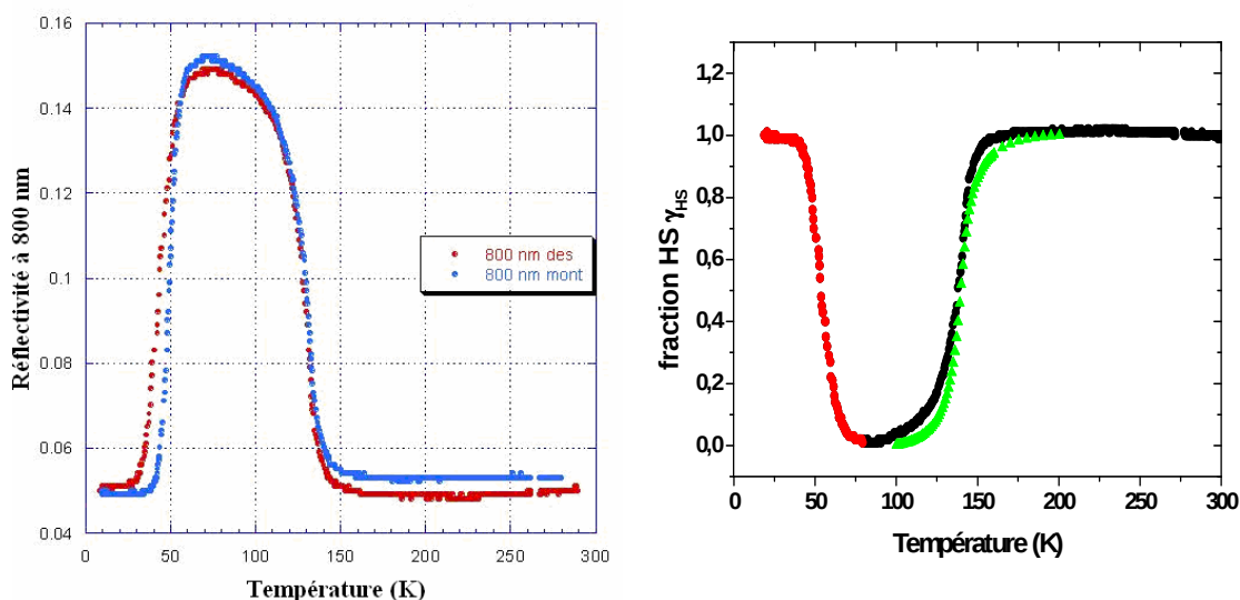
Figure 2.27 : Courbe de réflectivité à 800 nm en fonction de la température pour le composé \text{FeDPEA}(\text{NCS})_2 en descente et en remontée en température (gauche).
