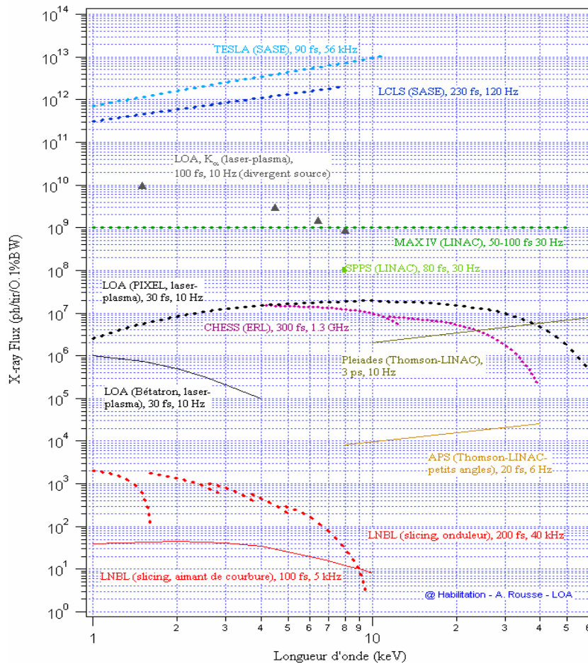
Figure 1.21 : Comparaison en terme de flux en fonction de la longueur d'onde entre différentes sources de rayonnement X pulsés (habilitation Antoine Rousse LOA).
