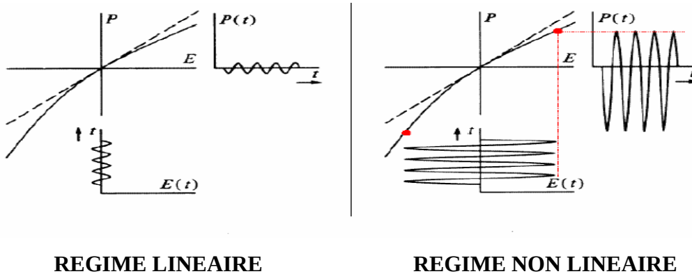
Figure 3.10 : Partie linéaire et non linéaire de la polarisation en fonction du champ électrique.
