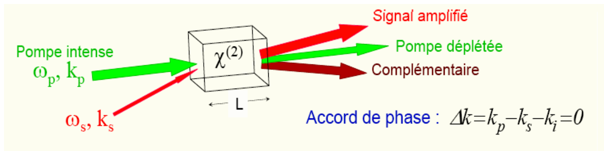
Figure 3.11 : Schéma de la différence de fréquence
