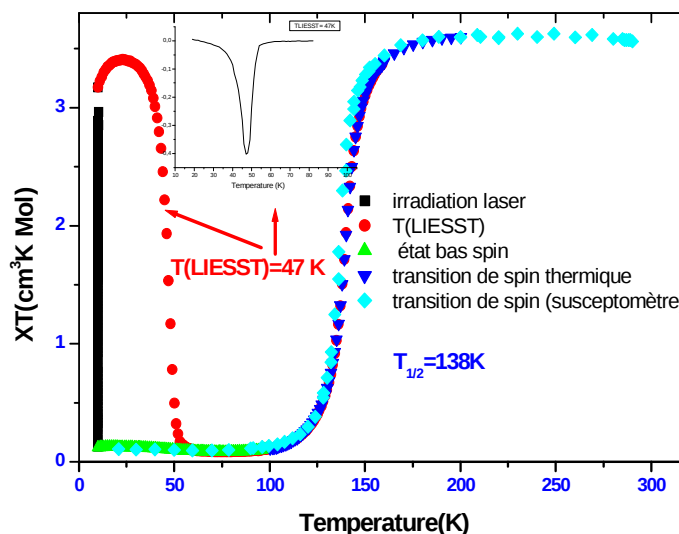
Figure 2.28 : Dispositif SQUID équipé d'un LASER et d'une fibre optique monté à l'ICMCB à Bordeaux (gauche). Détermination de la valeur du T(\text{LIESST}) dans le cadre du composé à transition de spin \text{FeDPEA}(\text{NCS})_2 (à droite). Sur la figure, cette température T(\text{LIESST}) ainsi que celle de la transition de phase thermique sont indiquées.
