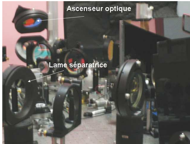
Figure 4.17 : Photo du dispositif optique mis en place en salle bordelaise.
