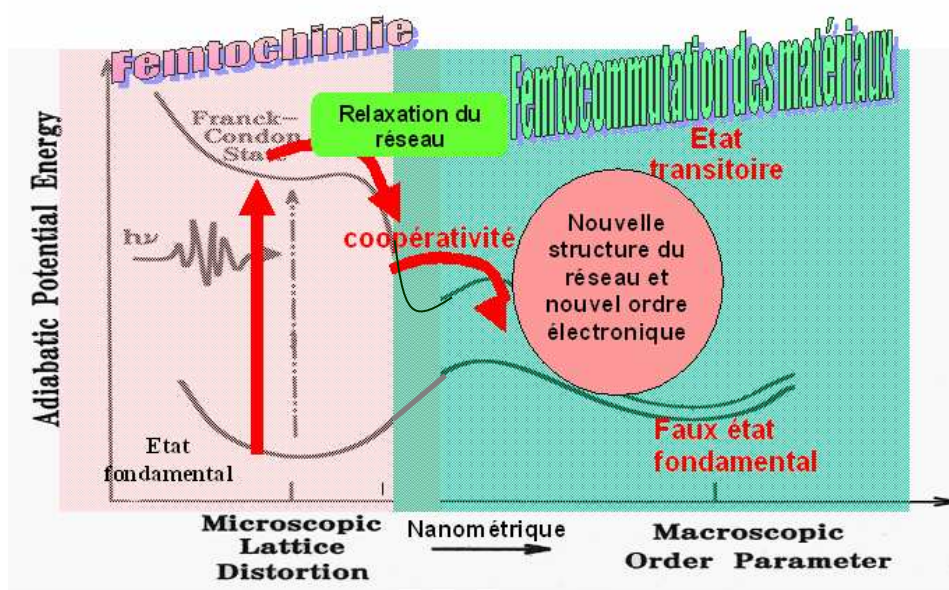
Figure 1.11 : Représentation schématisée d'une transformation de phase photo-induite (multi-stabilité et prolifération) (d'après Nasu (2004)).
