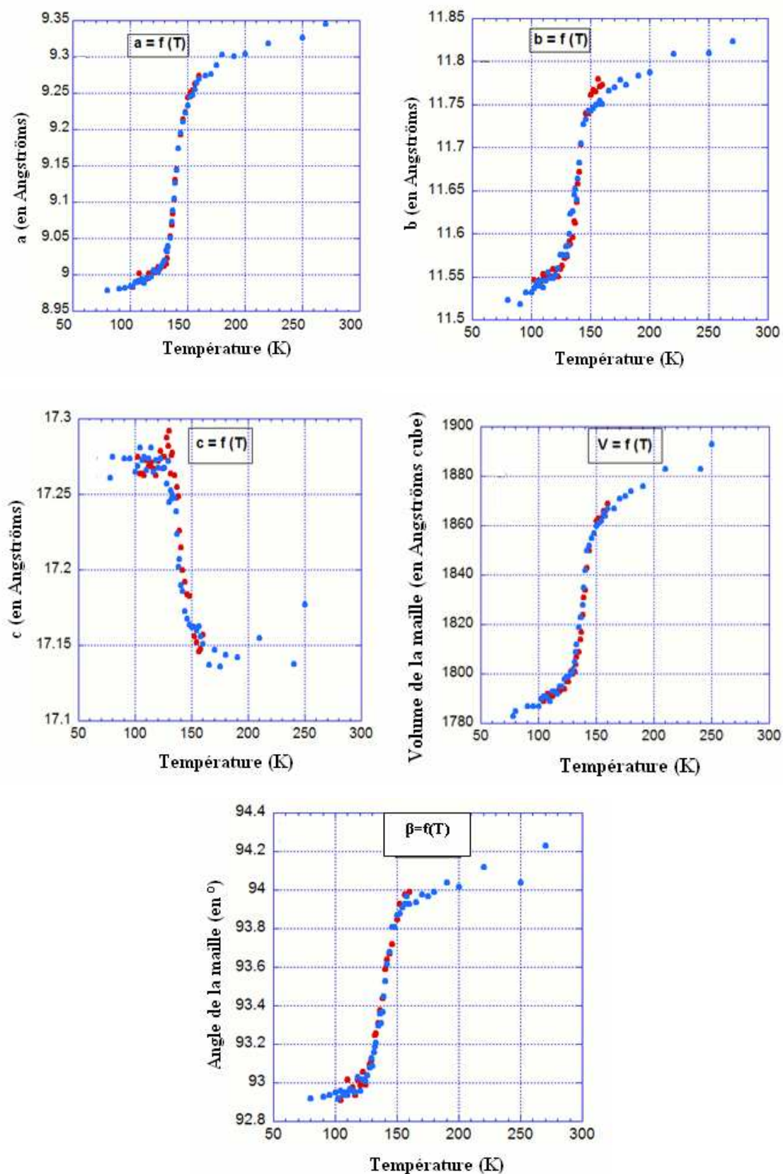
Figure 2.16 : Evolution en température des paramètres de maille du complexe \text{FeDPEA}(\text{NCS})_2 . Les points rouges correspondent à la phase de remontée en température alors que les points bleus sont caractéristiques de la descente en température.
