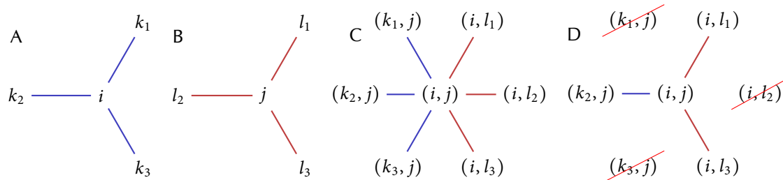
FIG. IV.1 : Topologie de l'hyper-réseau \mathbf{S} en fonction de celle des réseaux neutres \mathbf{A} et \mathbf{B} . A — Une séquence i de \mathbf{A} et ses connexions. B — Une séquence j de \mathbf{B} et ses connexions. C — Dans l'hyper-réseau \mathbf{S} le génotype (i,j) peut muter la séquence i ou la séquence j , mais pas les deux à la fois. Le nombre de connexions est donc la somme du nombre de liens de i dans \mathbf{A} et du nombre de liens de j dans \mathbf{B} . D — Après que les génotypes non viables ont été éliminés (ceux qui sont barrés dans le schéma B), on obtient l'hyper-réseau neutre s . La robustesse du génotype (i,j) vaut trois dans l'exemple présenté.
