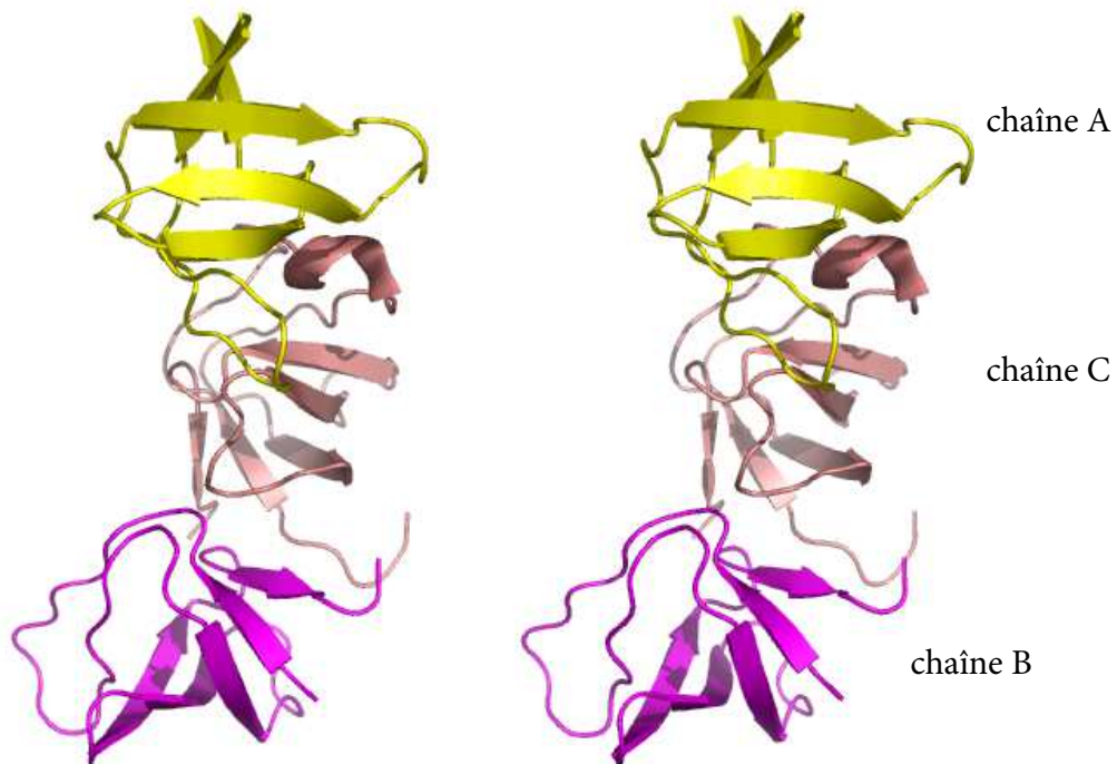
FIG. II.12 : Vue stéréoscopique de IGCQ. Les chaînes B et C sont les domaines SH3 de Grb2 de Vav que nous allons étudier.
