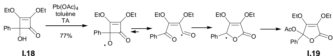
Schéma 1.8 : Synthèse de furanones par oxydation de 4-hydroxycyclobuténones.
