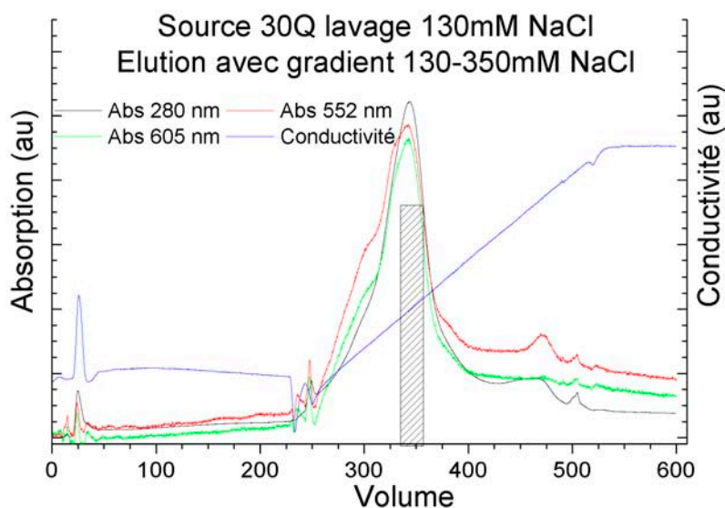
Figure 4.5 : Chromatogramme de l'élué de l'oxydase aa_3 sur la résine Source 30Q. la zone hachurée correspond aux fractions sélectionnées.
