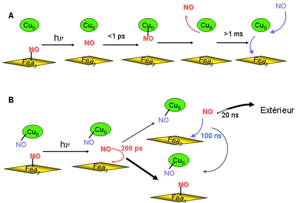
Figure 4.21 : Modèles décrivant la dynamique du NO après photodissociation lorsque 1 NO (A) et 2 NO (B) sont présents dans le site actif.
