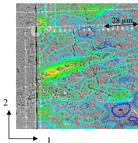
Figure 13 : Isovaleurs de la composante de la déformation E22 (dans le sens de sollicitation) concentrées autour d'un hydrure radial, révélé par attaque chimique (pas de la grille 4 μm).
