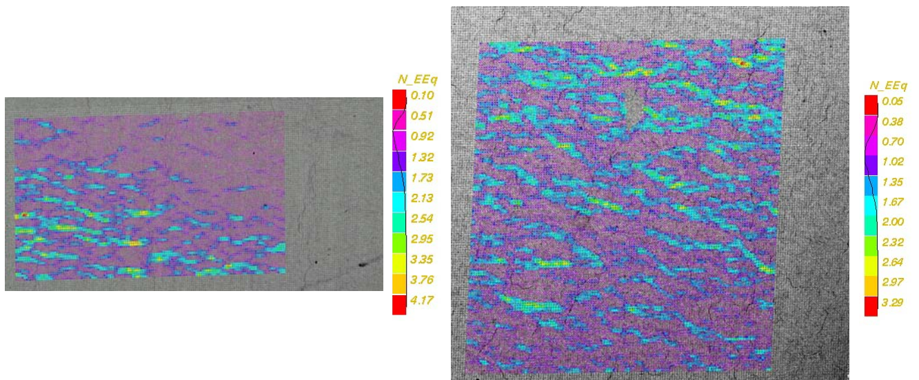
Figure 16 : Cartes de déformation des différentes configurations dans l'une des zones les plus déformées de ces éprouvettes. Comparaison de la répartition des bandes. Pour une meilleure visibilité, certaines cartes sont représentées dans la configuration de référence. Les images de la microstructure ont été acquises avec les électrons rétrodiffusés.
