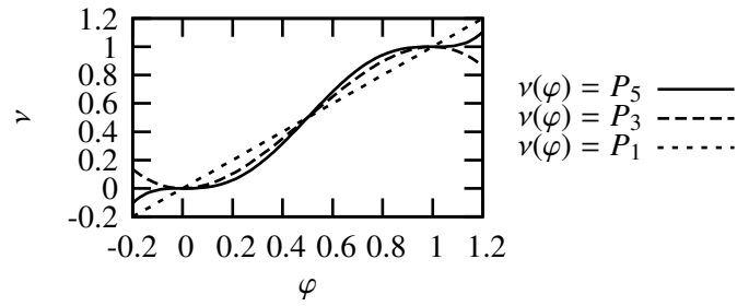
Figure C.6: Fonction d'interpolation
