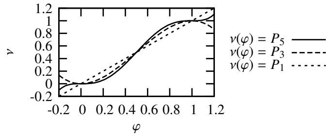
Figure C.6: Fonction d'interpolation
