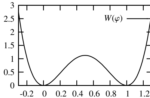
Figure C.5: Fonction double-puits
