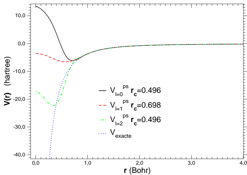
FIG. 1.2 – Comparaison du pseudopotential avec le potentiel exact avant désécrantage. Rayon de coupure en Bohr.
