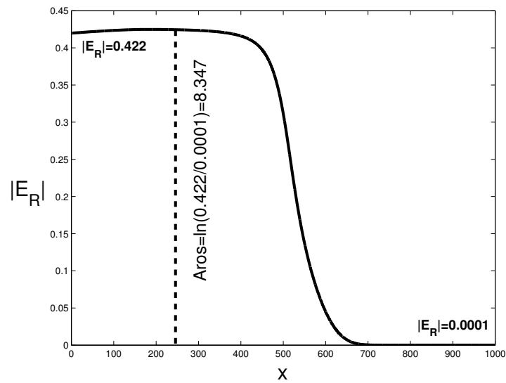
FIG. A.4.: Amplification spatiale de Rosenbluth : onde rétrodiffusée en fonction de l'espace, à t = 30000\omega_0^{-1} , pour la résonance sélectionnée au centre du plasma
