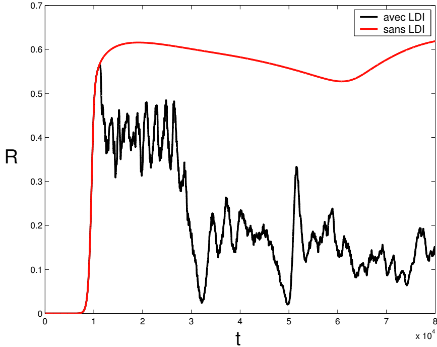
FIG. 6.18.: réflectivités en fonction du temps pour T = [0 : 80000]\omega_0^{-1} avec et sans couplage au LDI
