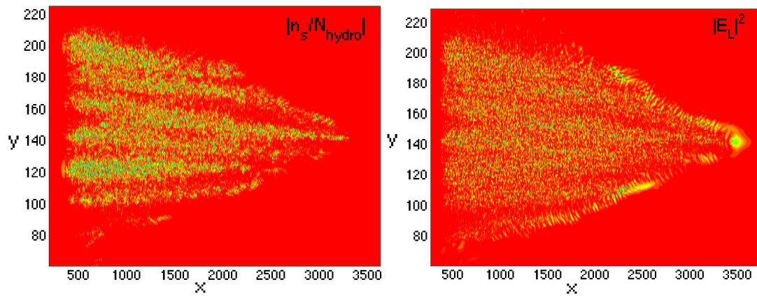
FIG. 6.36.: SRS couplée aux ondes sonores : onde sonore avec |\frac{n_s}{N_{hydro}}|_{moy} = 0.7 (G) et onde de Langmuir avec |E_L|_{moy}^2 = 35 (D) sur L_x = [61 : 915] \frac{c}{\omega_0} ( L_x = [250 : 3750] sur le maillage), L_y = [130 : 450] \frac{c}{\omega_0} ( L_y = [65 : 225] sur le maillage) à t = 17500\omega_0^{-1}
