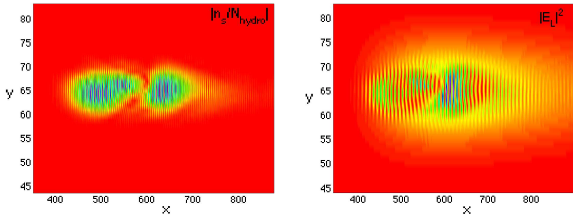
FIG. 6.19.: SRS couplée aux ondes sonores : onde sonore avec \left| \frac{n_s}{N_{hydro}} \right|_{moy} = 0.095 (G) et onde de Langmuir avec |E_L|_{moy}^2 = 3 (D) sur L_x = [85 : 214] \frac{c}{\omega_0} ( L_x = [350 : 875] sur le maillage), L_y = [86 : 166] \frac{c}{\omega_0} ( L_y = [43 : 83] sur le maillage) à t = 11500\omega_0^{-1}
