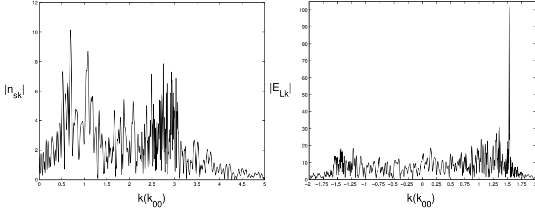
FIG. 4.43.: cascade LDI : spectre de Fourier de l'onde sonore (G) et de l'onde de Langmuir (D) à t = 32000\omega_0^{-1}
