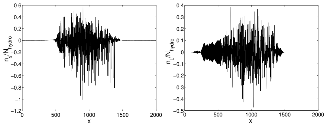
FIG. C.5.: SRS couplée aux ondes sonores pour G_{Ros} < 6 : onde sonore (G) et onde de Langmuir (D) en fonction de l'espace pour t = 100000\omega_0^{-1}
