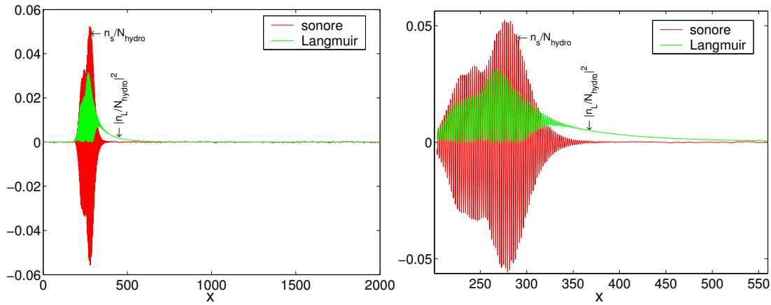
FIG. 4.37.: SRS couplée aux ondes sonores : ondes sonore et de Langmuir dans tout le plasma (G) puis zoom sur L = [210 : 555] \frac{c}{\omega_0} (D) à t = 19000 \omega_0^{-1}
