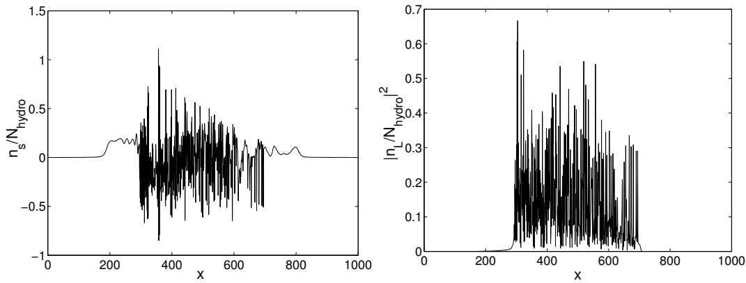
FIG. 5.15.: SRS couplée aux ondes sonores pour 3.5 \leq G_{Ros} \leq 7 : onde sonore (G) et onde de Langmuir (D) en fonction de l'espace à t = 100000\omega_0^{-1}
