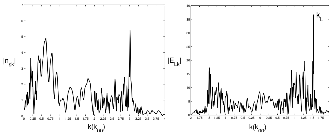
FIG. 4.20.: cascade LDI : spectre de Fourier de l'onde sonore (G) et de l'onde de Langmuir (D) à t = 50000\omega_0^{-1}
