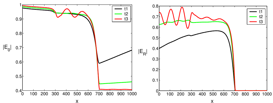
FIG. 5.3.: SRS sans couplage avec les ondes sonores pour 3.5 \leq G_{Ros} \leq 7 : ondes incidentes (G) et rétrodiffusées (D) en fonction de l'espace pour t_1 = 7500\omega_0^{-1} , t_2 = 8500\omega_0^{-1} et t_3 = 10000\omega_0^{-1}
