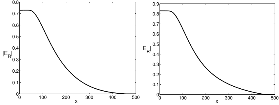
FIG. 4.8.: SRS sans couplage avec les ondes sonores : onde rétrodiffusée en fonction de l'espace à t = 35000\omega_0^{-1} (G) et t = 80000\omega_0^{-1} (D)
