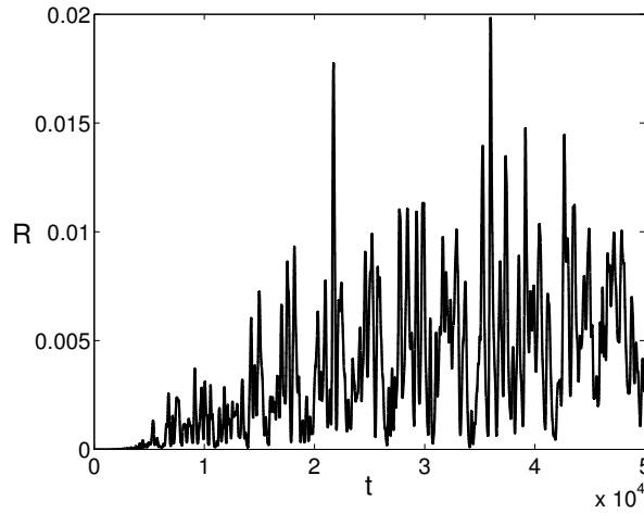
FIG. 6.42.: SRS sans couplage avec les ondes sonores pour 3.5 \leq G_{Ros} \leq 10 : réflectivité en fonction du temps
