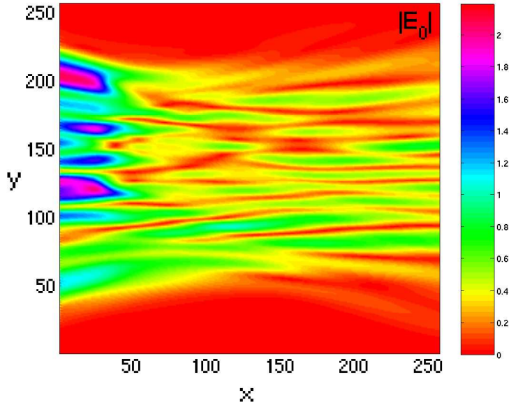
FIG. 6.27.: SRS sans couplage avec les ondes sonores : onde incidente dans tout le plasma à t = 17500\omega_0^{-1}
