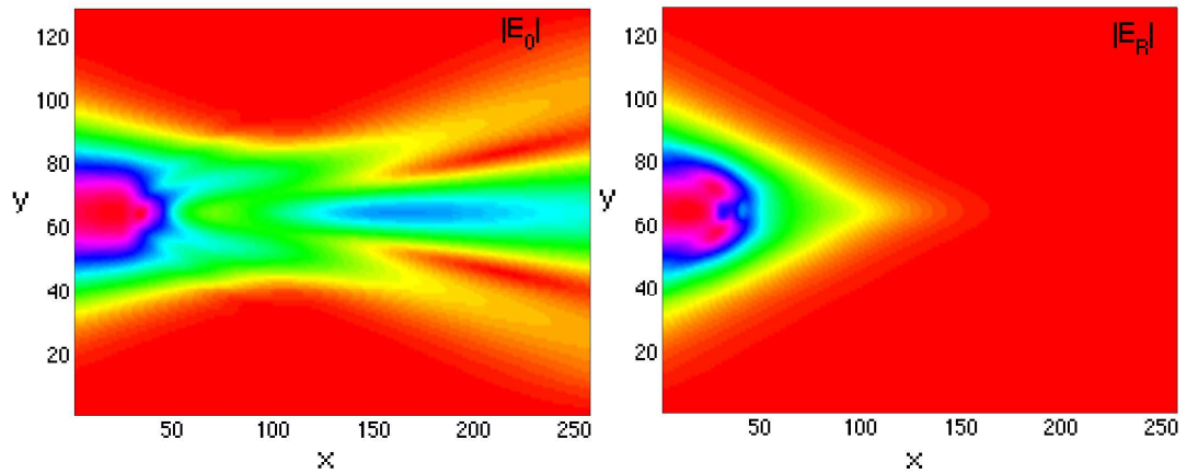
FIG. 6.20.: SRS couplée aux ondes sonores : onde incidente (G) et onde rétrodiffusée avec |E_R|_{max} = 0.6 (D) dans tout le plasma à t = 11500\omega_0^{-1}
