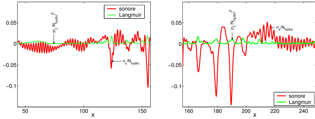
FIG. 4.22.: zoom sur [45, 155] \frac{c}{\omega_0} (G) puis sur [156, 250] \frac{c}{\omega_0} (D) de l'onde sonore et de Langmuir à t = 80000\omega_0^{-1}
