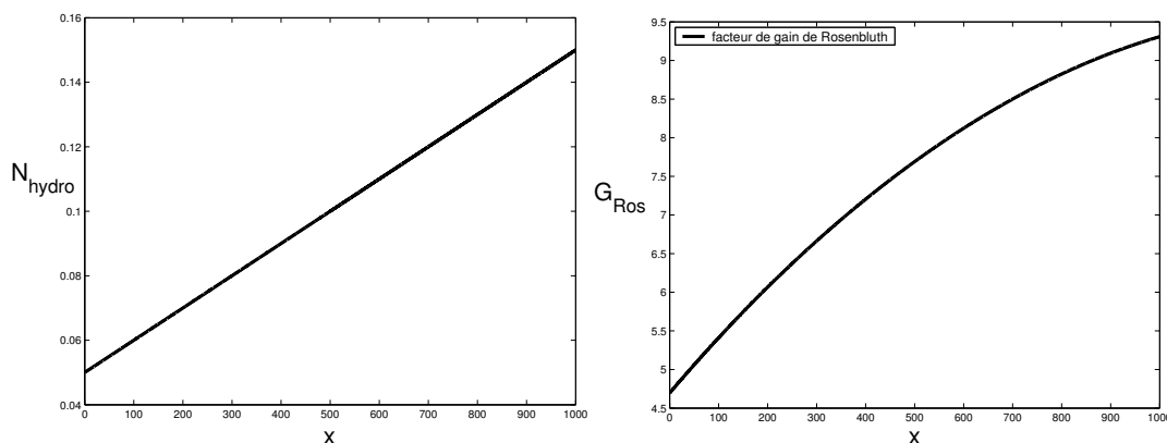
FIG. 3.1.: profil de densité (G) et facteur de gain de Rosenbluth (D) en fonction de l'espace
