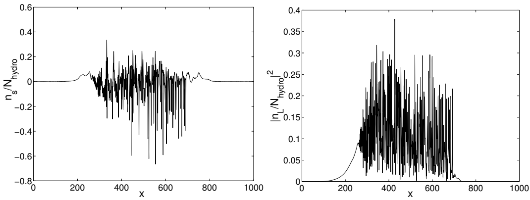
FIG. 5.24.: SRS couplée aux ondes sonores pour 1 \leq G_{Ros} \leq 3.5 : onde sonore et onde de Langmuir à t = 100000\omega_0^{-1}
