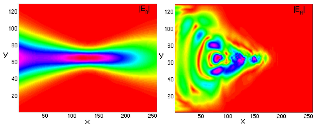
FIG. 6.51.: SRS couplée aux ondes sonores pour 3.5 \leq G_{Ros} \leq 10 : onde incidente (G) et onde rétrodiffusée avec |E_R|_{max} = 0.09 (D) dans tout le plasma à t = 7500\omega_0^{-1}
