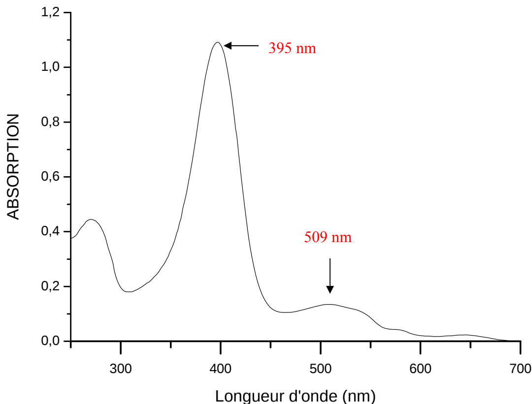
Figure 2.4: Spectre d'absorption de FixLH après purification et élimination de l'imidazole. Les maxima d'absorption correspondent à la bande Soret (395 nm) spécifique d'un hème pentacoordonné à l'état oxydé \text{Fe}^{3+} et à la bande \alpha (509 nm).
