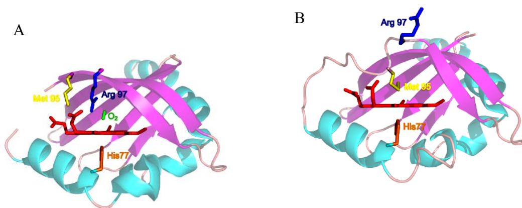
Figure 1.14 : Structure de la poche de l'hème de DosH. L'oxycomplexe est représenté sur la figure (A) avec la présence d'O 2 (en vert) et l'état déoxy est représenté sur la figure (B). Les résidus importants sont identifiés sur la structure, en particulier H77, M95 et R97). On constate la grande différence de la position de Met95 et Arg97 dans les deux structures (d'après Park et coll. , 2004).
