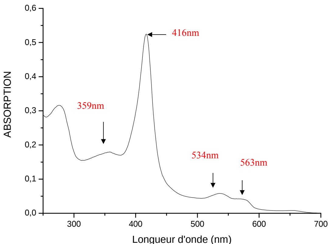
Figure 2.20: Spectre d'absorption de DosH après purification et élimination de l'imidazole. Le maximum d'absorption correspond à la bande Soret (416 nm) spécifique d'un hème b \text{Fe}^{3+} hexacoordonné et les bandes \alpha sont situées à 534 nm et 563 nm. La bande à 359 nm correspond à la bande \delta de l'hème.
