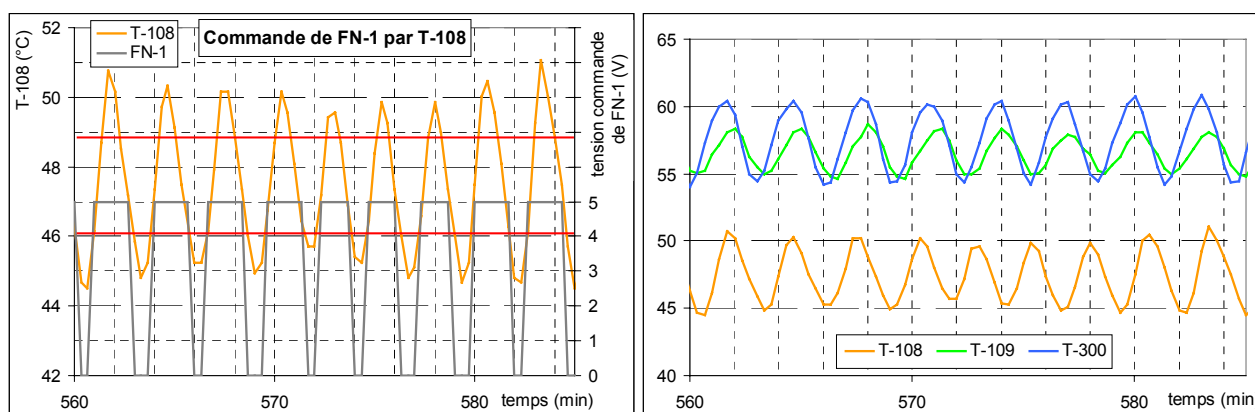
figure II. 23 : commande du ventilateur FAN-1 (g.) et températures du reformat en différents points (dr.)
