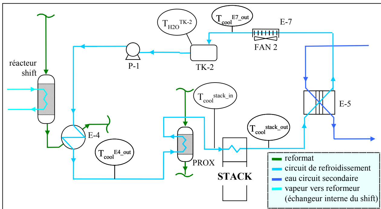
figure II. 20 : schéma du circuit de refroidissement interne du RCU-4500
