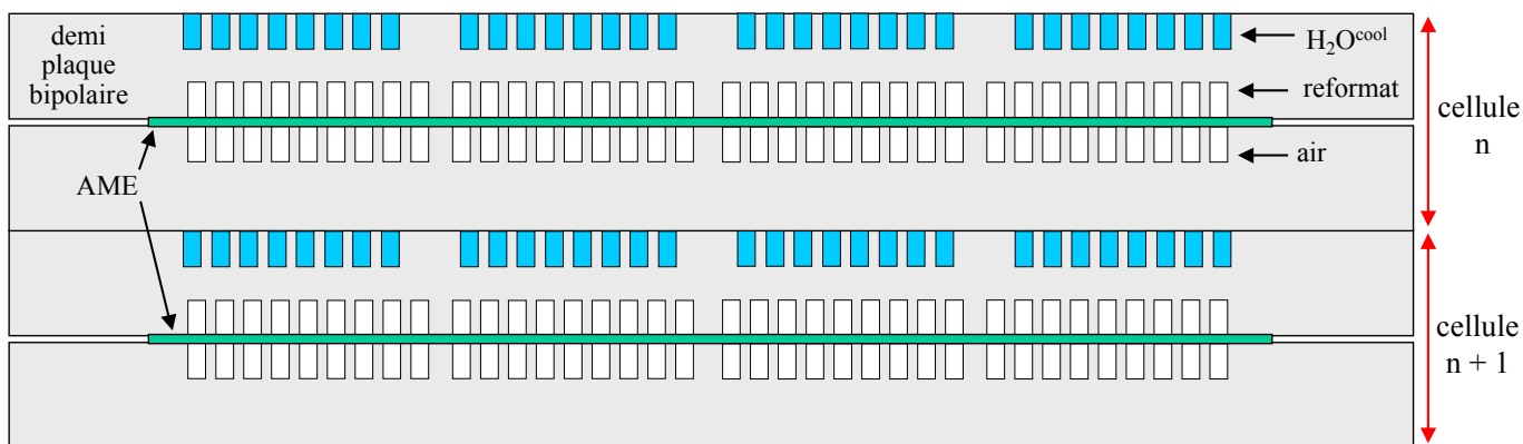
figure II. 7 : coupe de deux cellules consécutives, dans le plan perpendiculaire aux canaux de distribution
