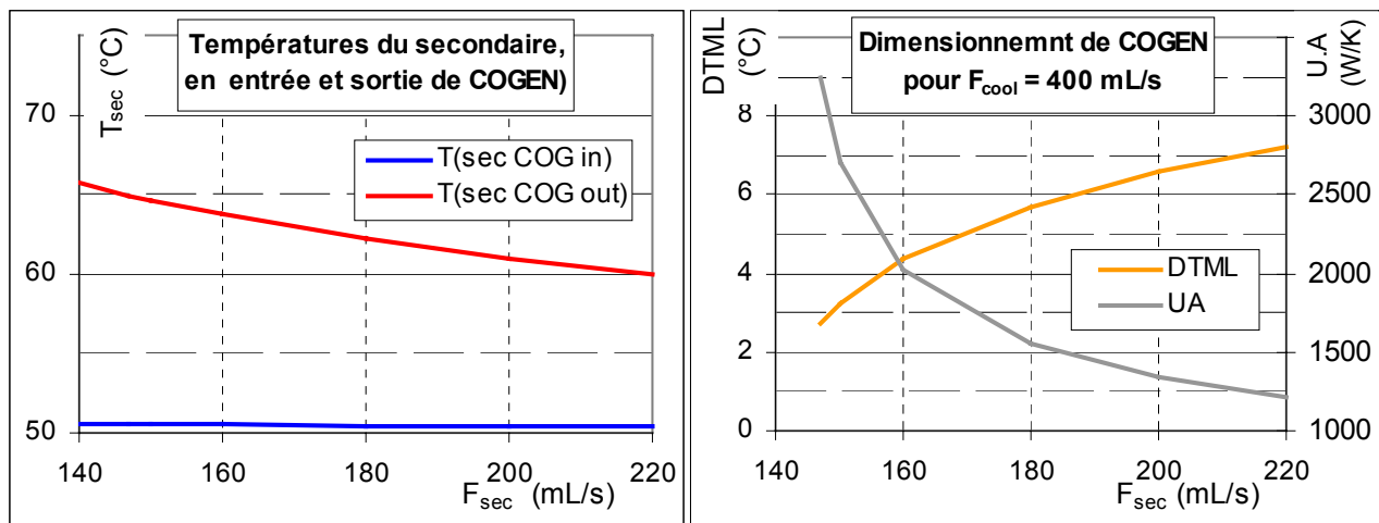
figure IV. 10 : températures du secondaire en entrée-sortie de COGEN (g.) et dimensionnement de cet échangeur (dr.) en fonction de F_{sec} , pour F_{cool} = 400 mL/s
