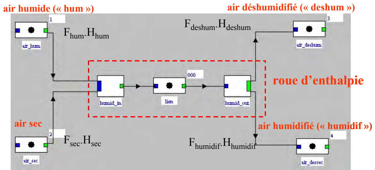
Figure 3 : schéma du composant et de son environnement sous Thermoptim
