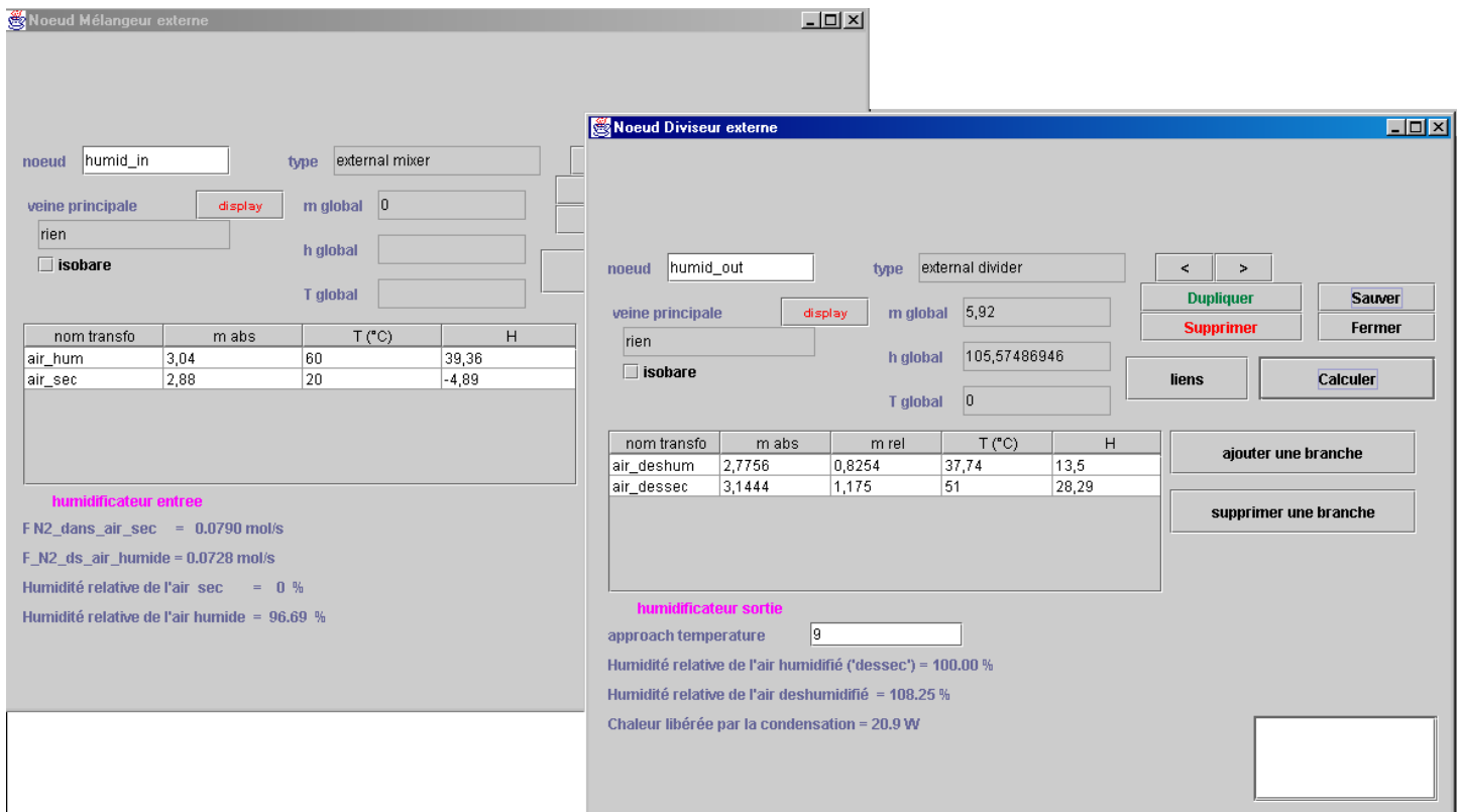
Figure 4 : aspect des écrans des deux nœuds externes "humid_in" et "humid_out"
