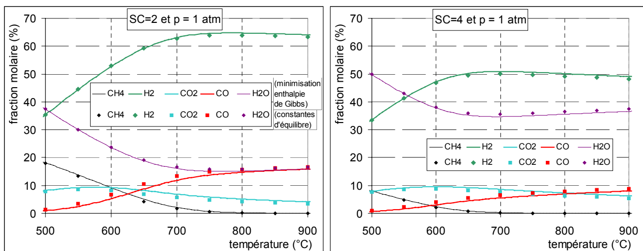
figure I. 12 : composition calculée du reformat primaire pour les deux méthodes (en traits continus : méthode de minimisation de l'enthalpie de Gibbs ; en carrés : méthode des constantes d'équilibre)
