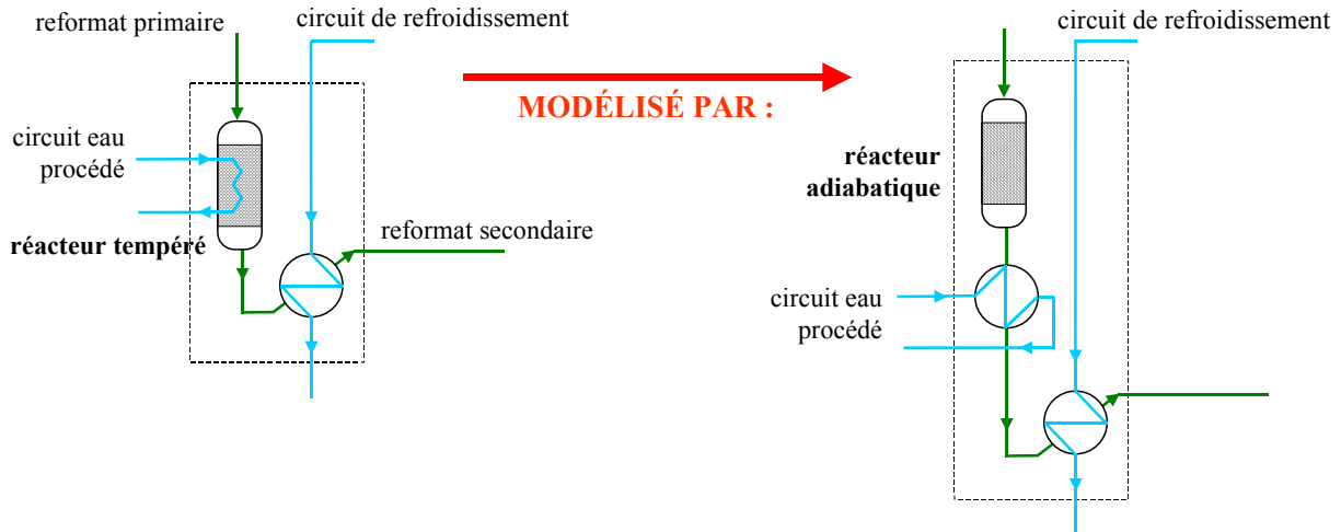
Figure 1 : modélisation du réacteur shift par un réacteur adiabatique
