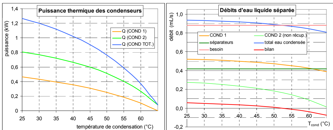
figure IV. 11 : puissance thermique récupérée aux condenseurs (g.) et eau condensée en fonction de la température de condensation (dr.)
