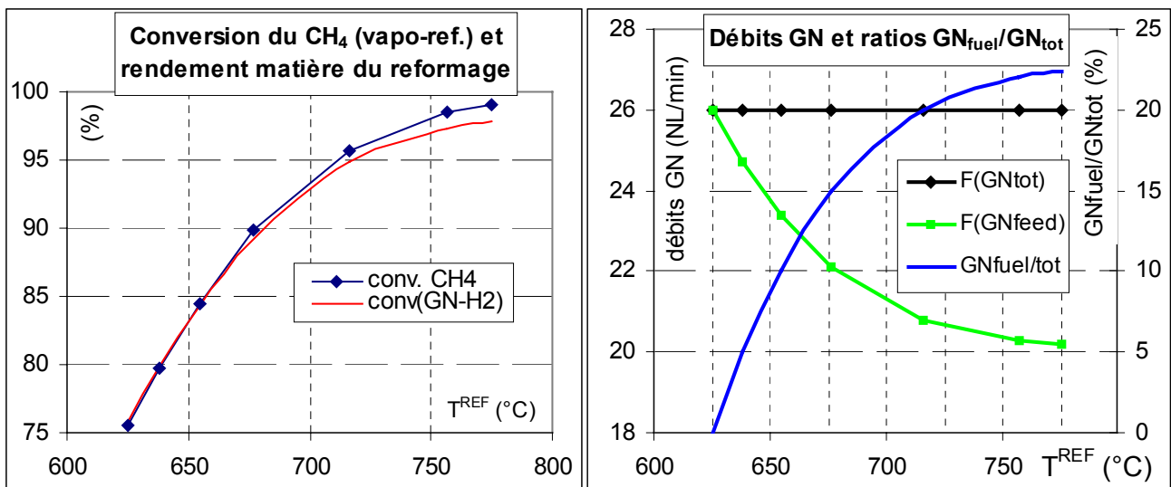
figure IV. 2 : influence de la température du vapo-reformeur ( T^{\text{REF}} ) sur le taux de conversion du CH_4 (g.) et le débit de GNfeed (dr.)
