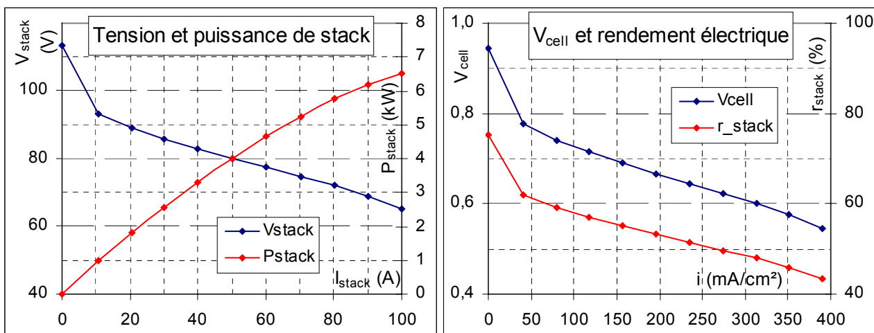
figure II. 14 : exemple de courbe de polarisation de stack et de cellule
