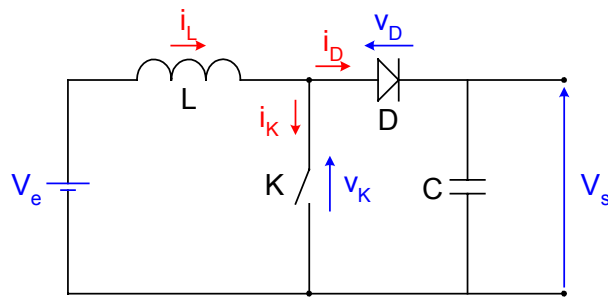
Figure 2 : schéma de principe du hacheur élévateur
