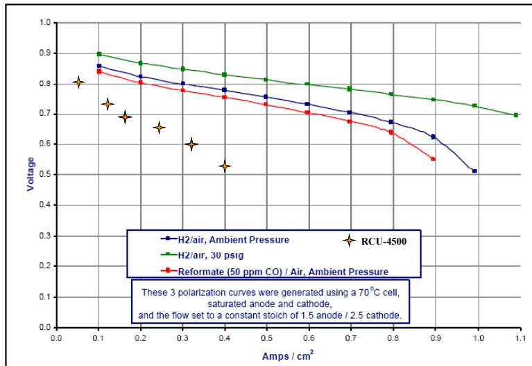
figure IV. 13 : courbe UI d'un AME de 3M [3M_MEA], A = 100 cm 2
