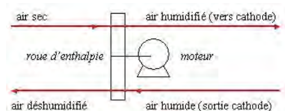
Fig. 2 : schéma élément dans le plan H Power
