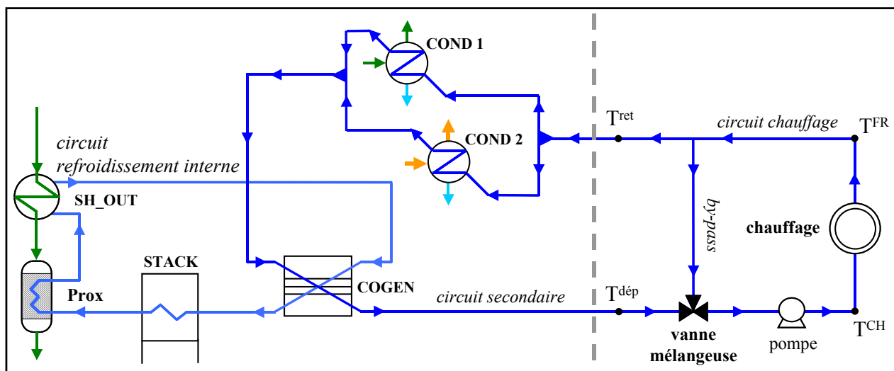
figure IV. 5 : schéma de la valorisation de la chaleur (emplacement des condenseurs : figure IV. 1)
