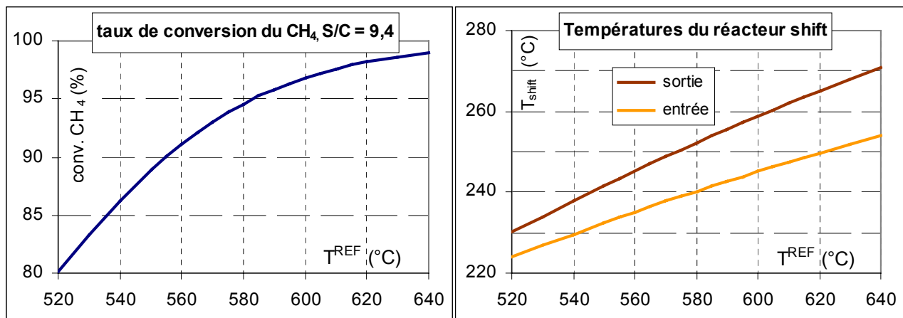
figure IV. 20 : influence de la température du vapo-reformeur sur le taux de conversion du méthane (g.) et sur les températures du réacteur shift (dr.)
