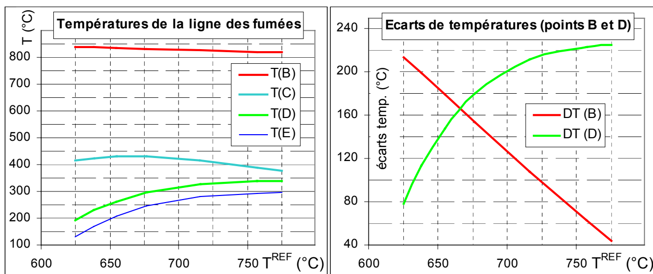
figure IV. 4 : températures de la ligne des fumées (g.) et écarts de température minimaux (dr.)
