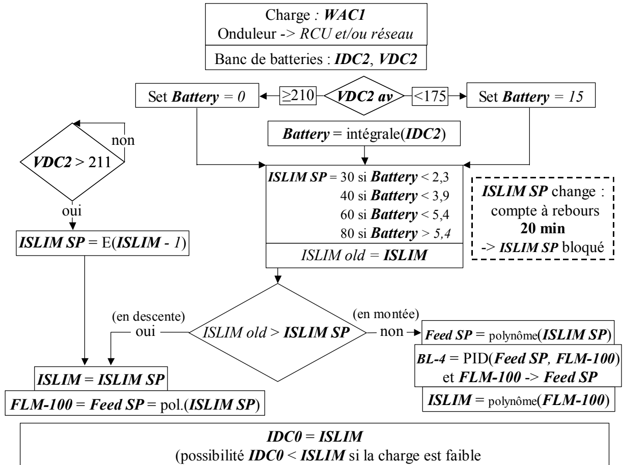
Figure 1 : diagramme du processus d'obtention de l'intensité délivrée par le stack
