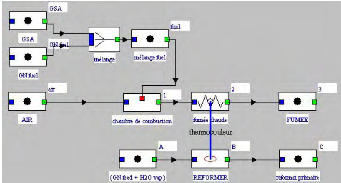
Figure 2 : La chambre de réaction (REFORMER), la chambre de combustion et le thermocoupleur (échangeurs de préchauffe et bouilloire non représentés).
