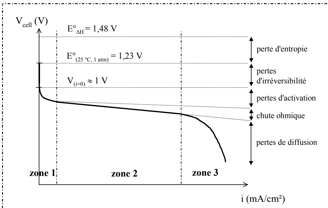
figure I. 10 : courbe de polarisation type pour une cellule alimentée en \text{H}_2/\text{air}
