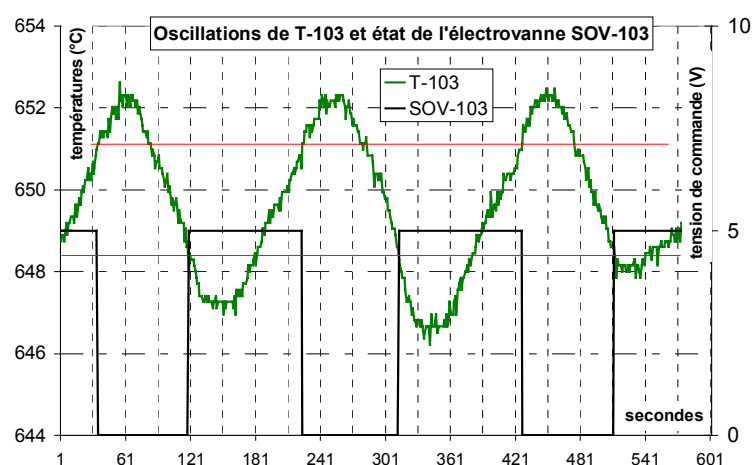
Figure 3 : commande de SOV-103 par la température du vapo-reformeur
