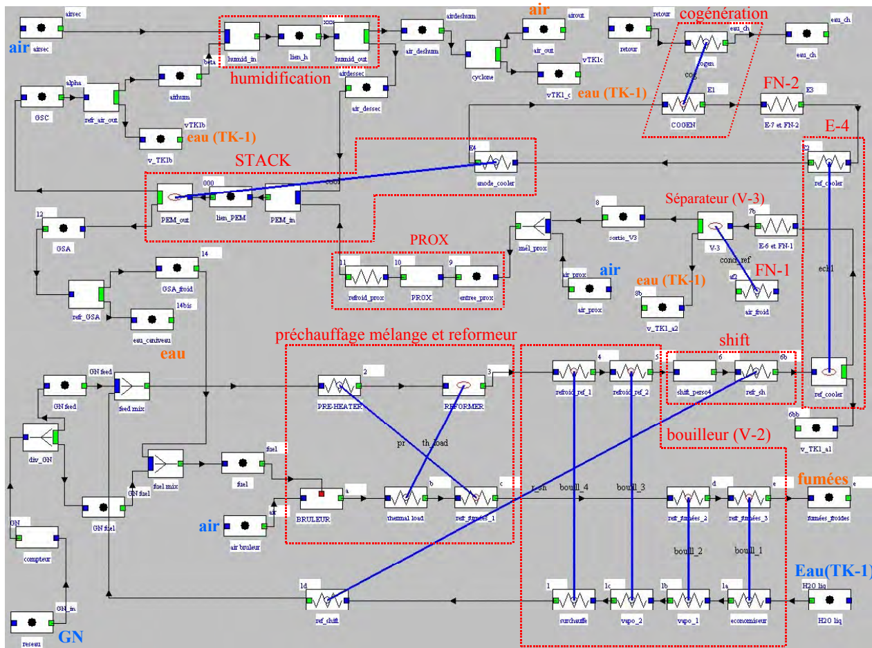
figure II. 19 : schéma du procédé sous Thermoptim
