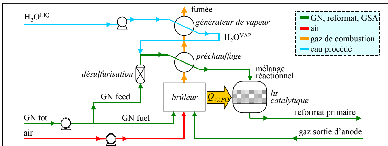
figure I. 5 : exemple de schéma du bloc reformeur
