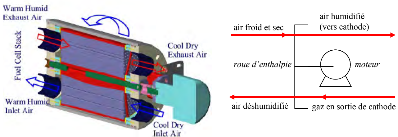
figure II. 9 : schéma de la documentation du fabricant (g.) et schéma de l'élément sur le plan H Power
