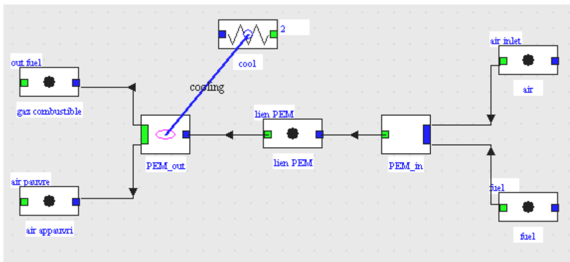
Figure 1 : schéma du composant PEMFC sous Thermoptim, avec ses quatre entrées-sorties
