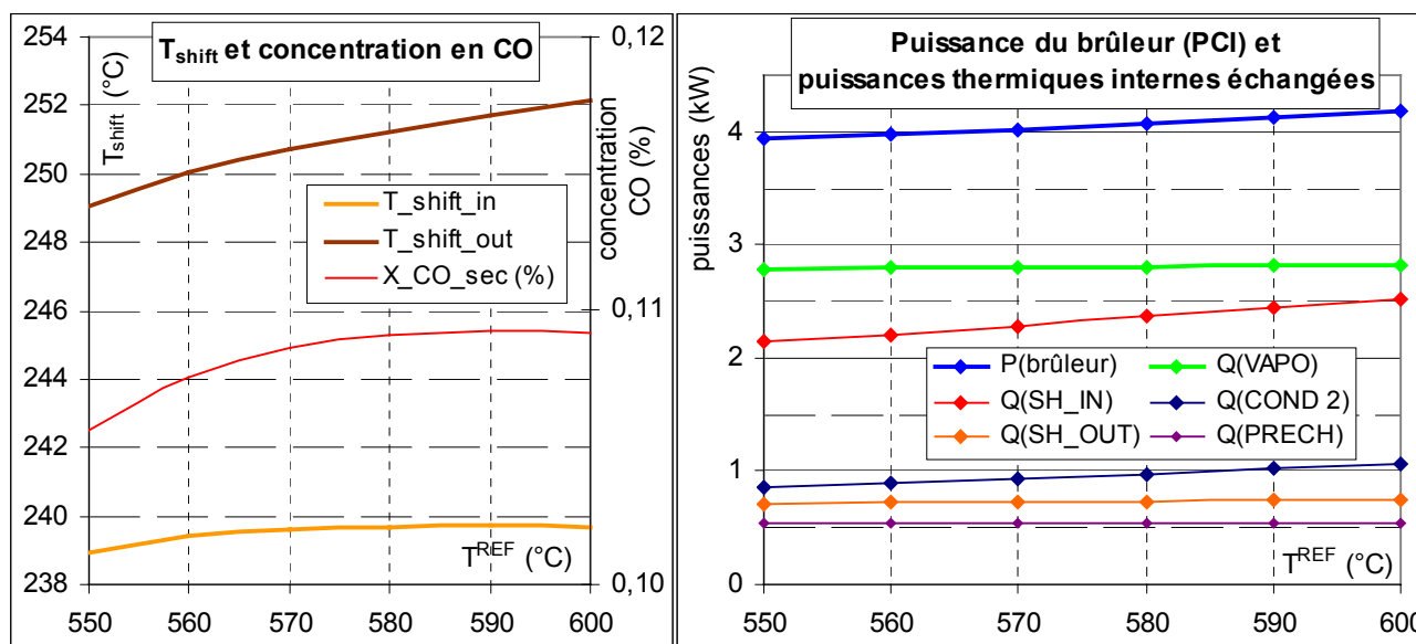
figure IV. 22 : températures d'entrée et sortie du shift (g.) et puissances échangées dans le procédé (dr.)
