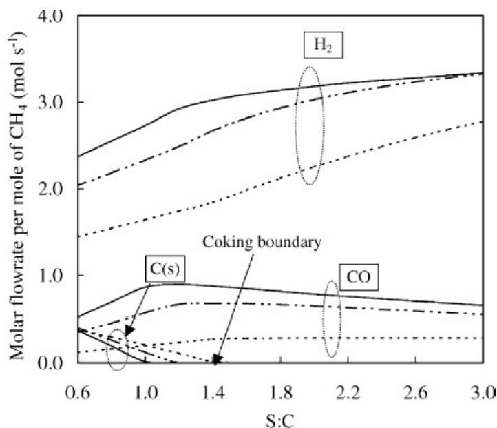
figure I. 11: effet du ratio S/C sur l'équilibre thermodynamique dans un réacteur de vapo-reformage à 1 bar et à 600 °C (---), 700 °C (—) et 800 °C (trait continu).
