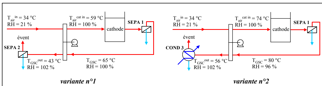
figure IV. 14 : températures et humidités relatives en entrée et sortie de la roue d'enthalpie pour les deux variantes
