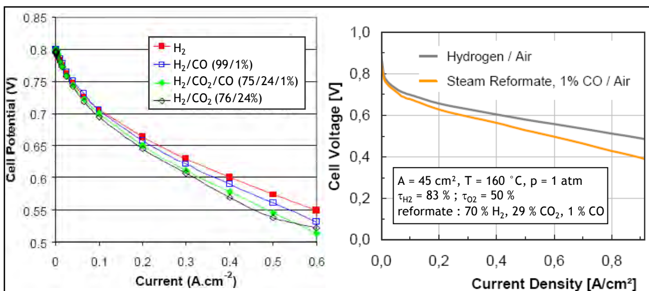
figure IV. 17 : exemples de courbes de polarisation de cellules avec une membrane de type PBI
