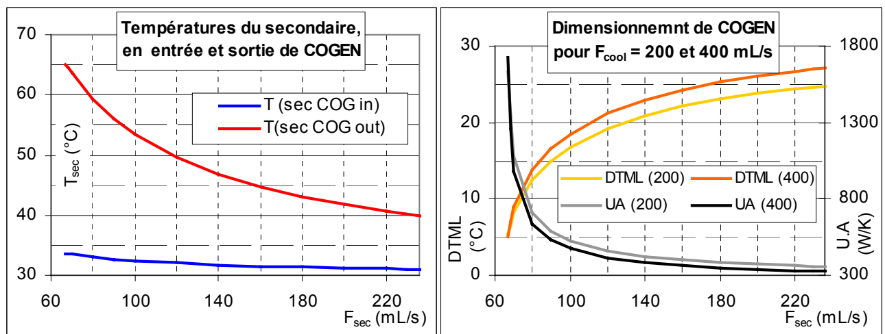
figure IV. 7 : températures du secondaire en entrée-sortie de COGEN (g.) et dimensionnement de cet échangeur (dr.) en fonction de F_{sec} pour deux valeurs de F_{cool}
