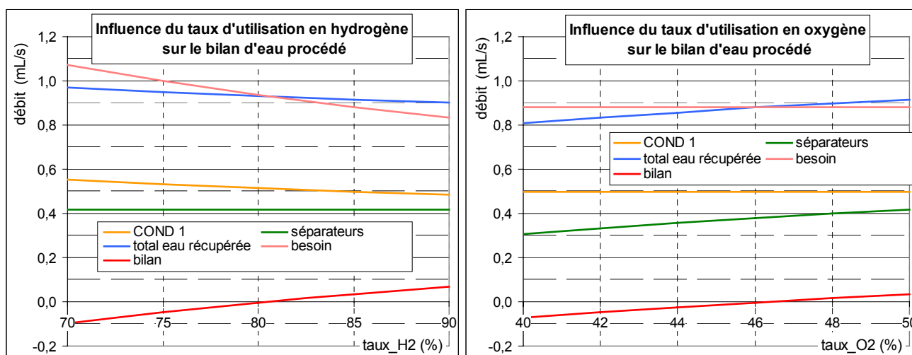
figure IV. 12 : influence du taux d'utilisation en hydrogène sur le bilan d'eau procédé
