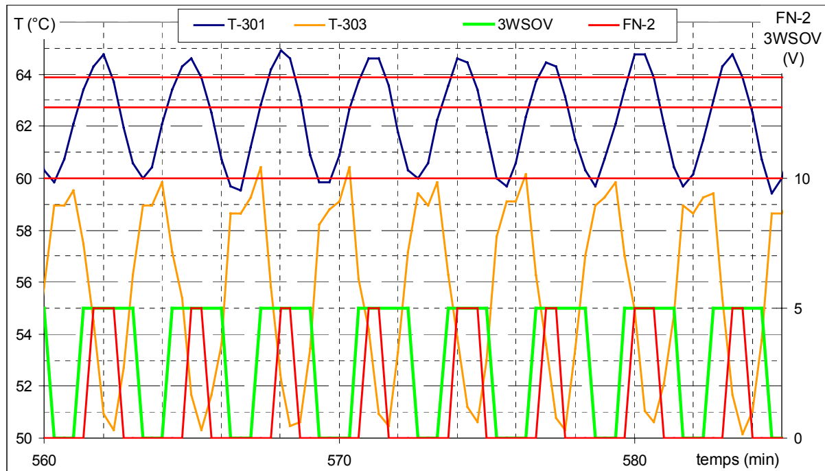
Figure 6 : commande de T-301 sur FAN-2 et 3WSOV et effet sur la température en aval (unité de Sophia Antipolis, pleine charge)
