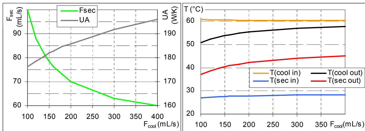
figure IV. 8 : F_{\text{sec}} et UA en fonction de F_{\text{cool}} (g.) et 4 températures de l'échangeur COGEN (dr.)
