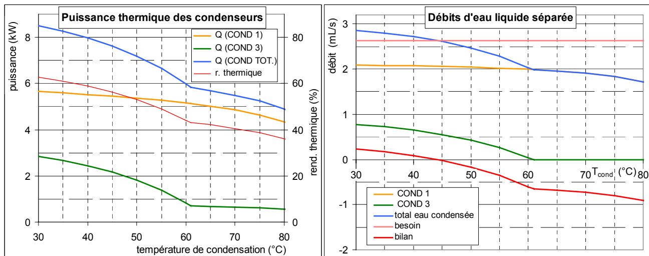
figure IV. 24 : valorisation thermique et bilan d'eau en fonction de la température de condensation
