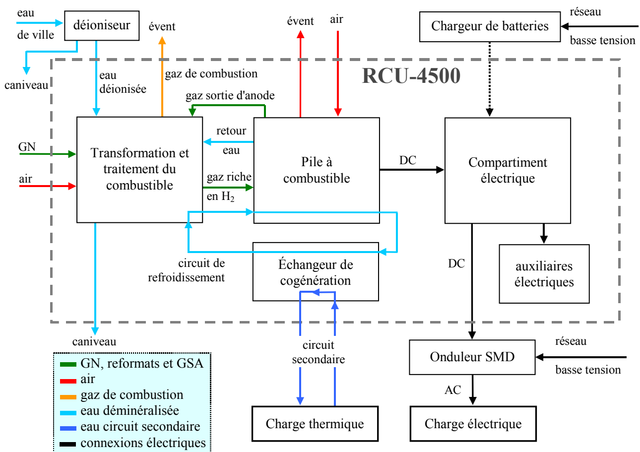
figure II. 1 : schéma de principe du RCU-4500, des auxiliaires externes, des raccordements électriques et thermiques
