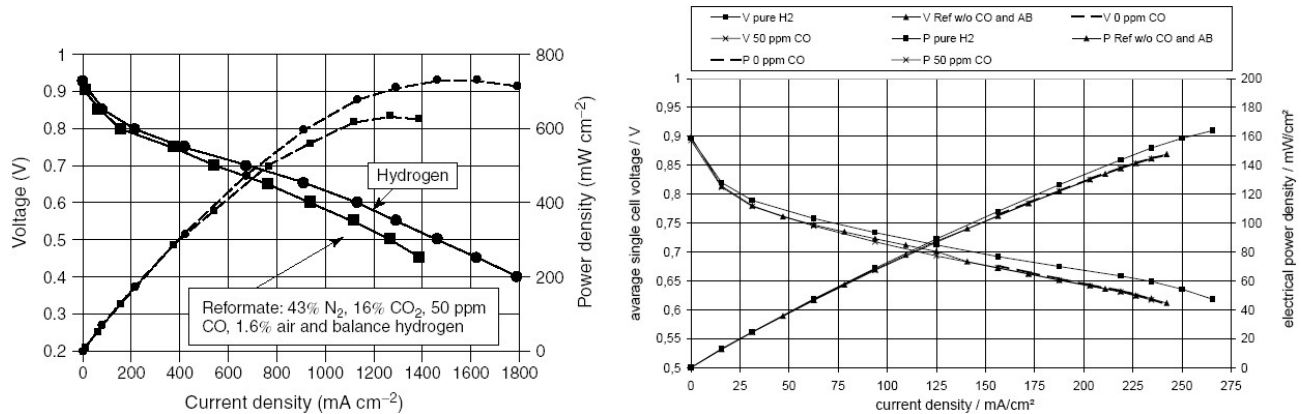
figure I. 9: courbe caractéristique d'un AME (g.) et d'un stack (dr.) dans des conditions proches
