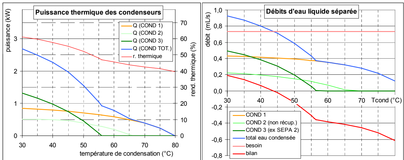
figure IV. 15 : puissances échangées aux condenseurs (g.) et bilan d'eau (dr.) en fonction de la température de condensation
