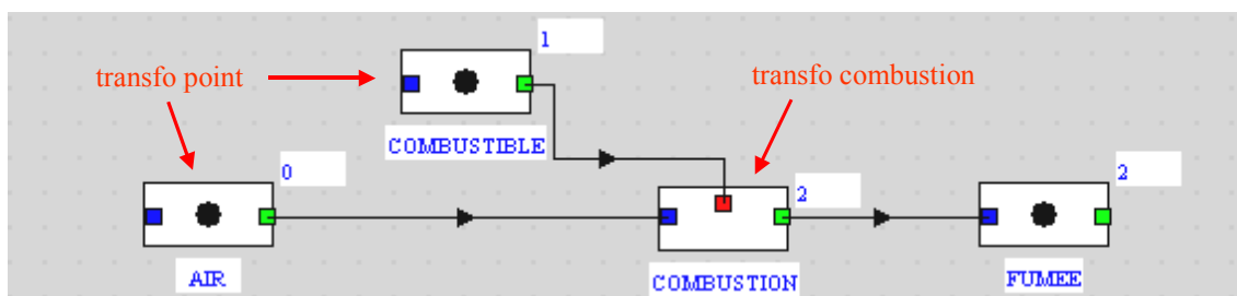
figure II. 16 : exemple de transfo combustion et de transfos point dans l'éditeur de schéma
