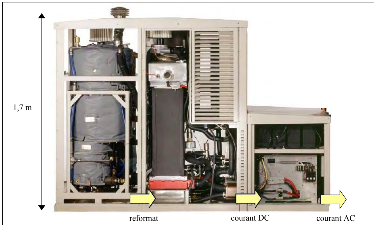
figure I. 1 : vue ouverte du GenSys 1 , avec de gauche à droite, la partie reformage, la pile à combustible et ses auxiliaires, le compartiment électrique
