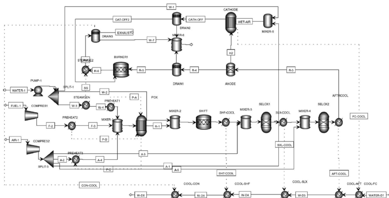
figure I. 14 : schéma de procédé du travail de W. Colella
