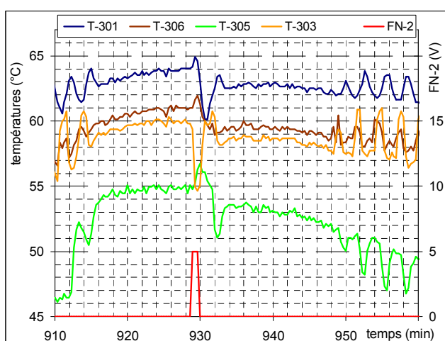
figure II. 25 : stabilisation partielles des températures
