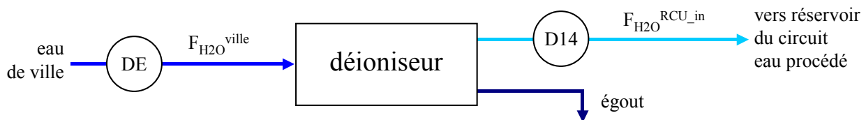
figure II. 15 : schéma de principe du raccordement du déioniseur avec le circuit d'eau de ville et le RCU
