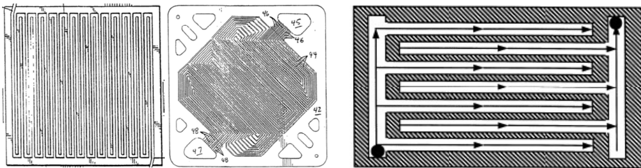
figure I. 7 : exemples de canaux en serpentins (g., version ancienne et récente) et de canaux intercalés (dr.)
