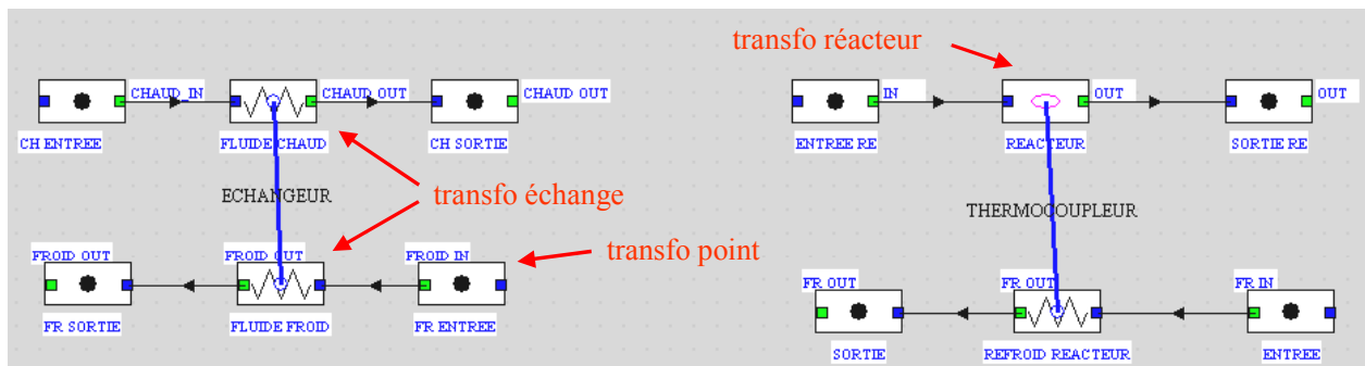
figure II. 17 : représentation d'un échangeur et d'un thermocoupleur dans l'éditeur de schéma
