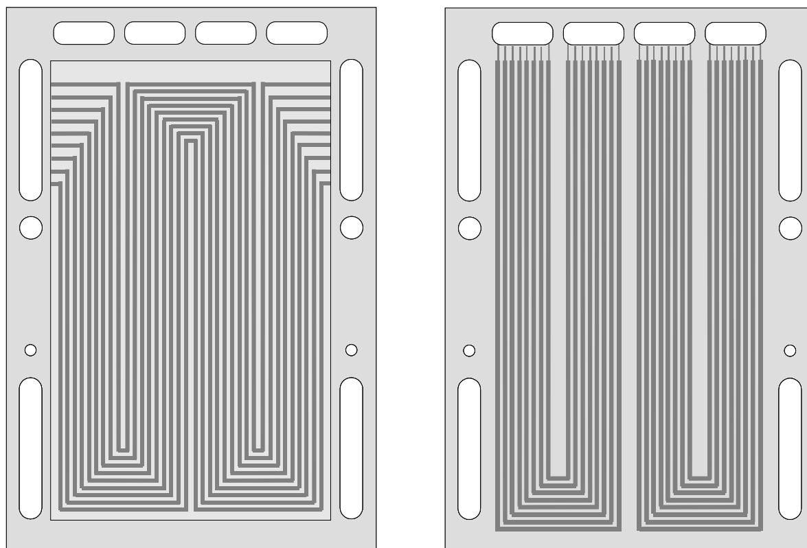
figure II. 8: demi plaque bipolaire avec les canaux de distribution du reformat (g.) et du circuit de l'eau de refroidissement (dr.)
