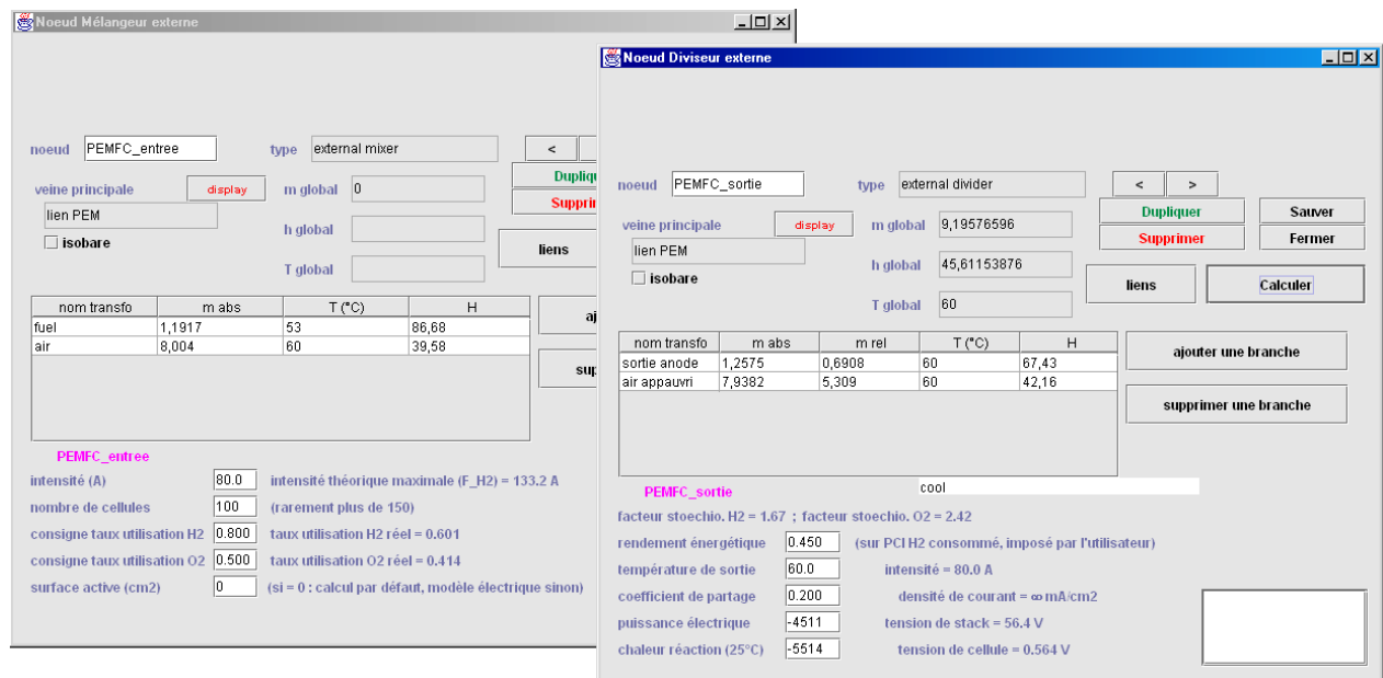
Figure 2 : aspect des écrans des classes PEMFCentree et PEMFCsortie pour la première utilisation
