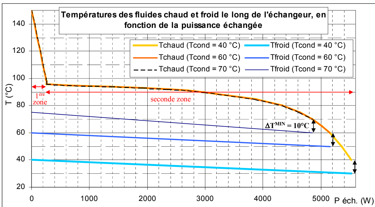
figure IV. 23 : courbe flux d'enthalpie vs. température du condenseur COND 1
