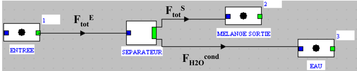
Figure 1 : schéma du composant avec les notations de débits molaires
