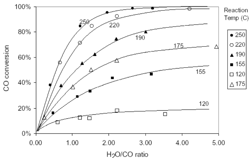
figure I. 13: taux de conversion du CO en fonction de la température et du ratio H_2O/CO du mélange entrant, à 1 atm et GHSV = 6100 h^{-1} .
