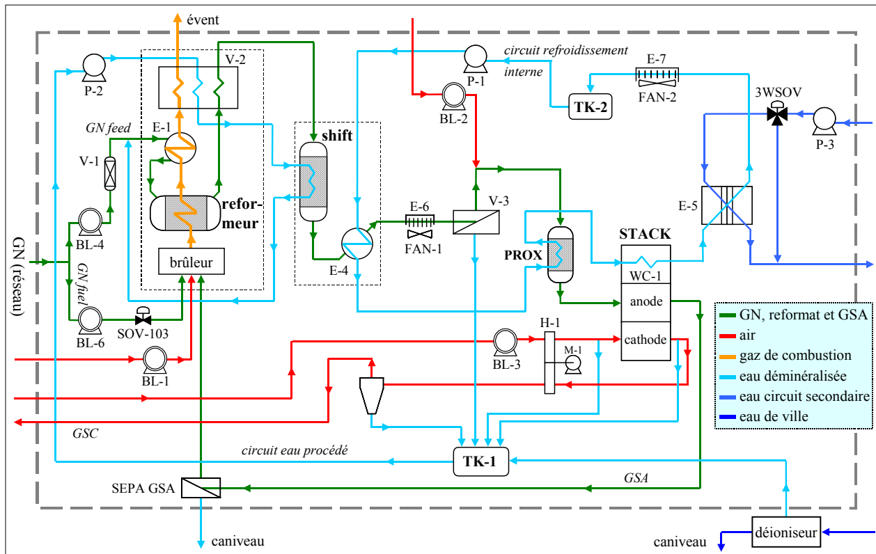
figure II. 3: schéma de procédé du RCU-4500
