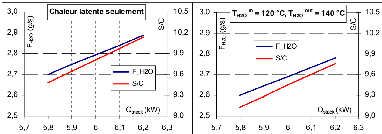
figure IV. 19 : débit du circuit d'eau en fonction de Q_{\text{stack}} , pour deux écarts de température
