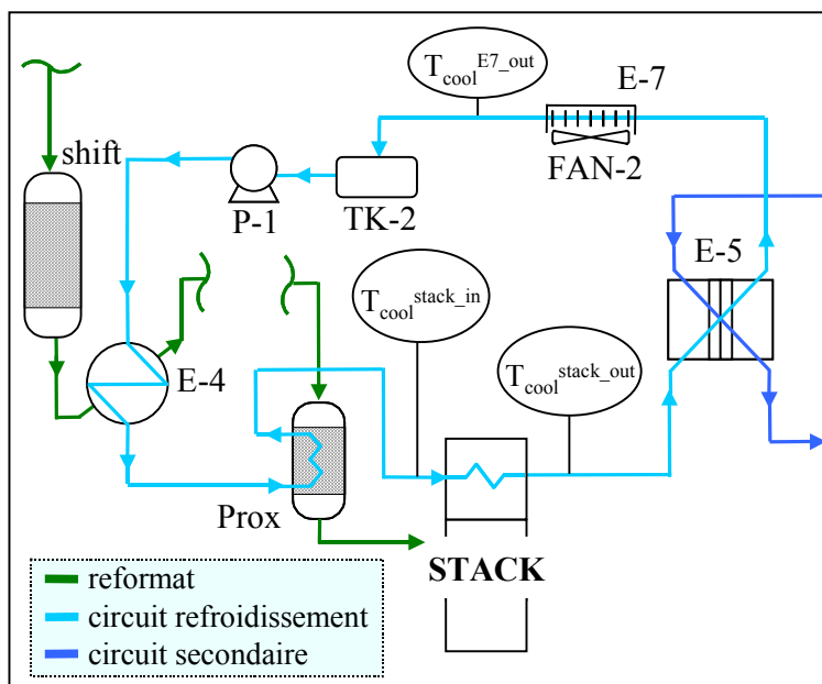
figure III. 4 : circuit de refroidissement et températures
