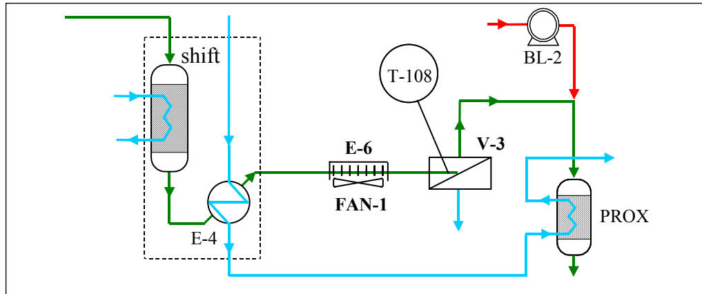
Figure 4 : extrait du schéma de procédé
