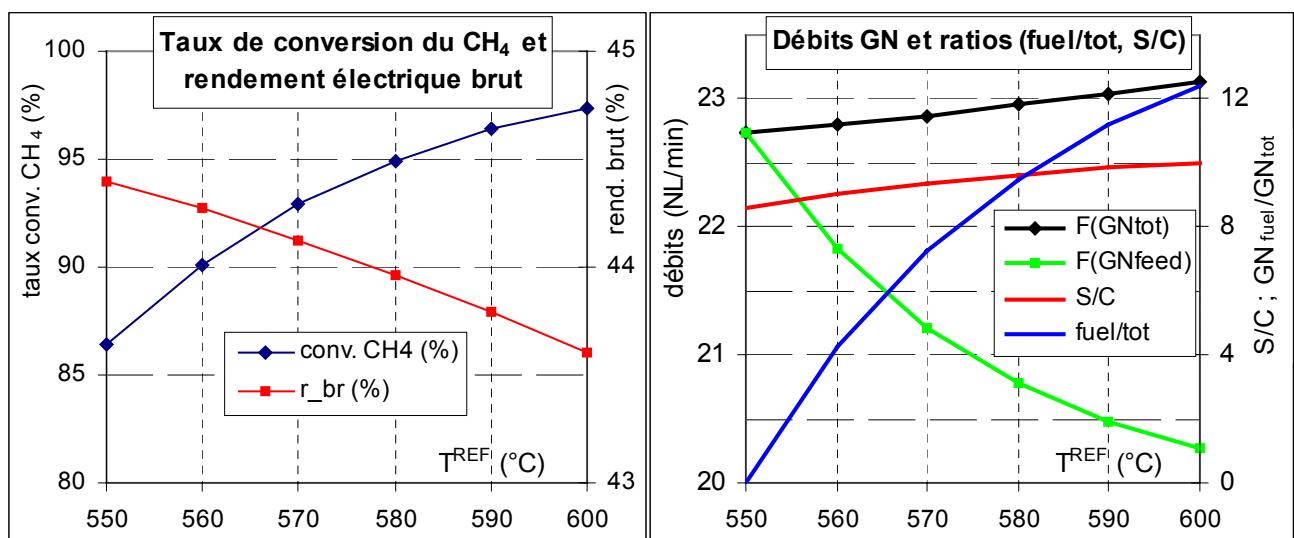
figure IV. 21 : rendement brut, taux de conversion (g.), débits et ratios en fonction de T REF (dr.)
