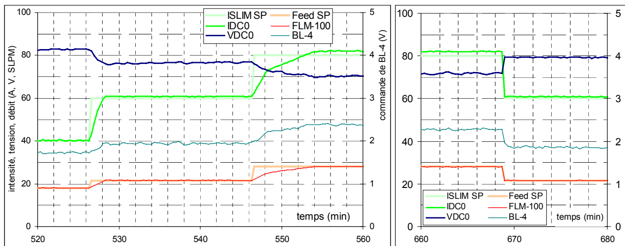
figure II. 21 : suivi de consigne pour deux échelons montant (g.) et un échelon descendant (dr.)
