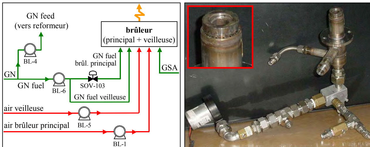
figure II. 5 : schéma de l'alimentation du brûleur et photo du brûleur démonté (photo Gaz de France)
