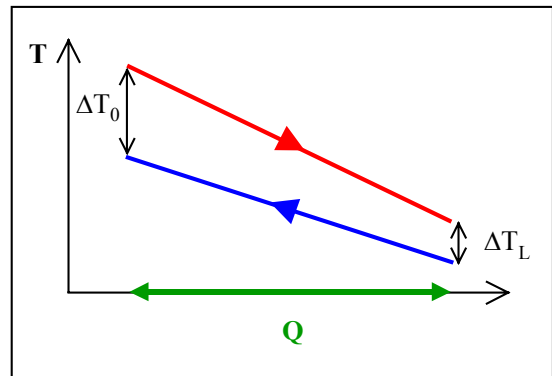
figure II. 18 : graphique flux vs. températures
