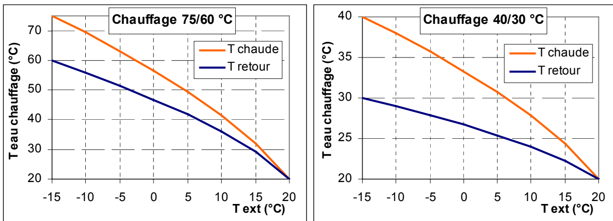
figure IV. 6 : courbes de chauffe pour T^{CH}/T^{FR} = 75/60\text{ °C} (g.) et 40/30\text{ °C} (dr.), avec T_{int} = 20\text{ °C} [VIESS]
