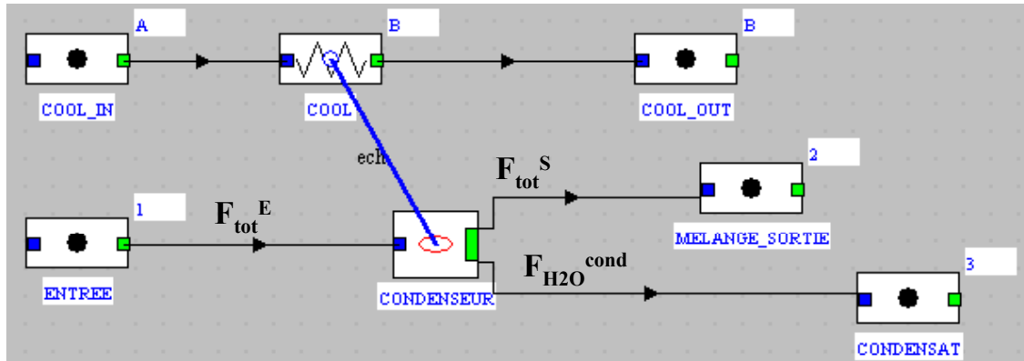
Figure 1 : écran du composant CONDENSEUR et de son environnement sous Thermoptim
