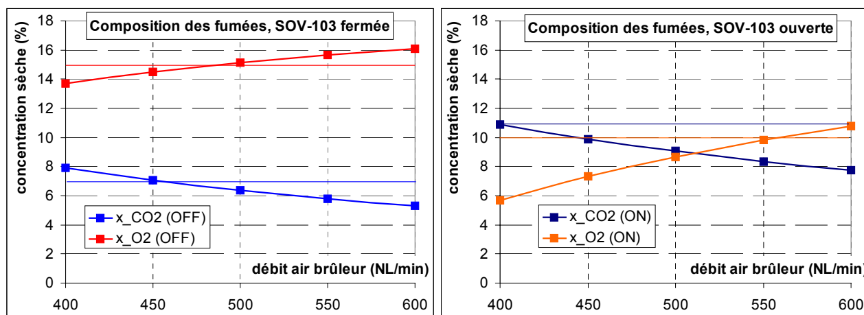
figure III. 5 : compositions sèches calculées des fumées pour SOV-103 fermée (g.) et ouverte (dr.). La valeur mesurée est rappelée par la droite de même couleur
