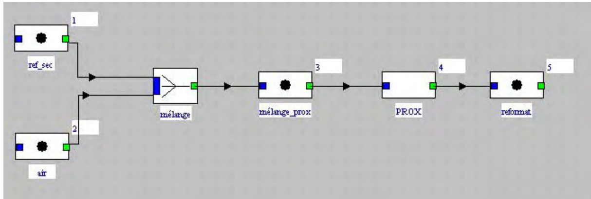
Figure 1 : schéma du composant PROX et de son environnement sous Thermoptim
