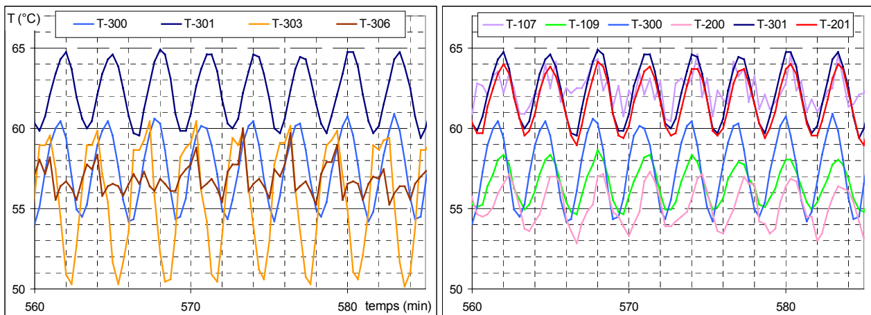
figure II. 24 : températures des circuits primaire et secondaire (g.), du reformat et de l'air cathode (dr.)
