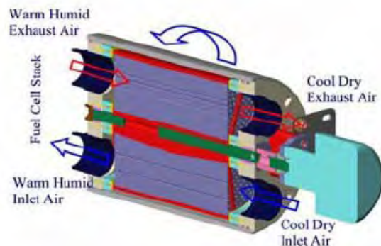
Fig. 1 : schéma issu de la documentation constructeur
