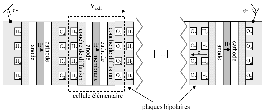
figure I. 8 : schéma d'un stack (l'échelle n'est pas respectée, contrairement à la figure I. 6)
