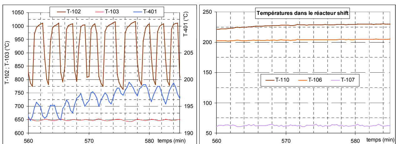
figure II. 22 : températures dans le bloc reformeur (g) et dans le réacteur shift (dr.)
