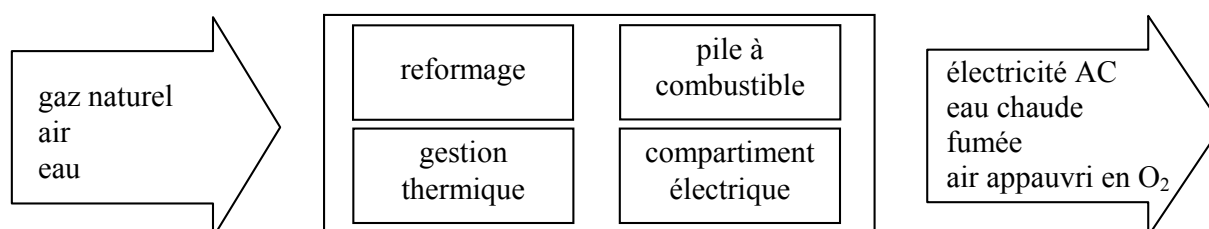
Schéma générique d'un petit cogénérateur basé sur une PEMFC et alimenté en gaz naturel
