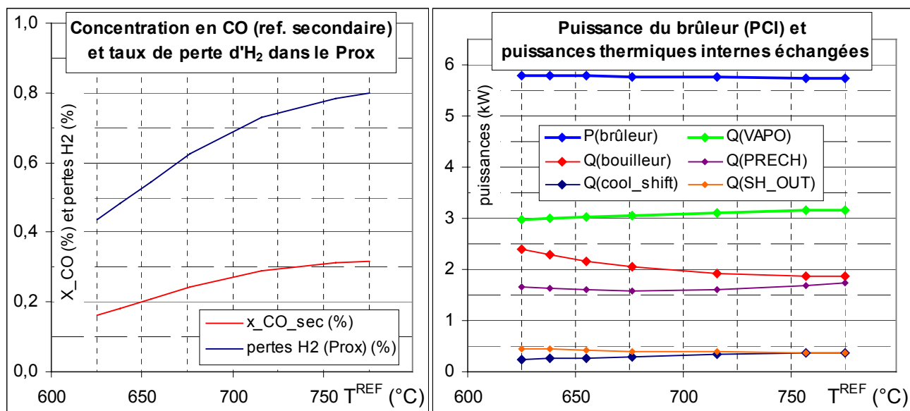
figure IV. 3 : fraction sèche de CO dans le reformat secondaire et pertes en H_2 dans le Prox associées (g.) ; puissances thermiques échangées dans le procédé (dr.)
