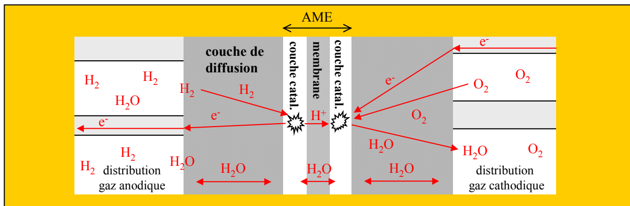
figure I. 6 : vue schématique d'une cellule de pile à combustible PEM (échelle respectée dans la direction perpendiculaire au plan de la membrane)
