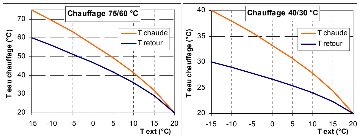
Fig. a et b : Courbes de chauffe pour 75/60 °C et 40/30 °C avec T_{int} = 20 °C [VIESS]
