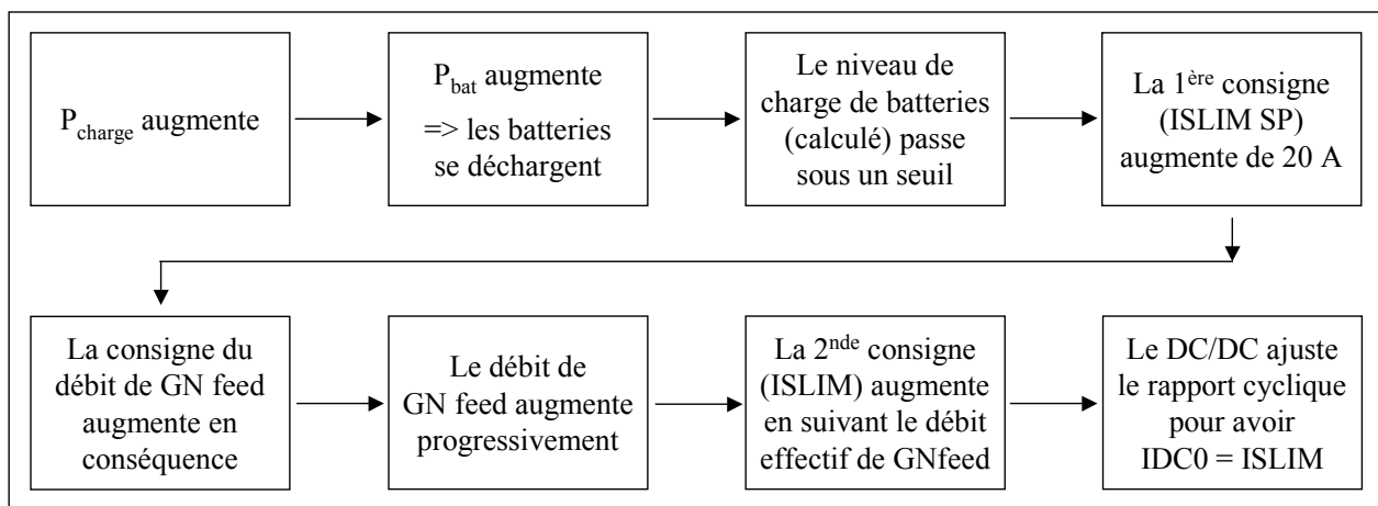
figure II. 12 : schéma simplifié de la régulation électrique
