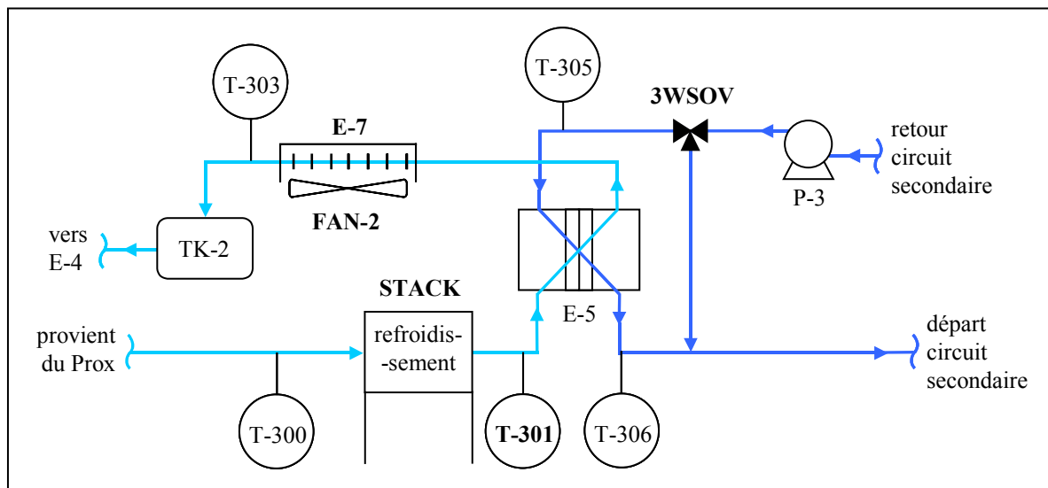
Figure 5 : schéma du circuit de refroidissement au niveau du stack et du circuit secondaire
