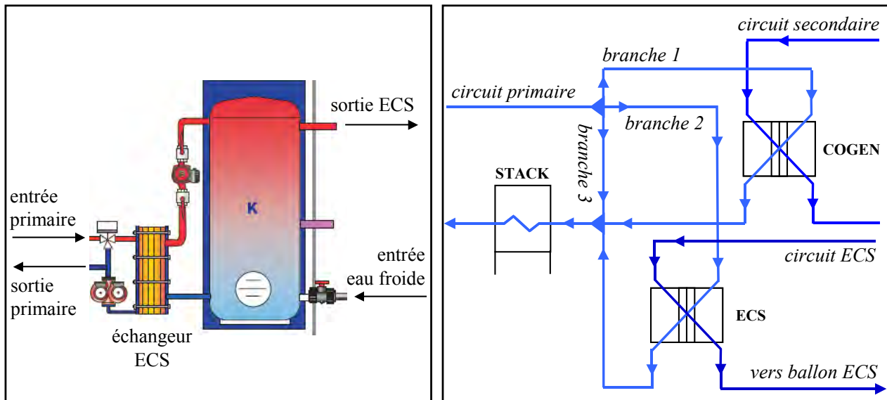
figure IV. 16 : exemple de ballon stratifié avec échangeur à plaques externe (g.), schéma hydraulique (dr.)
