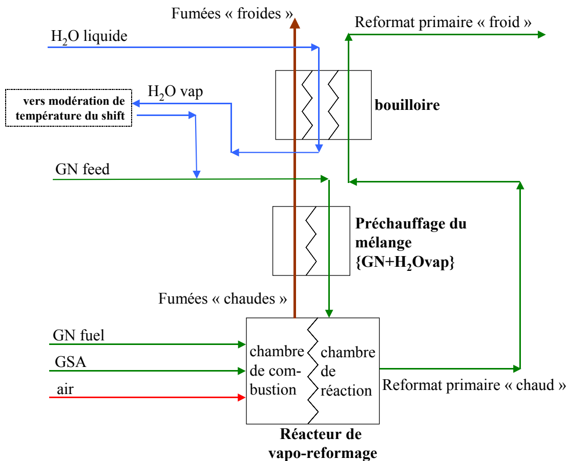
Figure 1 : vue éclatée de l'ensemble du bloc reformeur, constitué de réacteur de vapo-reformage, du préchauffage du mélange réactif et de la bouilloire à deux fluides chauds
