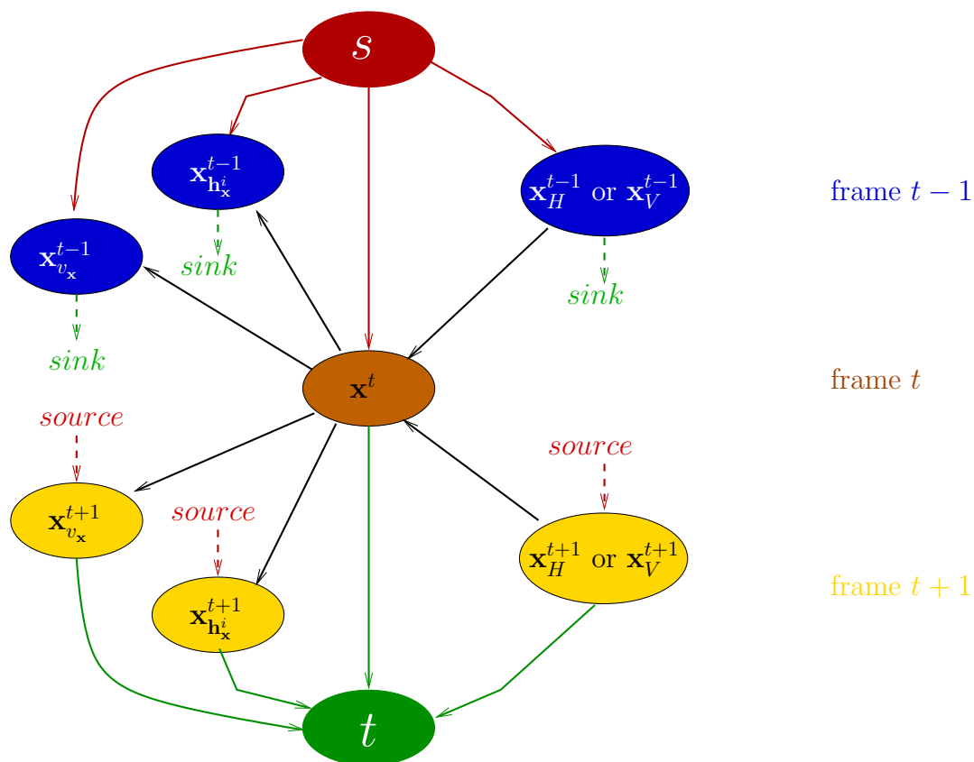
FIGURE 5.8 – Construction du graphe : les t -links vers la source sont en rouge, les t -links vers le puit en vert. Pour une (V, \mathbf{h}^V = \text{false}) -expansion donnée (ou \mathbf{h}^H -expansion), les n -links temporeux sont en noir et relient le pixel \mathbf{x} (image t ) aux pixels \mathbf{x}_{v_x}, \mathbf{x}_{h_x^i}, \mathbf{x}_V (or \mathbf{x}_H ) des images t - 1 et t + 1 . Note : pour la clarté, seuls les liens relatifs à la i^e couche cachée sont montrés.
