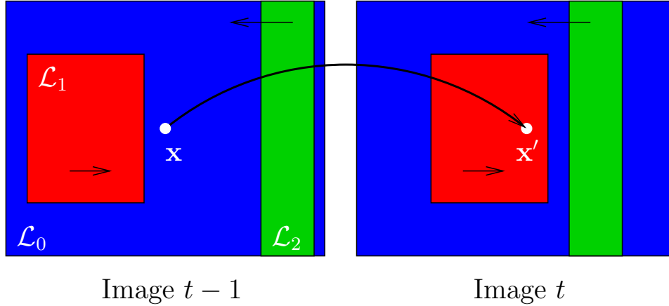
FIGURE 4.4 – Il y a ici trois couches l_0, l_1, l_2 (respectivement en bleu, rouge et vert), le pixel blanc \mathbf{x} et son projeté \mathbf{x}' = \mathcal{T}_0(\mathbf{x}) . Le tableau 4.1 résume pour les trois cas possibles (selon l'étiquette de \mathbf{x}' ) la pénalité définie par la fonction d_V . Note : aucune couche n'étant cachée en \mathbf{x} , la fonction d_H est toujours nulle.
