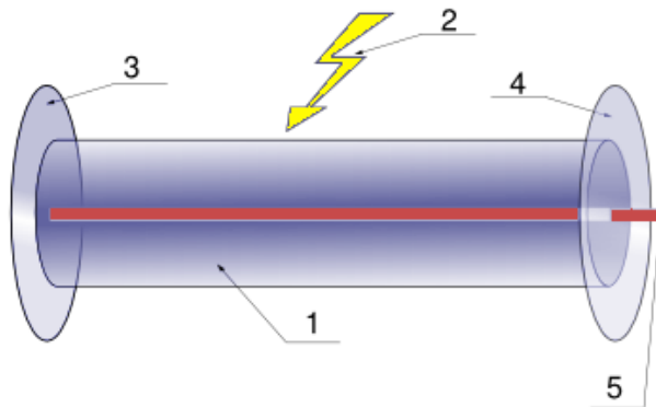
FIGURE 8.7 – Principe du laser : une source énergétique (2) excite le réservoir d'électrons solide, liquide ou gazeux (1) qui génère alors des photons. Ceux-ci rebondissent contre le miroir totalement réfléchissant (3) et le miroir semi-réfléchissant (4). Leur énergie augmente au fur et à mesure des aller-retours. Une partie de ces photons sort du réservoir via le miroir (4) donnant alors le faisceau lumineux directif (5).
