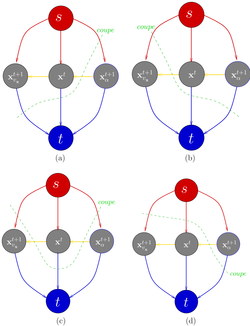
FIGURE 5.9 – Quatre exemples de coupes : (a) l'étiquette de \mathbf{x}^t ne change pas, seule l'étiquette de \mathbf{x}_{v_x}^{t+1} est considérée; (b) même cas que (a) sauf que le pixel \mathbf{x}_{v_x}^{t+1} voit son étiquette passer à \alpha rompant ainsi la cohérence temporelle. La coupe est alors pénalisée par le poids de l'arête \mathbf{x}_{v_x}^{t+1} \rightarrow \mathbf{x} ; (c) même cas que (b) sans influence sur l'étiquette de \mathbf{x}_{\alpha}^{t+1} ; (d) l'étiquette de \mathbf{x} passe à \alpha et seule l'étiquette de \mathbf{x}_{\alpha}^{t+1} est alors considérée et est ici pénalisée via l'arête \mathbf{x}_{\alpha}^{t+1} \rightarrow \mathbf{x} .
