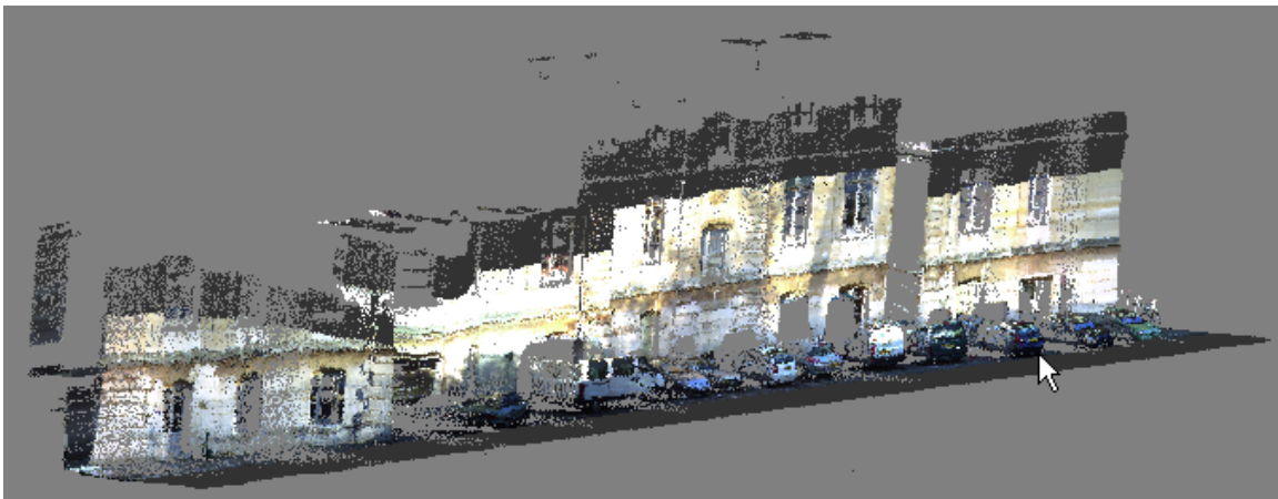
FIGURE 9.10 – Nuage de points obtenu à partir d’une succession de profils télémétriques. Les couleurs sont obtenues à partir de photographies prises simultanément et projetées sur le nuage de points.
