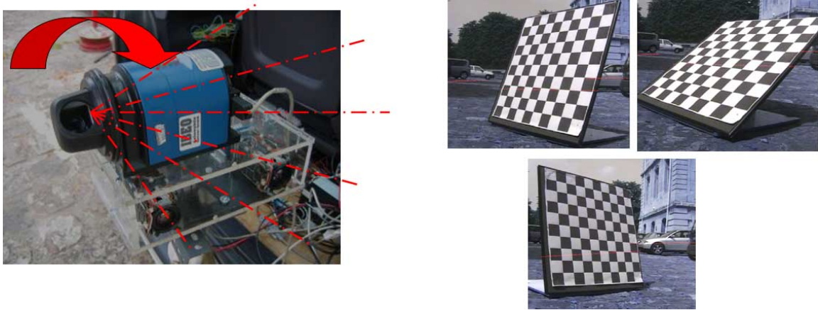
FIGURE 5 – Calibration sur mires des capteurs photographiques et télémétriques, rigidement fixés sur un bloc.
