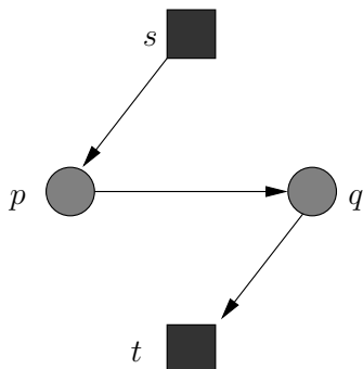
FIGURE 5.4 – Construction du graphe de l' alpha-expansion : arêtes orientées pour les contraintes spatiales et temporelles. Les poids sont donnés dans le tableau 5.1.
