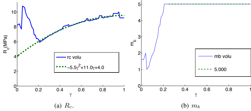
FIG. II.25 – Variations du critère de Høek-Brown
