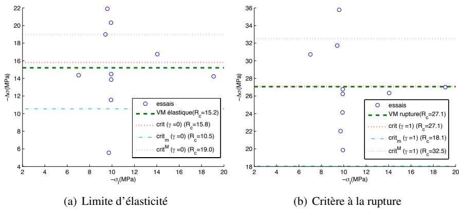
FIG. II.21 – Limite élastique et rupture pour la famille isochoire
