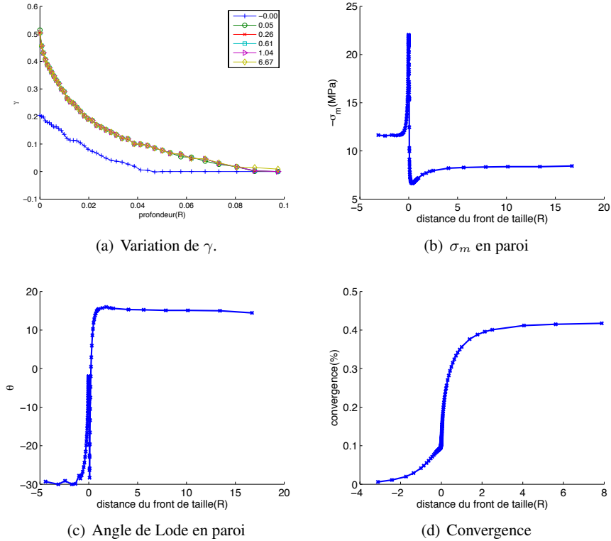
FIG. IV.9 – Évolution en fonction de l'avancement (famille isochores)
