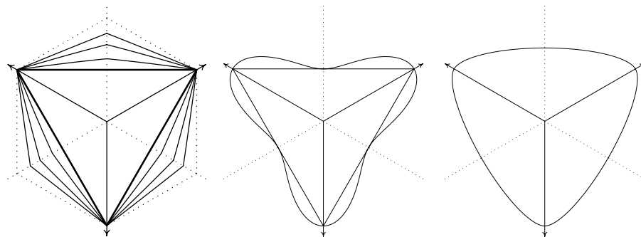
(a) Formes du critère de Høek-Brown en fonction de la pression moyenne (b) L_S = 0.5 . Critère triangulaire et forme régulière non William-Wanke ( L_S = 0.7 ) convexe(I.32)
