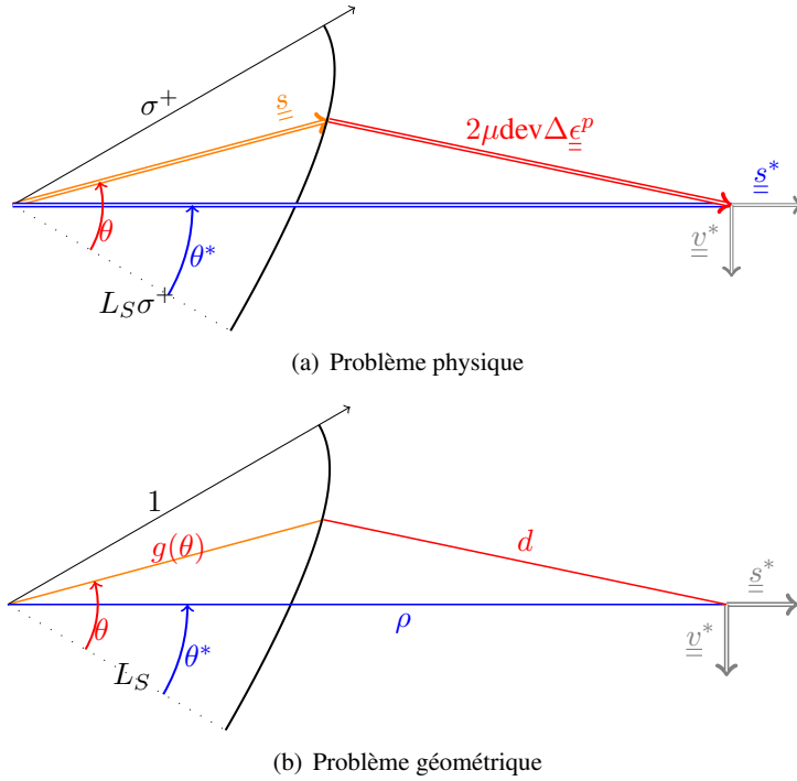
FIG. III.20 – Équivalence entre les problèmes
