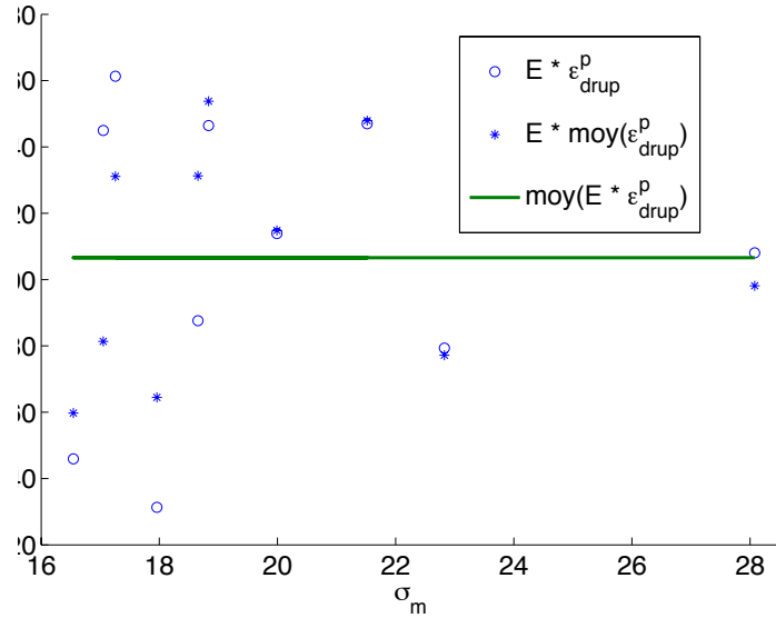
FIG. II.24 – Valeurs de E\epsilon_{drup}^p mesurées, valeur moyenne, et comparaison avec E_{moy}\epsilon_{drup}^p
