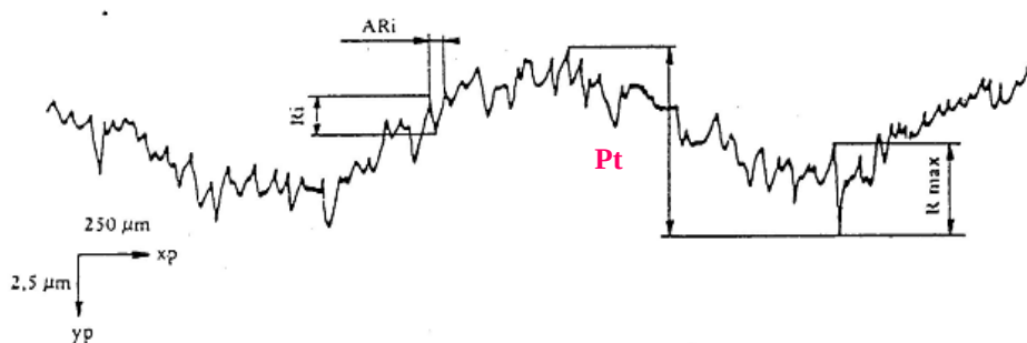
Fig. III-35 : Définition des critères de rugosité
