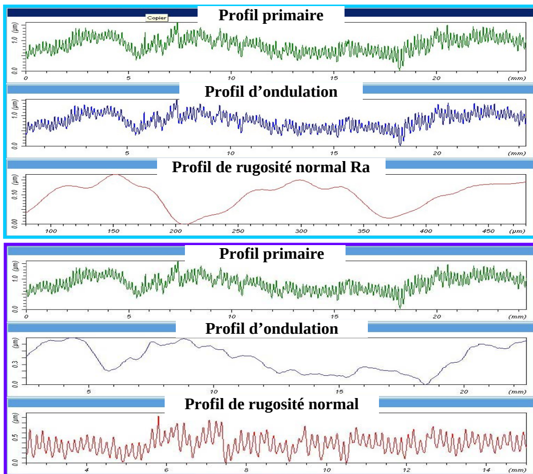
Fig. III-38 : Influence de la longueur de coupure sur la valeur du Ra
