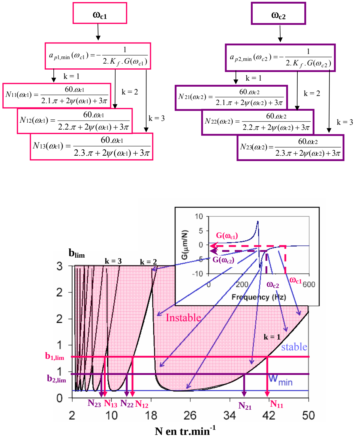
Fig. II-8 : algorithme de calcul des lobes de stabilité en tournage orthogonal
