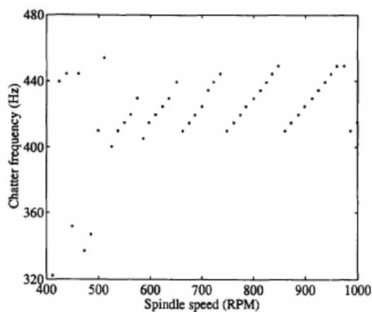
Fig. II-49 : f_c fonction de N [31]
