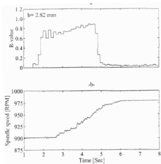
Fig. II-39 : Résultat de l'essai réalisé avec a_e=50\% , f=200 \text{ m.min}^{-1} , a_p=2.82 \text{ mm} , \text{rampe}_{\text{max}}=30 \text{ tr.min}^{-1}.\text{s}^{-1} , \text{rampe}_{\text{min}}=6 \text{ tr.min}^{-1}.\text{s}^{-1} [31]
