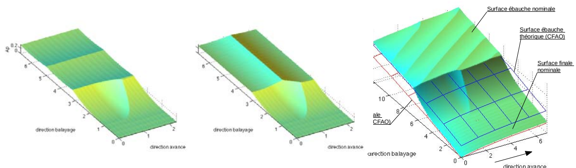
Fig. VI-1 : différentes configurations de balayage de la passe d'ébauche
