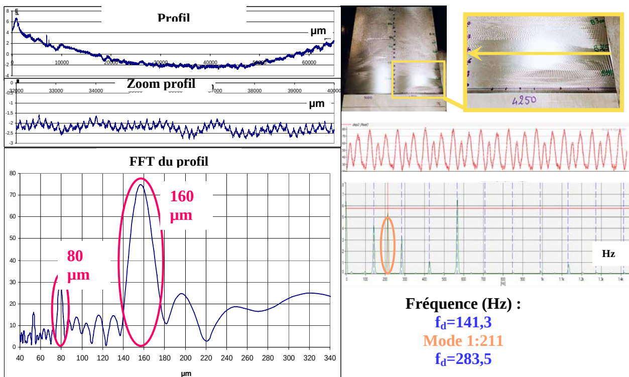
Fig. III-44 : Cas stable : Usi_v=0.26 , N=4250 \text{ tr.min}^{-1}
