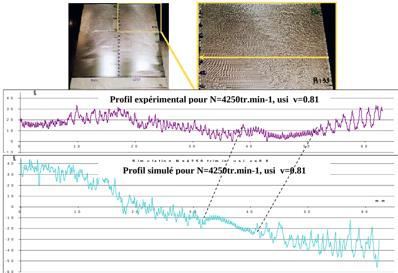
Fig. V-6 : comparaison entre profil simulé et expérimental pour N=4250 \text{ tr.min}^{-1} , usi v=0.81
