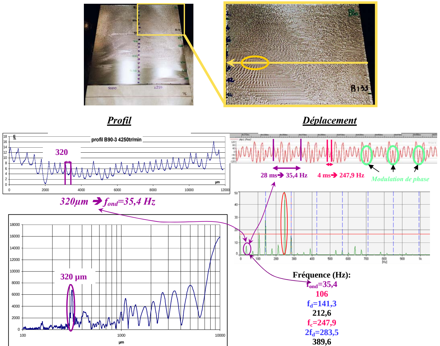
Fig. III-45 : Cas instable : Usi_v=0.80 , N=4250 \text{ tr.min}^{-1}
