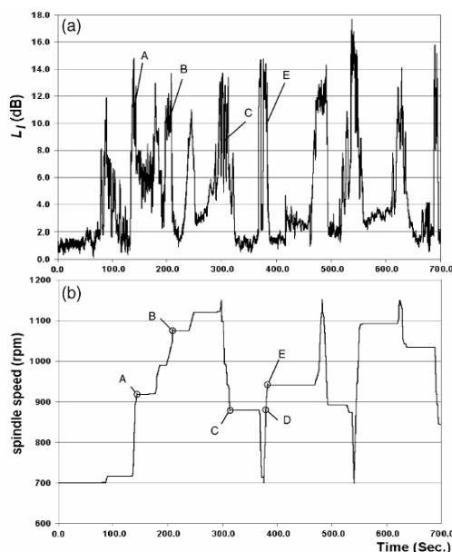
Fig. II-42 : résultat de la variation de vitesse lors d'une passe. (a) intensité sonore mesurée, (b) vitesse de rotation [32]
