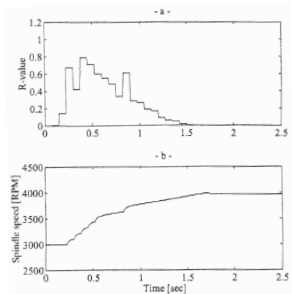
Fig. II-40 : Résultat de l'essai réalisé avec a_e=50\% , f=0.1 \text{ mm.dt}^{-1} , a_p=9 \text{ mm} , \text{rampe}_{\text{max}}=2000 \text{ tr.min}^{-1}.\text{s}^{-1} , \text{rampe}_{\text{min}}=1500 \text{ tr.min}^{-1}.\text{s}^{-1} [31]
