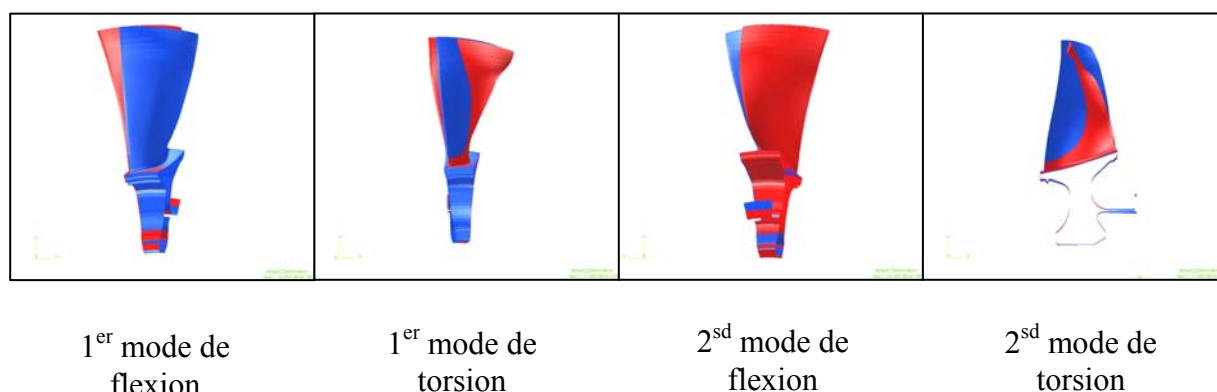
Fig. III-7 : Visualisation des modes propres de l'aube seule
