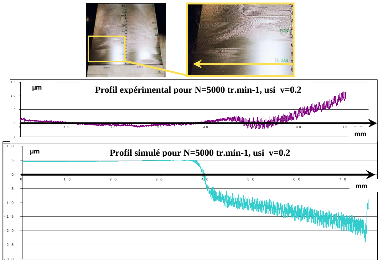
Fig. V-8 : comparaison entre profil simulé et expérimental pour N=5000 \text{ tr.min-1} , usi v=0.2
