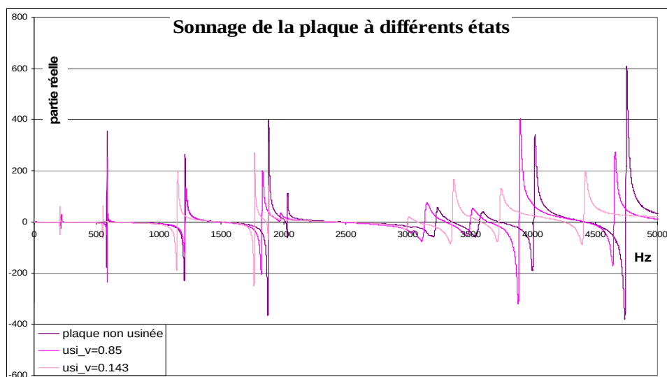
Fig. III-16 : fonction de transfert du système plaque + montage à différents états d'usure
