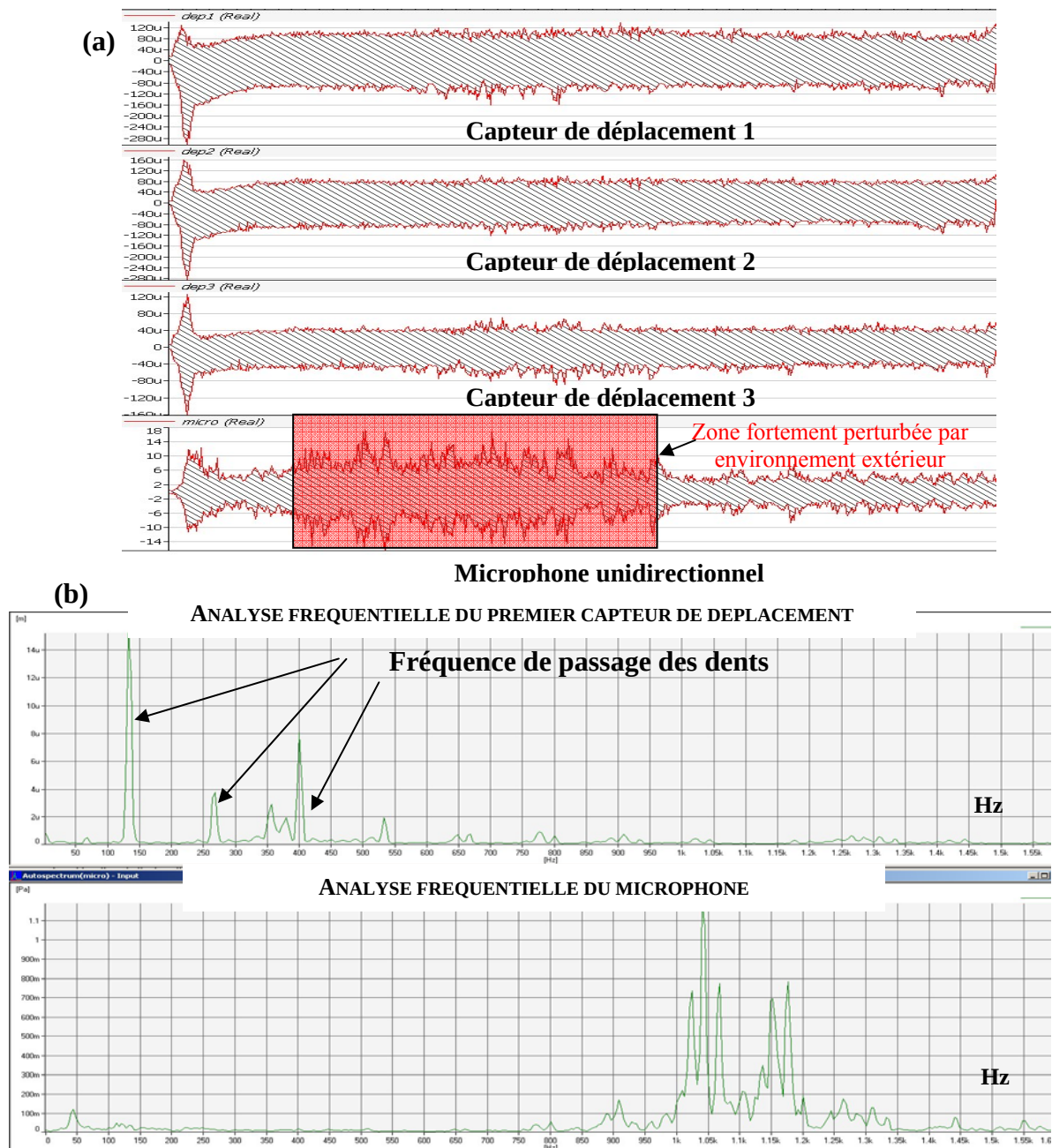
Fig. III-30 : (a) Signaux temporels enregistrés lors de l'usinage de la plaque 2 sur une bande à 4250 tr.min -1 en haut de la plaque, (b) Auto spectre du capteur de déplacement 1 et du micro calculés sur la partie matérialisée en rouge sur la figure.
