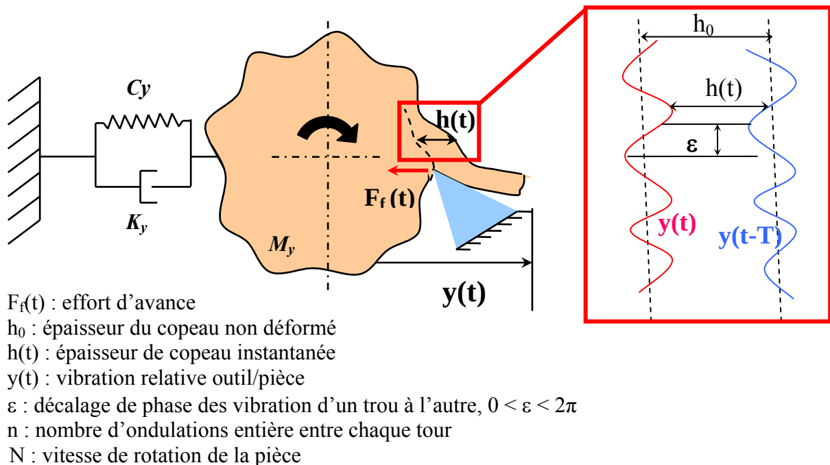
Fig. II-5 : Schématisation du procédé de tournage
