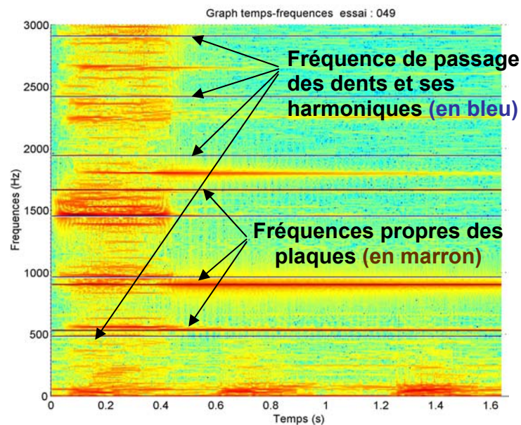
Fig. II-30 : spectrogramme obtenu lors de l'usinage d'une plaque mince bridée par deux cotés [15]
