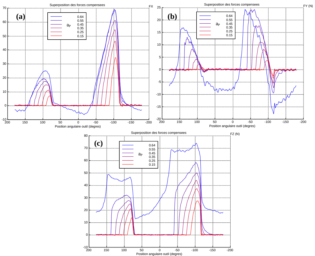
Fig. III-29 : mesure des effort de coupe pour un dépinçage de 25 : (a) dans la direction de l'avance, (b) perpendiculaire à l'avance, (c) normal au plan d'usinage
