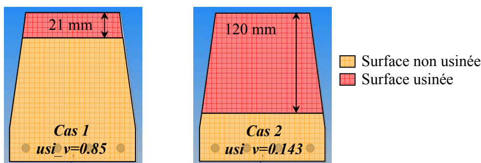
Fig. III-15 : schéma correspondant aux deux états de la plaque étudiés
