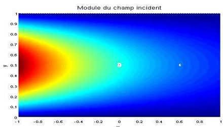
FIG. 4.17 – Emission du premier vecteur propre k = 3 . (guide d'ondes)
