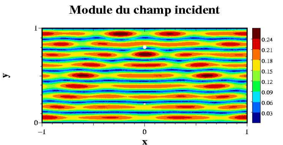
FIG. 4.35 – Emission du second vecteur propre k = 30 . (guide d'ondes)
