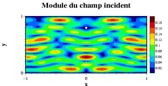
FIG. 4.37 – Emission du quatrième vecteur propre k = 30 . (guide d'ondes)
