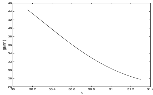
FIG. 4.5 – Gain associé à la première valeur propre. (disques disposés selon une horizontale)
