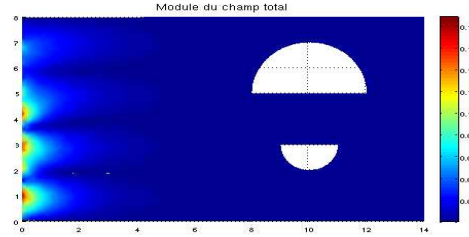
FIG. 4.53 – Champ total associé à l'émission du quatrième vecteur propre k = 1.4 . (guide d'ondes)
