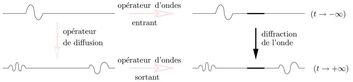
FIG. 5.1 – Opérateurs d'ondes et opérateur de diffusion.
