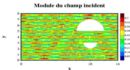
FIG. 4.71 – Champ incident associé à l'émission du premier vecteur propre k = 6 . (guide d'ondes)
