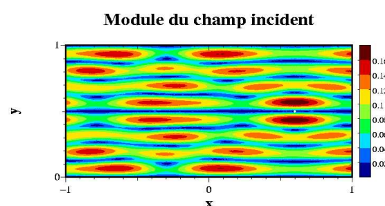
FIG. 4.30 – Emission du second vecteur propre k = 30 . (uniquement le petit obstacle est présent dans le guide)
