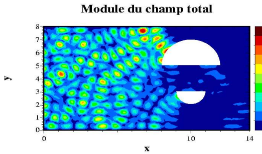
FIG. 4.68 – Champ total associé à l'émission du troisième vecteur propre k = 6 . (guide d'ondes)
