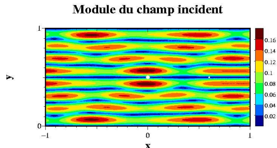
FIG. 4.24 – Emission du second vecteur propre k = 30 . (guide d'ondes)
