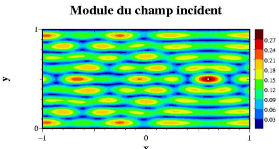
FIG. 4.29 – Emission du premier vecteur propre k = 30 . (uniquement le petit obstacle est présent dans le guide)
