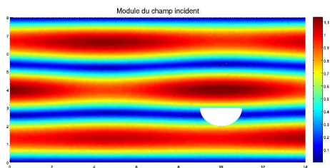
FIG. 4.64 – Champ incident associé à l'émission du premier vecteur propre k = 1.4 . (uniquement le petit obstacle est présent dans le guide)
