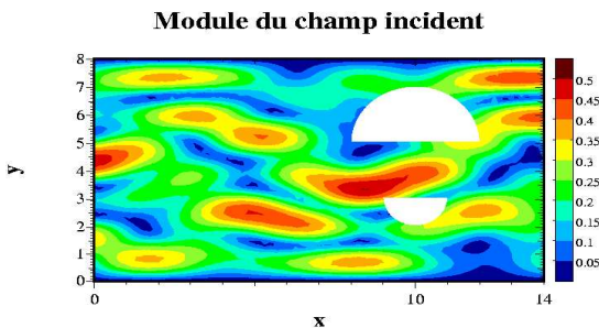
FIG. 4.47 – Champ incident associé à l'émission du troisième vecteur propre k = 6 . (guide d'ondes)
