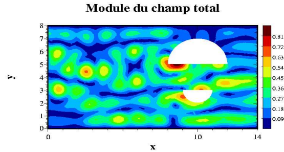
FIG. 4.43 – Champ total associé à l'émission du quatrième vecteur propre k = 3 . (guide d'ondes)
