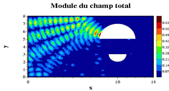
FIG. 4.70 – Champ total associé à l'émission du cinquième vecteur propre k = 6 . (guide d'ondes)
