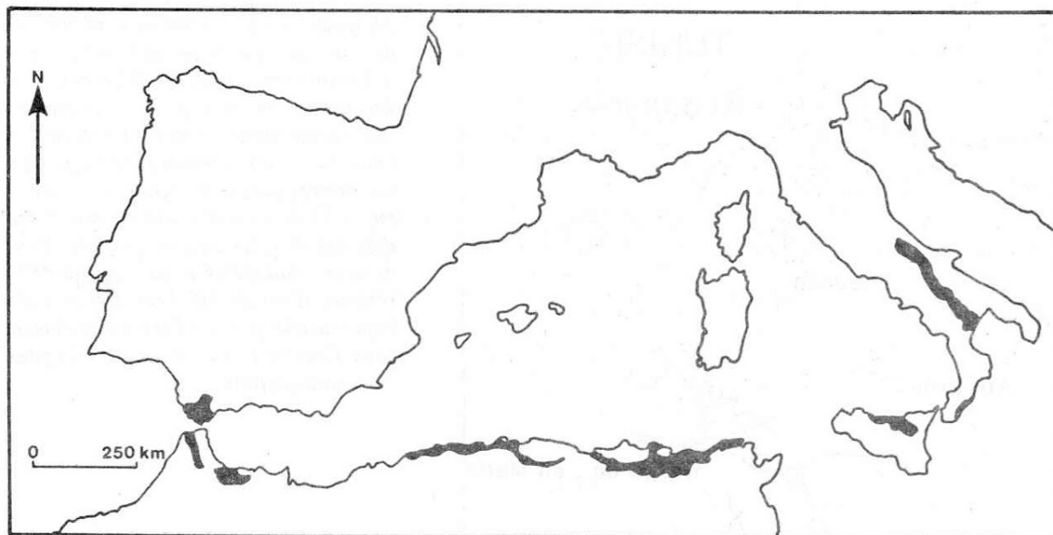
FIG. A.8 – Les principales zones d’affleurement du Numidien (Parize (1988) [120]).
