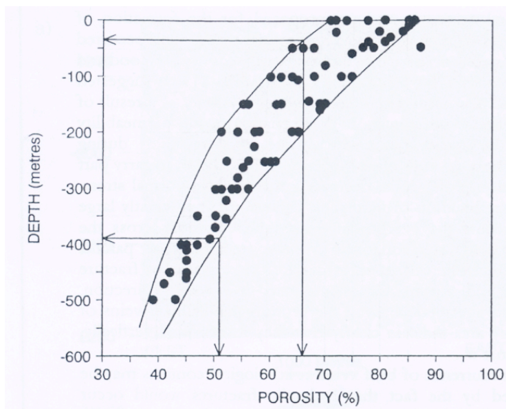
FIG. 2.5 – Relation entre porosité et profondeur pour des sédiments argileux sous faible recouvrement (d’après Velde, 1996 [160]), compilation de données ODP et DSDP. Remarque : Une porosité de 50 - 70 % correspond à un enfouissement de 40 à 400 m sous le paléofond de mer.
