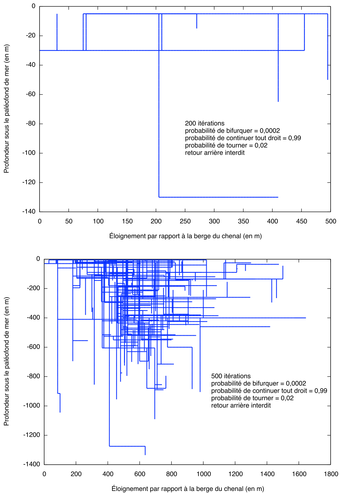
FIG. 6.4 – Influence du nombre d'itérations sur le nombre de bifurcations.
