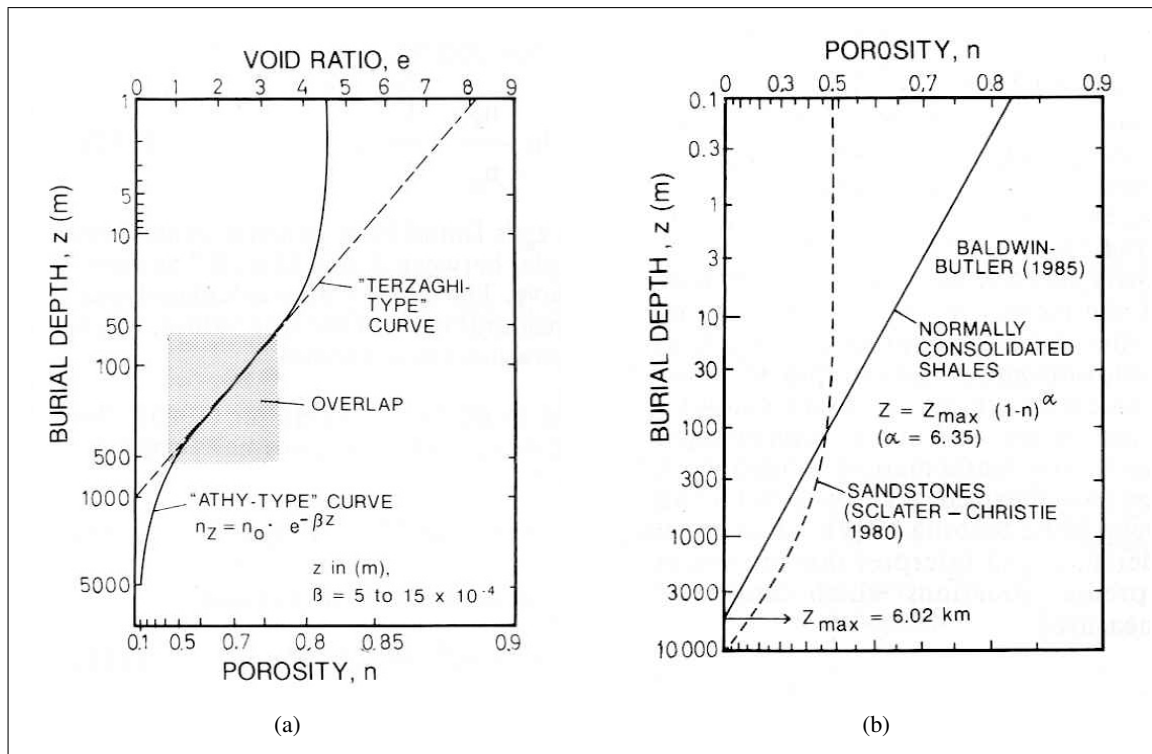
FIG. 3.3 – Représentation de différentes courbes de porosité ou d'indice des vides en fonction de la profondeur (dans Einsele, 1992 [49]). (a) Comparaison entre une courbe de Terzaghi et une courbe d'Athy, en utilisant une échelle logarithmique pour la profondeur et la porosité et une échelle linéaire pour l'indice des vides. (b) Représentation de courbes de porosité à l'aide d'équations puissance.
