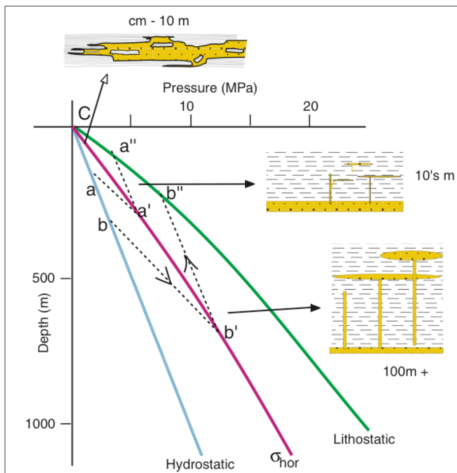
FIG. 2.4 – Modèle simple pour montrer comment la taille d'un complexe de sillons et de dykes clastiques est fonction de la profondeur à laquelle est scellé le corps sableux et de la profondeur où la couverture se rompt. Ce modèle est valable pour les bassins où la contrainte maximale principale est verticale (chargement gravitaire). A de très faibles profondeurs, les contraintes différentielles ( \sigma_v - \sigma_h ) sont petites et l'anisotropie due à la stratification favorise la formation de sillons plutôt que de dykes. Si un corps sableux se scelle à une faible profondeur (point a), la pression fluide dévie du gradient hydrostatique. Dans le cas le plus simple où aucun autre fluide de pore n'entre dans le corps sableux, la pression fluide augmente avec la profondeur d'enfouissement en suivant le gradient hydrostatique. Lorsque la pression fluide atteint la contrainte horizontale minimale ( \sigma_h ), la couverture se rompt et un dyke se forme (point a'). En supposant qu'il y ait un réservoir suffisamment grand de fluide sous pression, le dyke va se propager vers le haut jusqu'à ce que la pression fluide dépasse la pression lithostatique ( \sigma_v ) et un sillon pourra se former (point a''). Si le corps sableux est scellé à une grande profondeur (point b), la distance de la rupture de la couverture et celle de la formation d'un sillon (b' et b'', respectivement) sont plus grandes. Des dykes plus grands doivent se mettre en place entre le corps nourricier et la profondeur de formation des sillons (dans Jolly et Lonergan, 2002 [86]).
