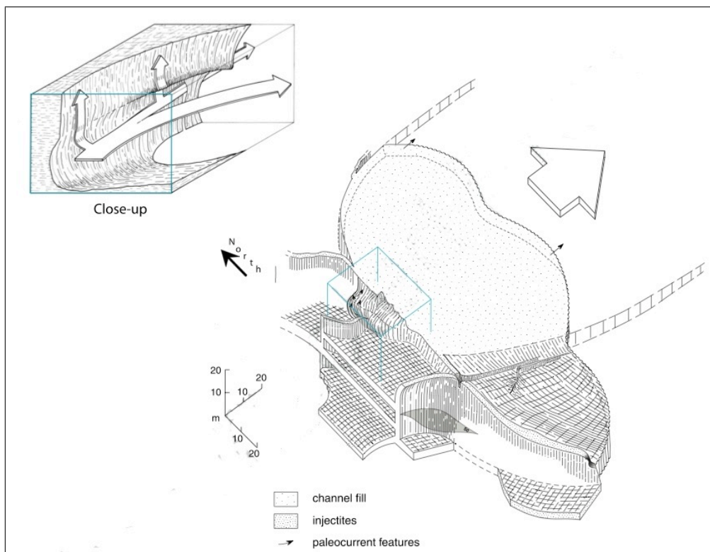
FIG. A.13 – Affleurement de La Baume (d'après Beaudoin et al. , 1985 [15] et Parize et Friès, 2003 [126] dans Parize et al. , 2006 [123]). Cet affleurement couronne la partie sud-est de la colline du Puy et a été cartographié en trois dimensions. Il constitue un des rares arguments de terrain montrant l'hydrofracturation développée pendant le dépôt massif chenalisé du corps nourricier.
