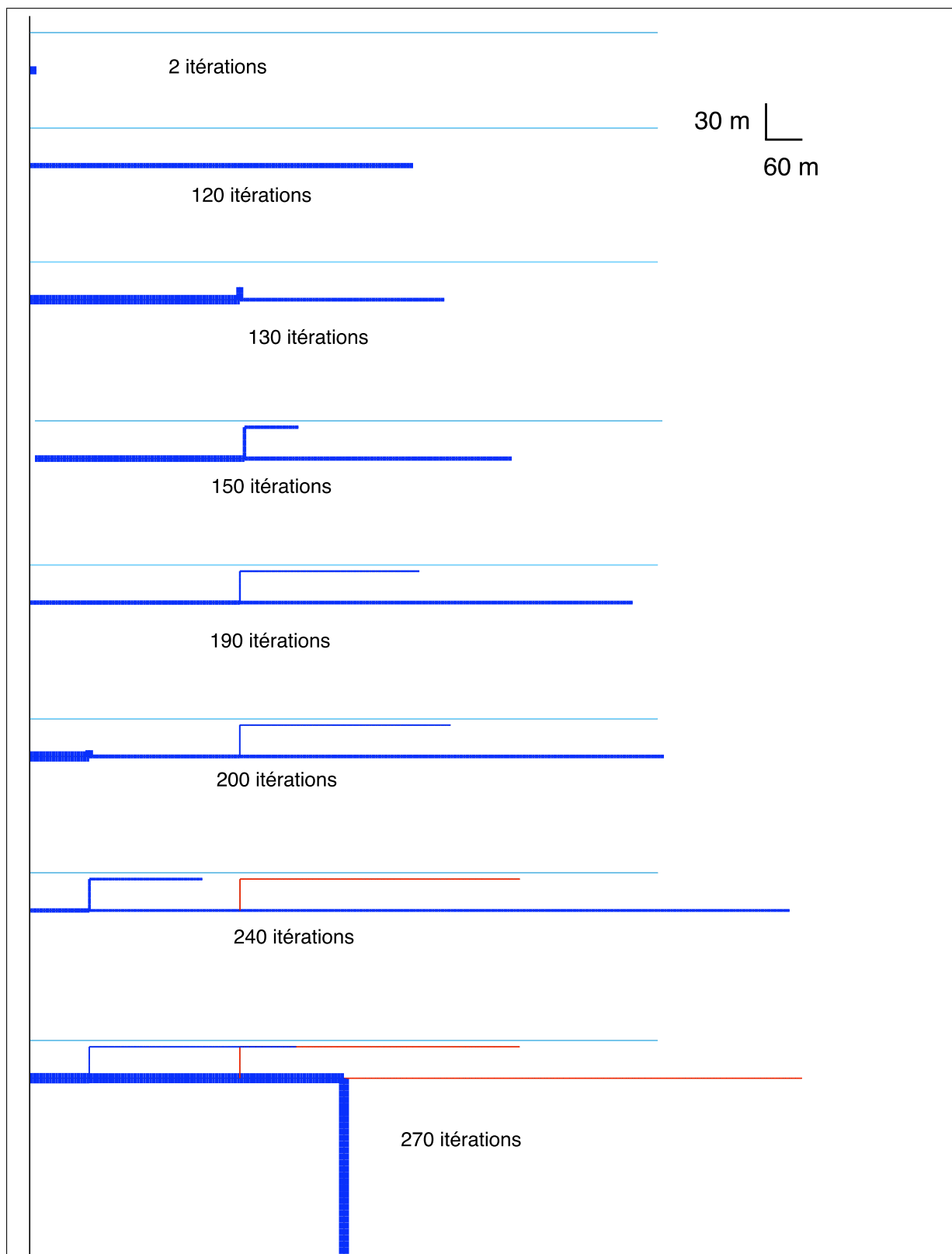
FIG. 6.27 – Représentation du réseau d'injection à plusieurs étapes. La couleur rouge est utilisée pour représenter les branches figées et la couleur bleue pour les branches où le fluide s'écoule. L'épaisseur des traits bleus est proportionnelle à la valeur du débit dans ces branches
