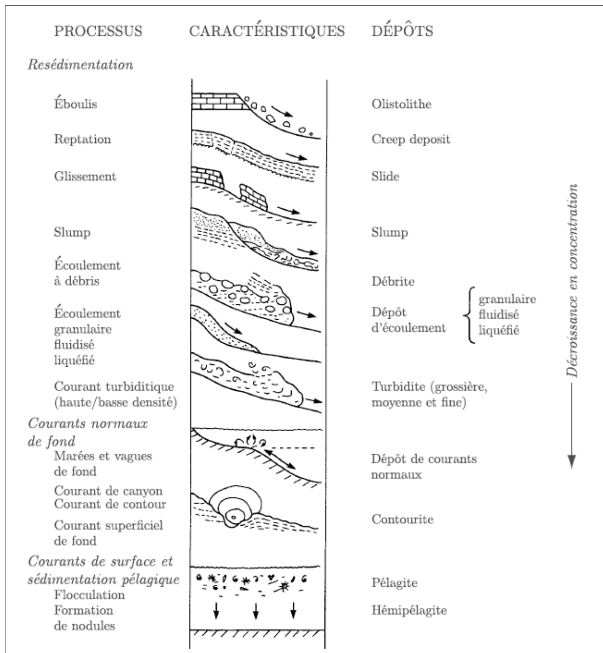
FIG. 3.5 – Les trois groupes de processus opérant en milieu marin profond (d'après Stow, 1986 [148]).
