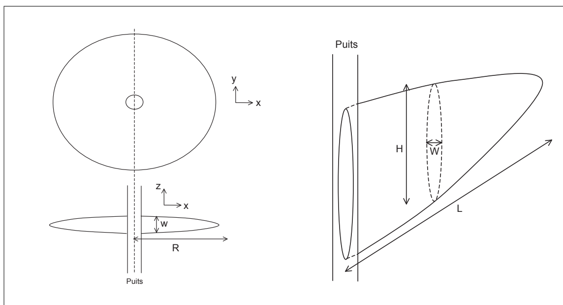
FIG. 5.2 – Coupes schématiques d'une fracture hydraulique horizontale (a) et verticale (b)
