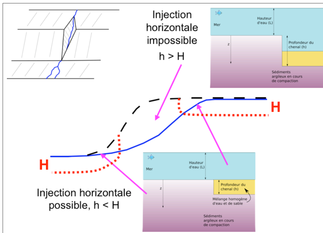
FIG. 4.8 – Schématisation du parcours d'un écoulement turbiditique et localisation des zones potentiellement injectée horizontalement
