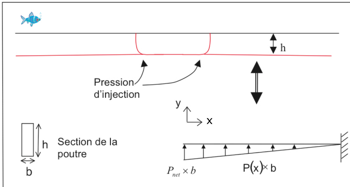
FIG. 5.9 – Schématisation d'une poutre encastrée pour modéliser le soulèvement des berges. Dans ce modèle la largeur b de la poutre est unitaire.
