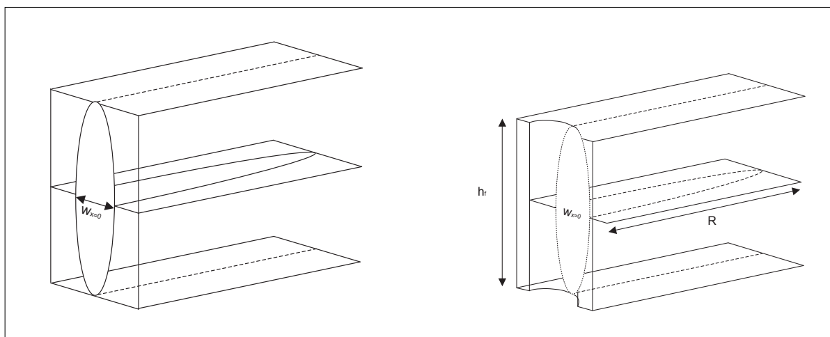
FIG. 5.4 – Modèle PKN
