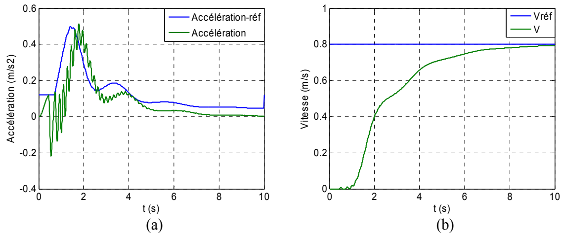
Fig. 3.16 Réponses du VAL 206 en présence de jeux mécaniques : (a) accélération, (b) vitesse
