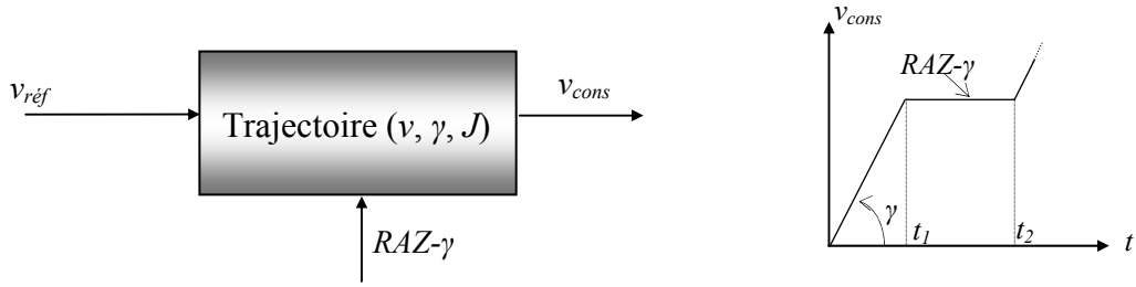
Fig. 2.44 Gestion de la trajectoire de vitesse : (a) principe, (b) blocage accélération
