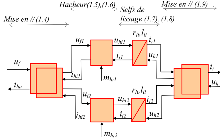
Fig. 1.5 REM du hacheur d'induit
