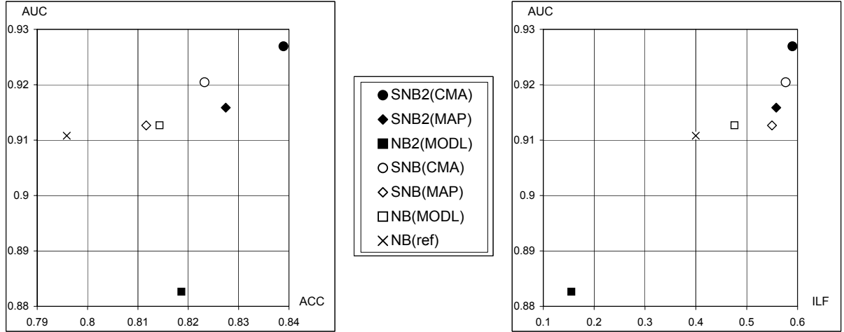
FIG. 4.7 – Moyenne des critères ACC, AUC et ILF pour l'évaluation de classifieurs Bayésiens naïfs sur 30 jeux de données de l'UCI.
