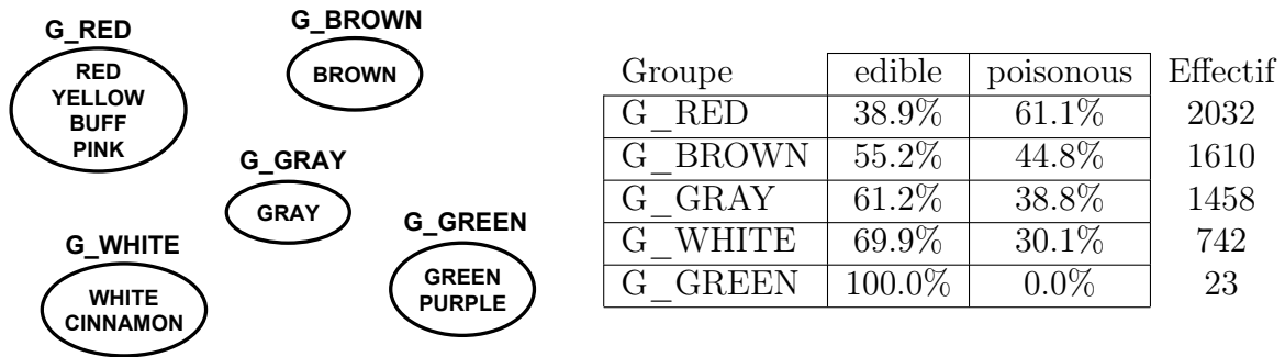
FIG. 2.3 – Exemple de groupement des couleurs de chapeau de champignon.
