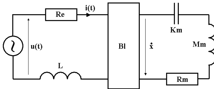
FIG. 5.1 – Modèle de Thiele et Small pour la transduction électromécanique.
