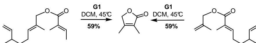
Fig 201 Synthèse de cyclopentènone avec le catalyseur de Grubbs I
