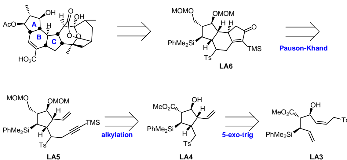
Fig 18 Rétrosynthèse proposée par Landais et al.
