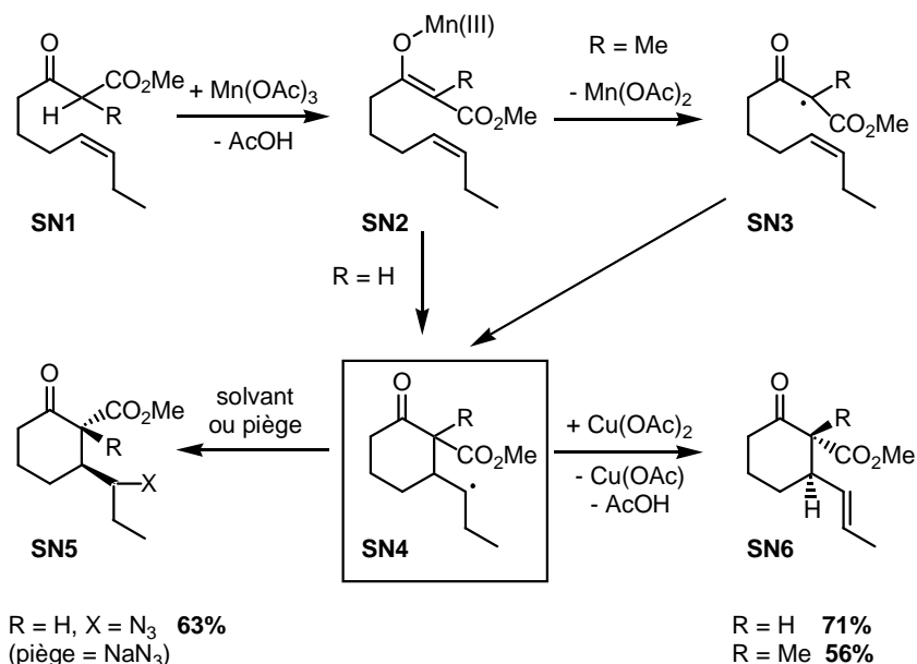
Fig 156 Mécanisme de la cyclisation radicalaire d'un \beta -cétoester présence de \text{Mn(OAc)}_3
