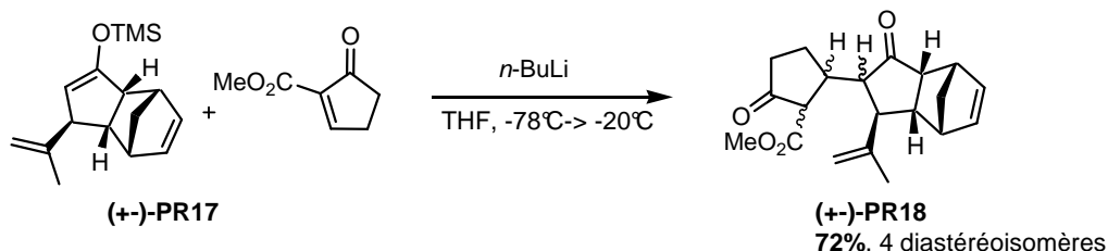
Fig 38 Addition avec un accepteur de Michael doublement activé
