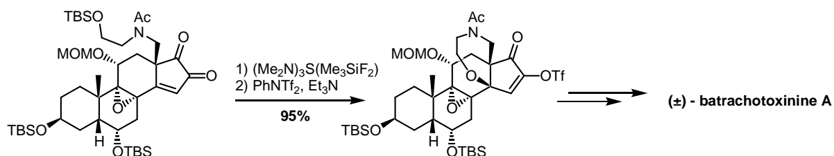
Fig 86 Etape clé de la synthèse de la (±)-batrachotoxinine par Kishi et al
