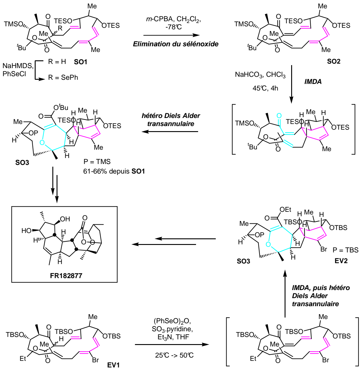
Fig 5 Etape clé des synthèses de Sorensen et Evans
