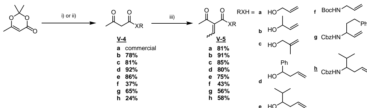
Fig 196 Synthèse des diènes V-5. i) 2,2,6-triméthyl-4H-1,3-dioxin-4-one (1 eq), a-f (1 eq), xylène, reflux, 30 min. ii) 2,2,6-triméthyl-4H-1,3-dioxin-4-one (2 eq), g ou h (1 eq), toluène, reflux, 16-24 h. iii) acétaldéhyde (4.5 eq), \text{TiCl}_4 (1.8 eq), pyridine (3.5 eq), THF, 0°C à 20°C, 16h.
