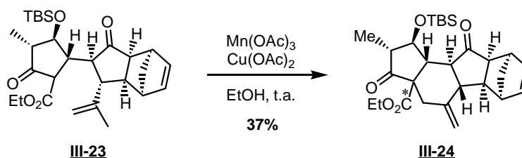
Fig 127 Cyclisation radicalaire
