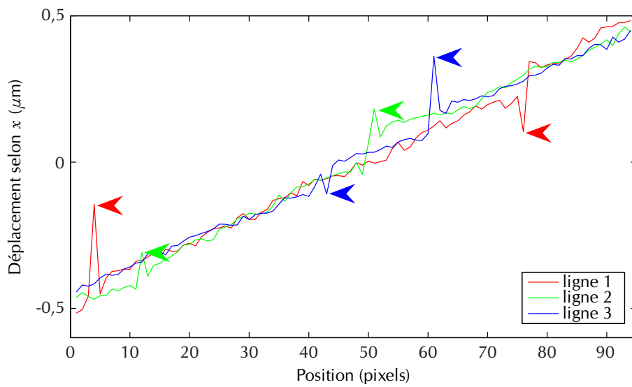
FIG. 4.25 : Carte u_x incrémentale correspondant à une déformation globale de 1,5 % et profil extrait.
