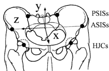
Figure 50: Repère bassin proposé par Leardini (PSIS : épinés iliaques postérieures; ASIS : épinés iliaques antérieures; HJC : centre de la tête fémorale) Issu de (Leardini et coll. 1999)
