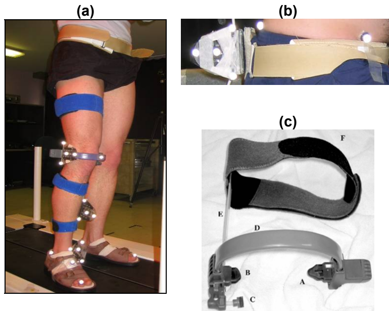
Figure 27: (a) sujet debout sur le tapis roulant, muni de l'ensemble des systèmes d'attache, (b) ceinture sacrale et (c) harnais fémoral (issu de Hagemeister, 2005).
