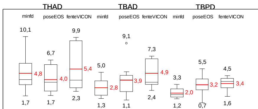
Figure 23: Erreur de recalage des marqueurs THAD, TBAD et TBPD avec 3 remplacements de marqueurs (2 sujets)
