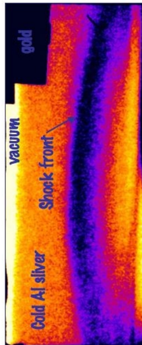
Figure A.1: Radiographie X d'une cible d'Al choquée. Le retard entre le faisceau ps et les faisceaux ns est de 8 ns.
