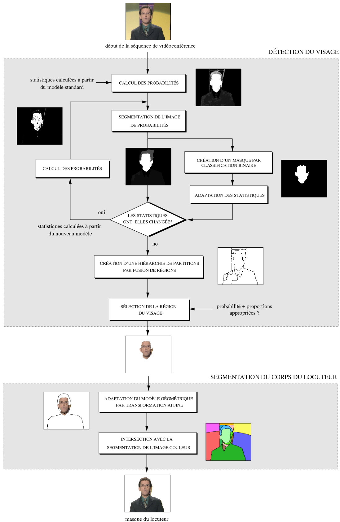
FIG. 9.7 – Schéma de la procédure d'initialisation automatique.
