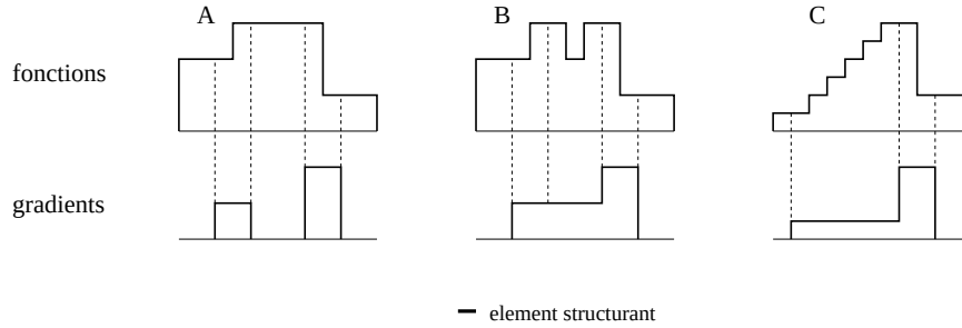
FIG. 4.2 – Gradient morphologique calculé sur trois signaux en une dimension.
