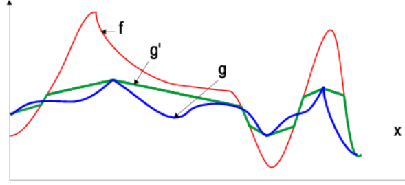
FIG. 3.11 – Construction du lambda nivellement.
