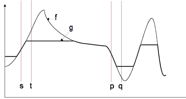
FIG. 3.8 – Définition des nivellements.
