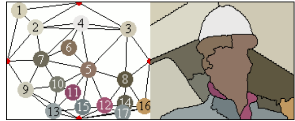
(c2) Graphe B' - Partition B'
