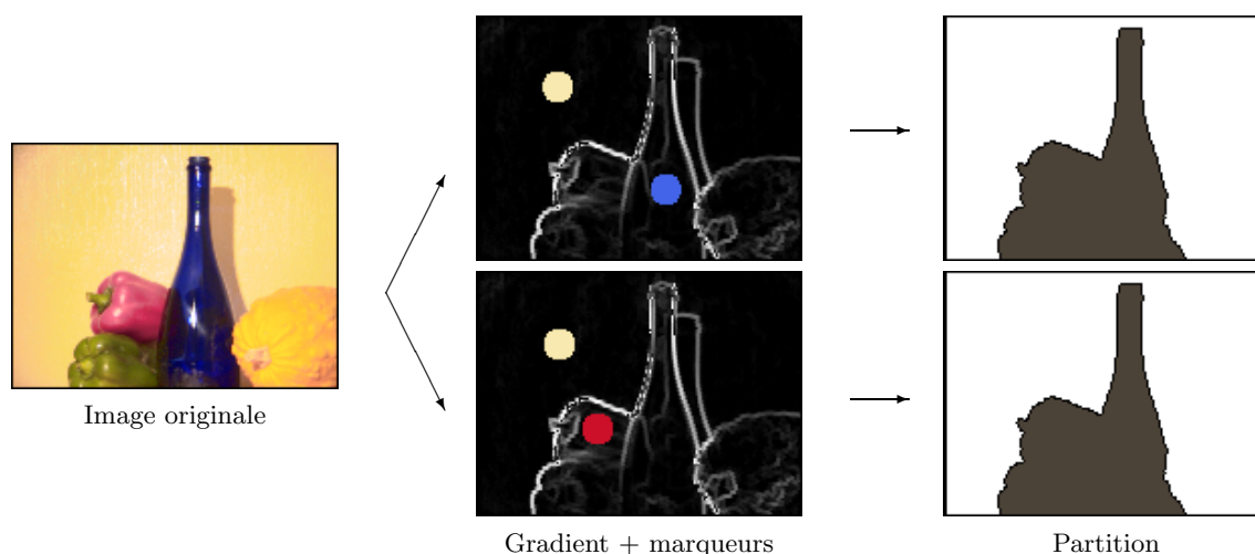
FIG. 4.9 – LPE classique calculée à partir de marqueurs.
