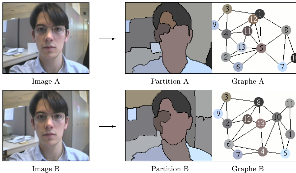
FIG. 6.4 – Problématique liée à la mise en correspondance de partitions.
