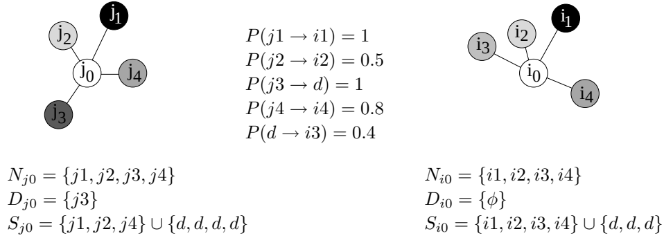
FIG. 6.10 – Calcul des voisinages de projection.
