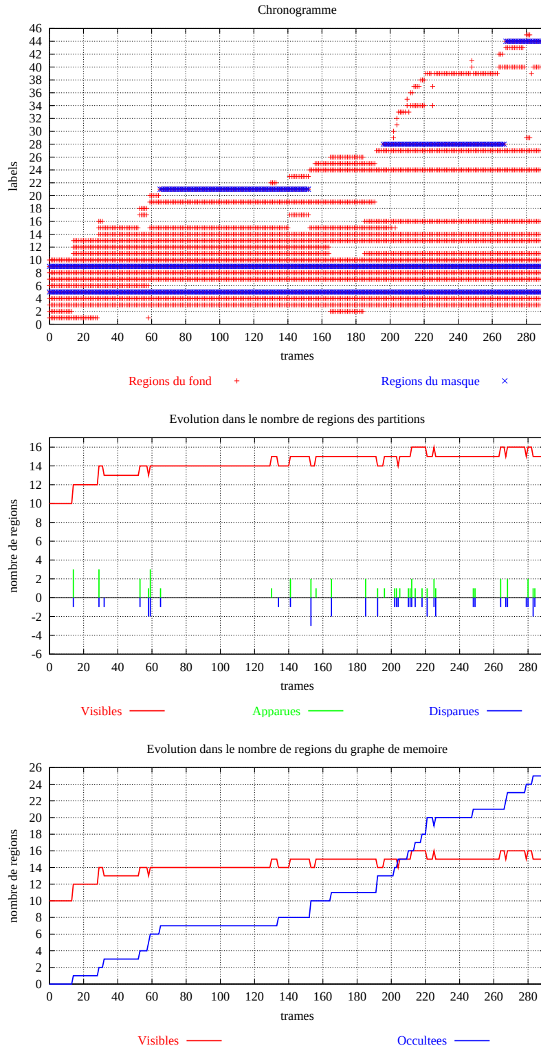
FIG. 7.17 – Séquence « Mother and daughter ». Chronogramme des noeuds. La séquence de masques de la Figure 7.10 (b) a été créée par suivi des labels : visage (9, 23, 44), cheveux (5) et bras (21).
