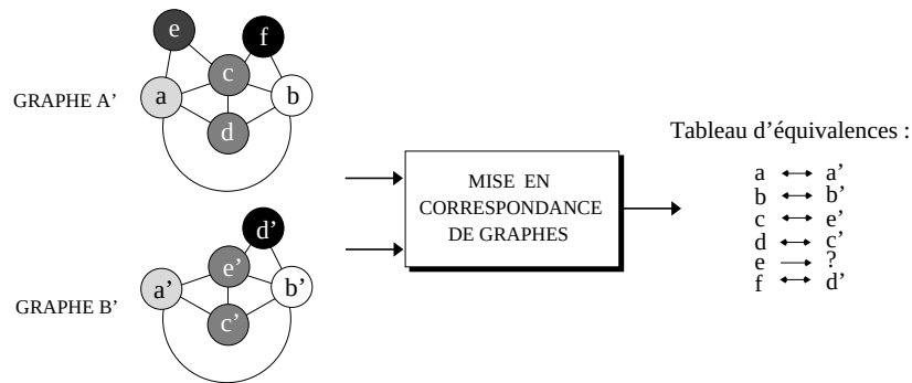
Etape 2 : mise en correspondance des graphes par relaxation probabiliste.
