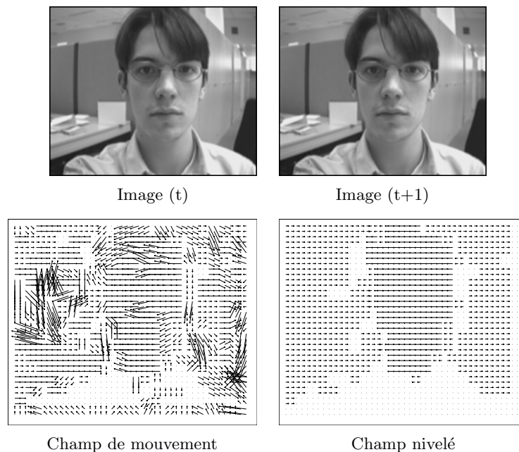
FIG. 3.23 – Nivellement d'un champ de mouvement.
