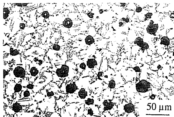
fig. II.40 - Germination de l'austénite dans les joints de grain lors d'un nouveau chauffage à 870\text{ °C} d'un échantillon comparable à celui de la figure II.39
