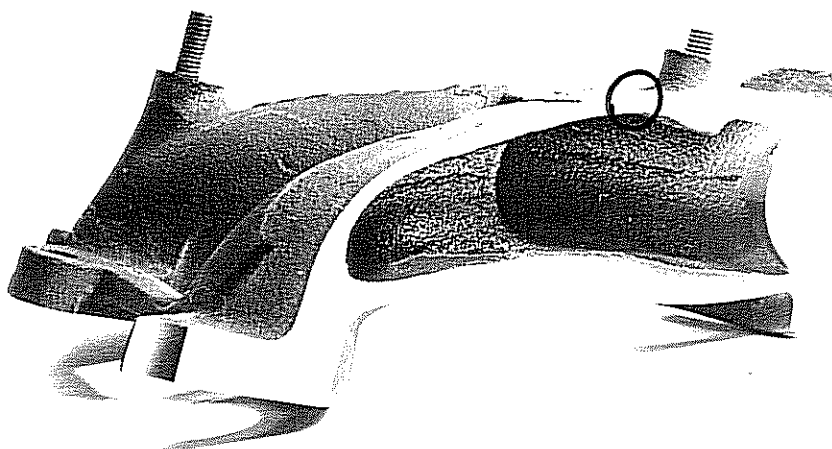
fig. 1.16 - Coupe polie d'un collecteur ayant été testé sur banc sans s'endommager
