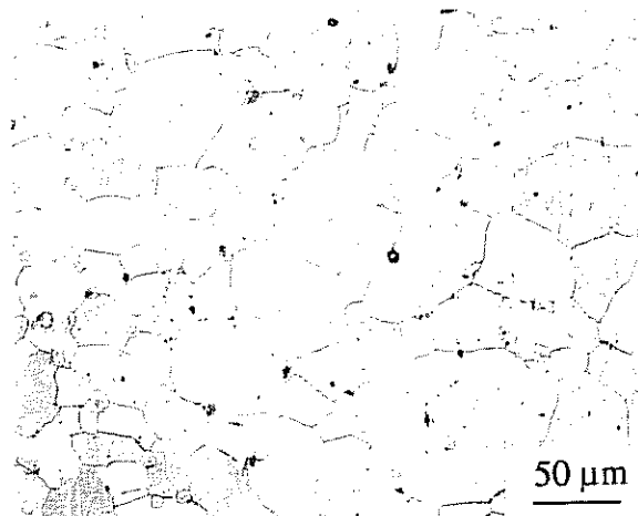
fig. II.16 - Exemple de décarburation non poreuse
