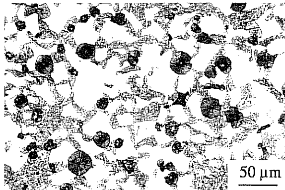
fig. II.39 - Structure biphasée de la matrice d'une fonte SiMo après 2 jours à 870\text{ °C}
