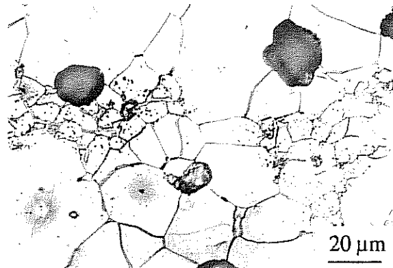
fig. II.18 - Précipités ayant résisté à un traitement de 6 jours à 855 °C
