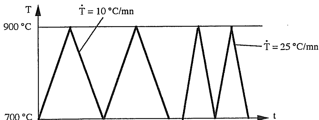
fig. III.41 - Chargement thermique appliqué à l'éprouvette de fonte GS50
