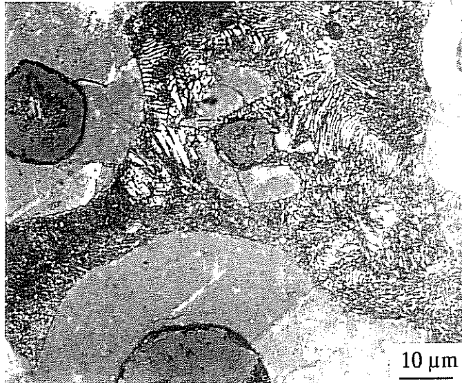
fig. I.1 - Perlite présente dans une fonte GS à matrice ferrito-perlitique
