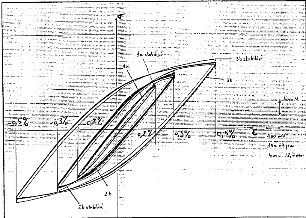
Ecrouissage cyclique
