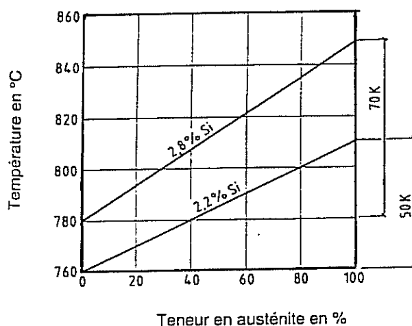
fig. I.8 - Evolution de la teneur en austénite en fonction de la température pour différents taux de Silicium [Wustenfeld, 1993]
