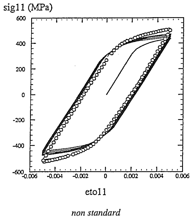
fig. III.30 - Simulation de l'écroutissage cyclique à 300 °C
