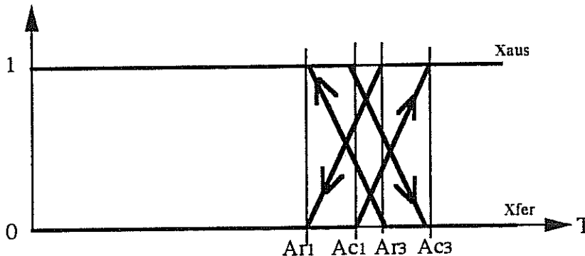
fig. III.5 - Variation des fractions de ferrite et d'austénite
