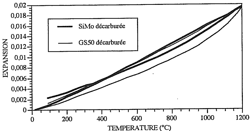
fig IV.23 - Dilatométrie sur GS50 et SiMo décarburees
