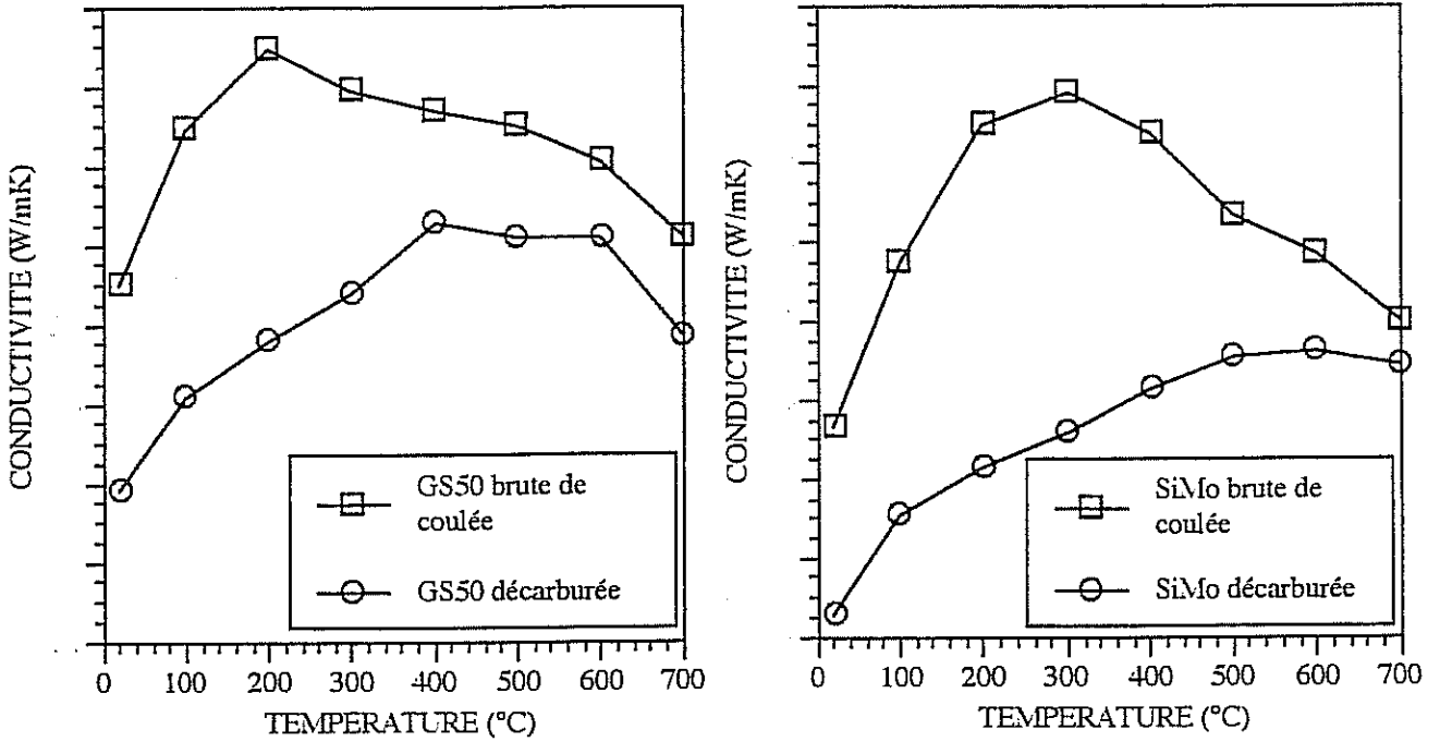
fig. III.17 - Evolution de la conductivité thermique
