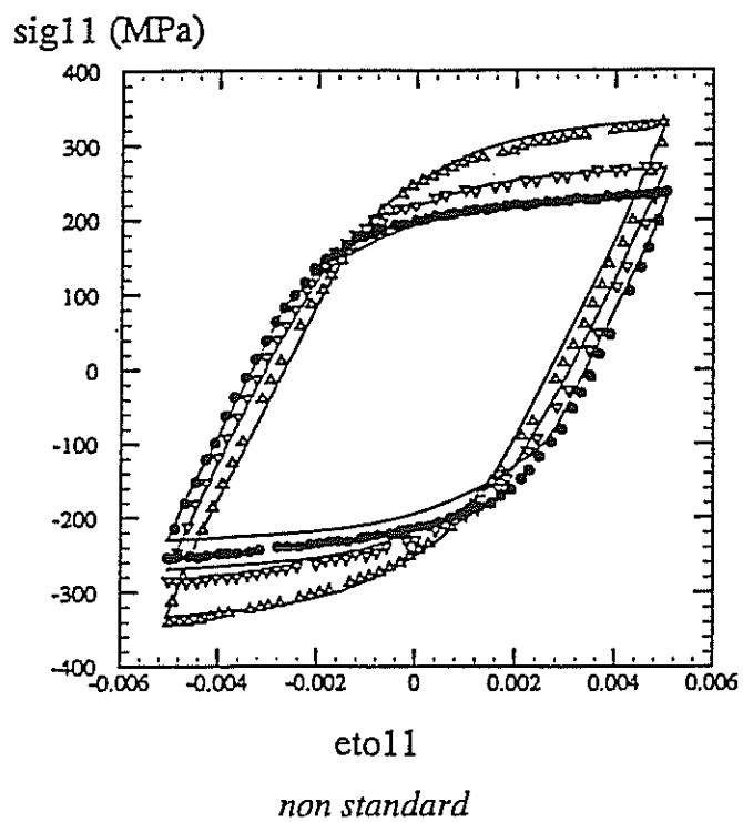
fig. III.27 - Comparaison simulation-expérience à 500 °C (vitesses de sollicitation : 10^{-3}, 10^{-4} et 10^{-5} s^{-1} )
