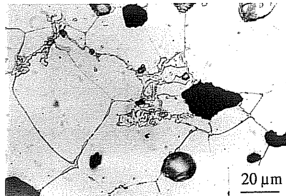
fig. II.19 - Il ne reste rien de ces précipités après 10 jours à 870 °C
