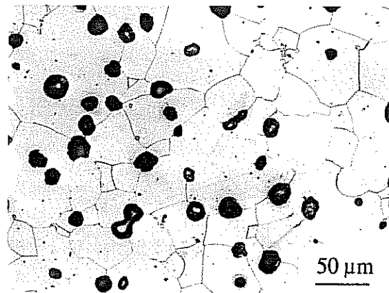
fig II.15 - Croissance de grain dans la GS50 lors d'un traitement de décarburation à 900°C
