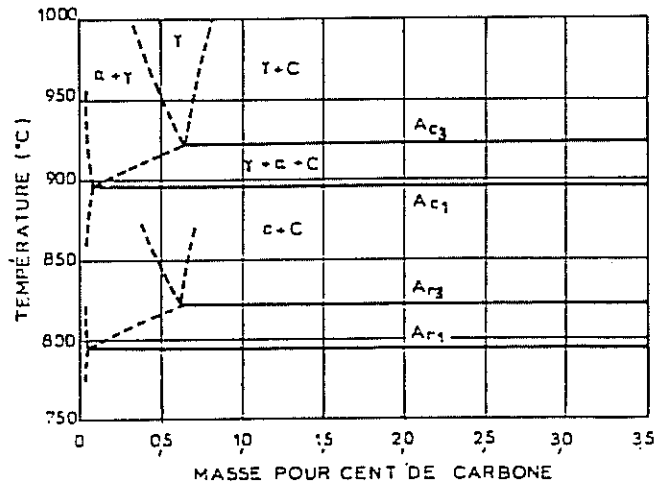
fig. 1.7 - Coupe pseudo-binaire du diagramme Fe-C-Si à 4,2 % de Si [TI-DE]
