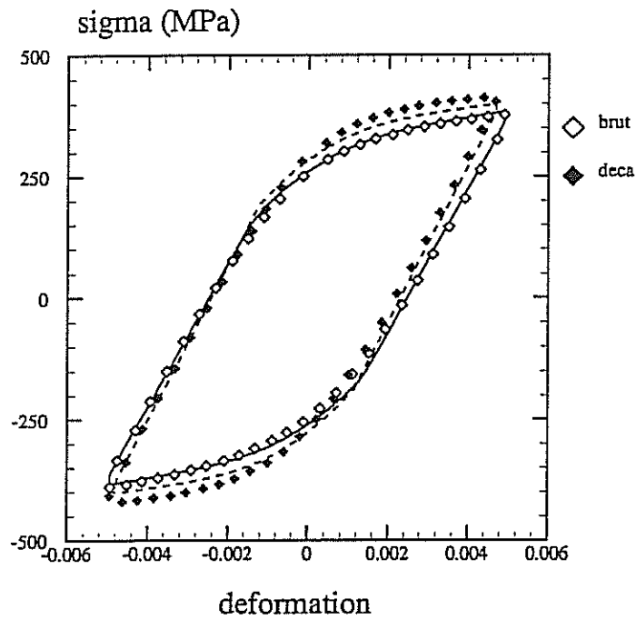
fig. III.34 - Identité de l'écroutissage à 400°C d'une fonte GS50 brute de coulée et d'une fonte GS50 décarburée (vitesse de sollicitation : 10^{-3} \text{ s}^{-1} )
