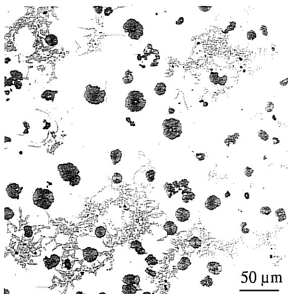
fig. II. 32 - SiMo exposée 1 h à 855 °C
