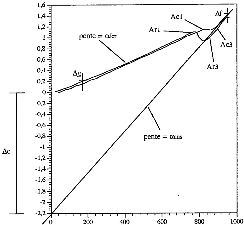
fig III.4 - Courbe de dilatométrie simple
