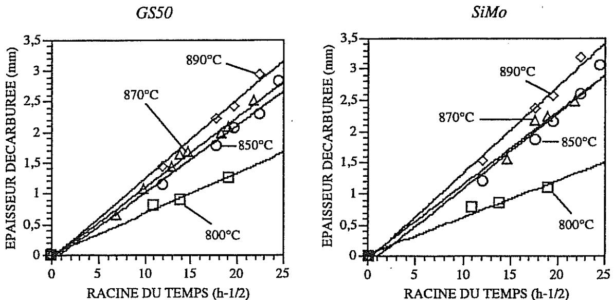
fig. II.20 - Evolution avec le temps de la profondeur de matériau décarburee pour différentes températures
