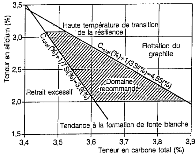
fig. 1.5 - Limitation du domaine de variation des teneurs en Carbone et Silicium [TI-PFGN]
