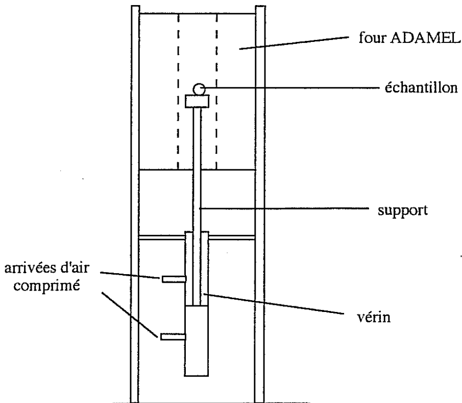
fig. III.12 - Schéma du dispositif de cyclage thermique
