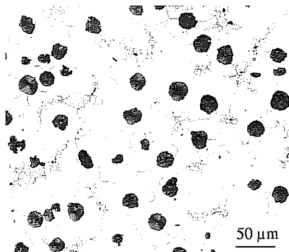
fig. II.2 - Branche de collecteur réalisé en fonte SiMo
