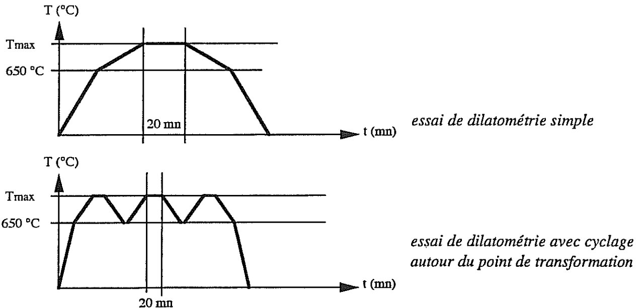
fig III.3 - Chargements thermiques
