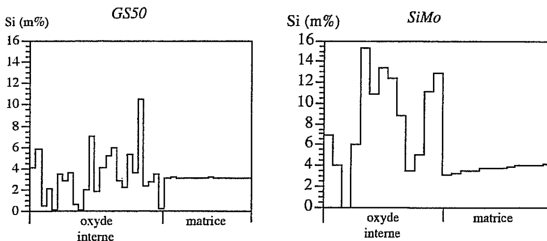
fig. II.9 - Profils de concentration en Silicium au voisinage de la couche d'oxydes
