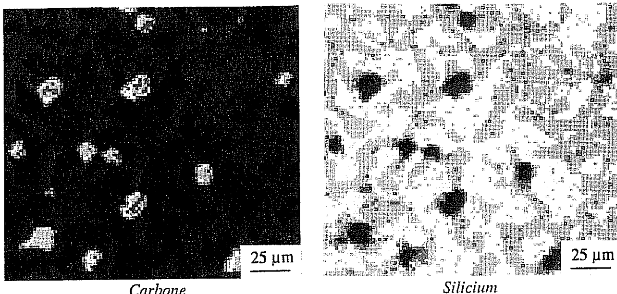
fig II.28 - Concentrations en Carbone et Silicium pour la SiMo après 2 jours à 870°C (imagerie X). Une zone claire indique un enrichissement en l'élément considéré.
