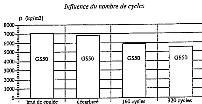
fig. II.38 - Masse volumique de divers échantillons déterminée par pycnométrie
