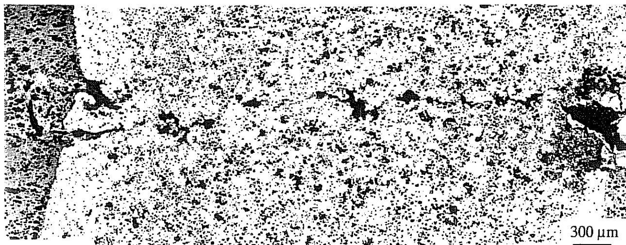
fig. I.19 - Fissure apparue sur un collecteur en service
