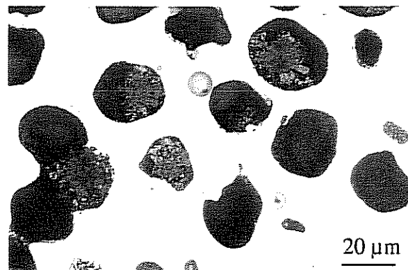
fig. II.36 - Apparition de lacunes autour des nodules sur un échantillon de GS50 cyclé entre T_{\text{amb}} et 900 ^{\circ}\text{C}
