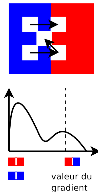
FIG. 5.5: Histogramme des distances et calcul du gradient. Le premier mode correspond aux couples intra-objets, le second aux couples inter-objets. L'abscisse de ce mode nous donne une bonne valeur de gradient.
