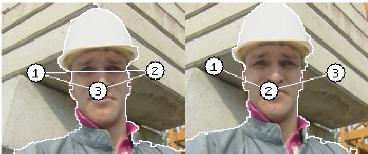
FIG. 3.15: Suivi d'un objet : même avec un mouvement faible, la restriction imposée par le champ de la caméra peut fortement influencer sur la topologie du graphe. Selon la position du casque, les zones de fond sur les deux côtés sont connectées ou non. Encore une fois, 33% des arêtes sont problématiques.
